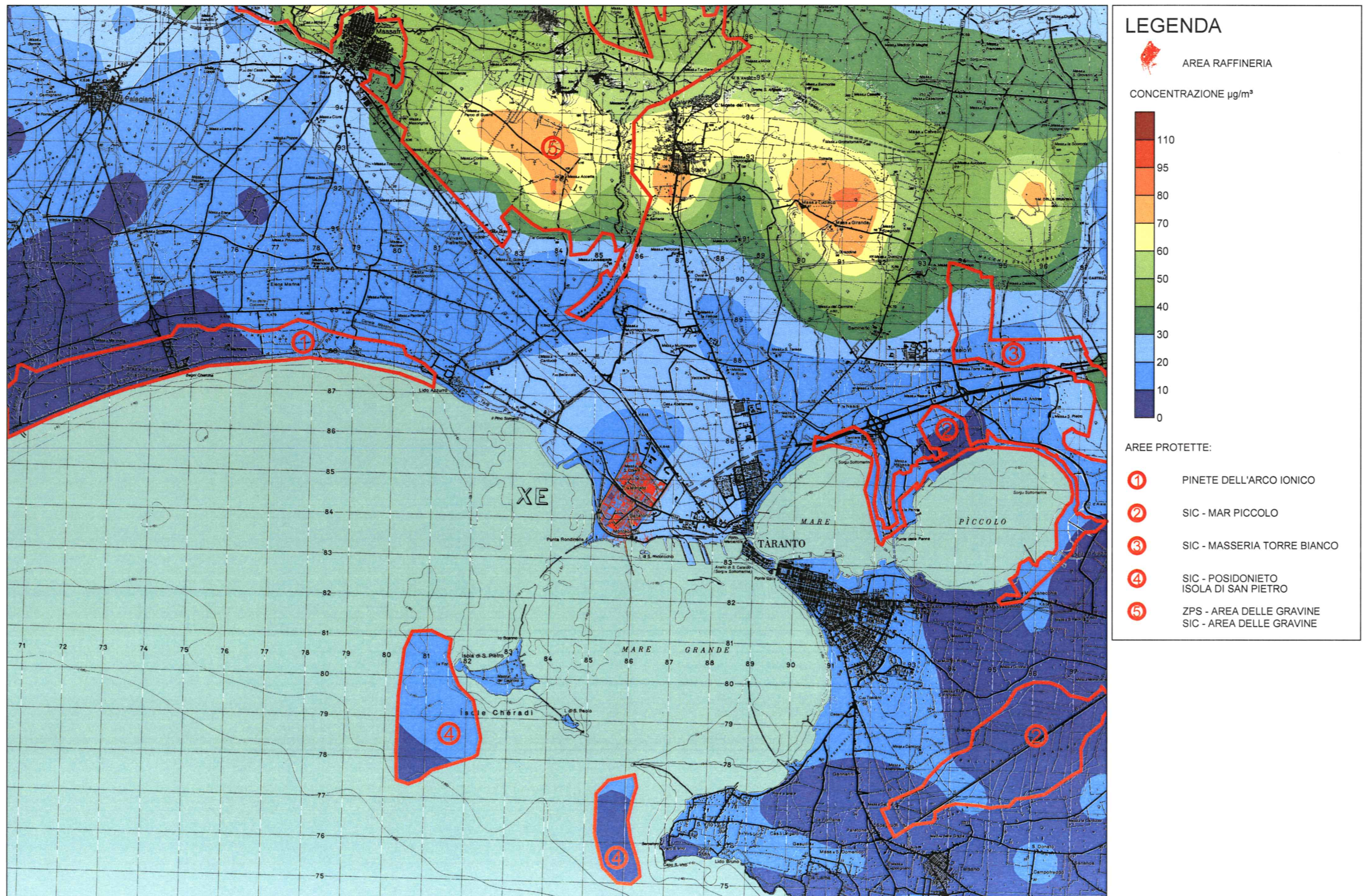
Figura 5.3.1.2e 99,8° Percentile delle Concentrazioni Medie Orarie di NOx nello Scenario Attuale (Scala 1:90.000)
