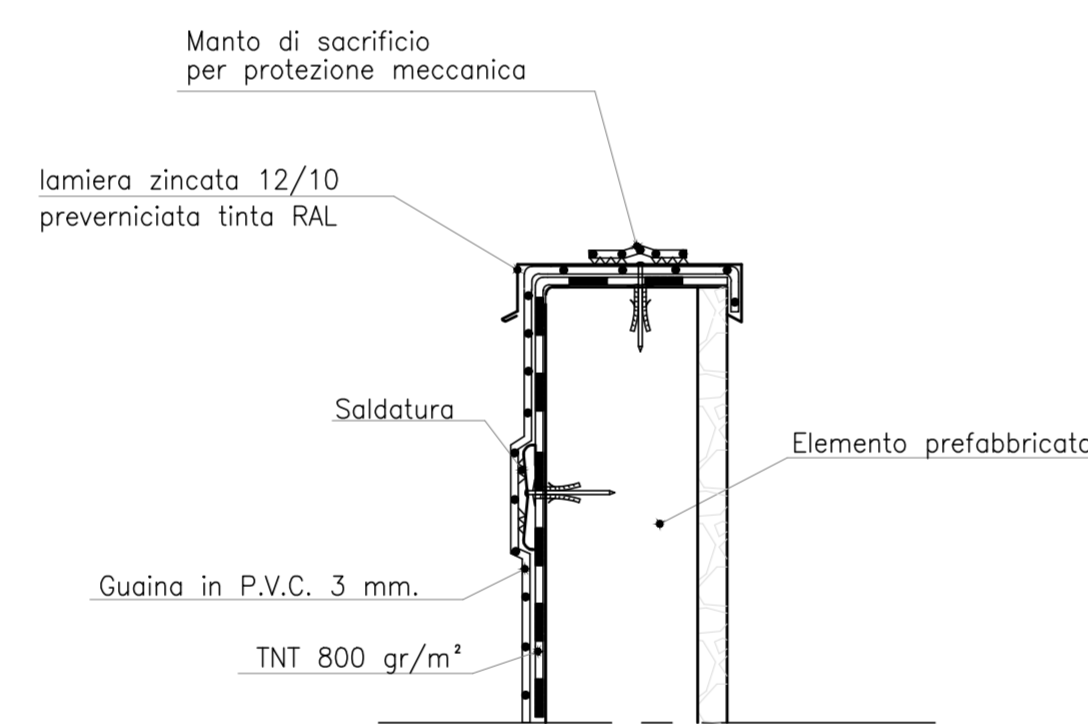
PARTICOLARE "A"
