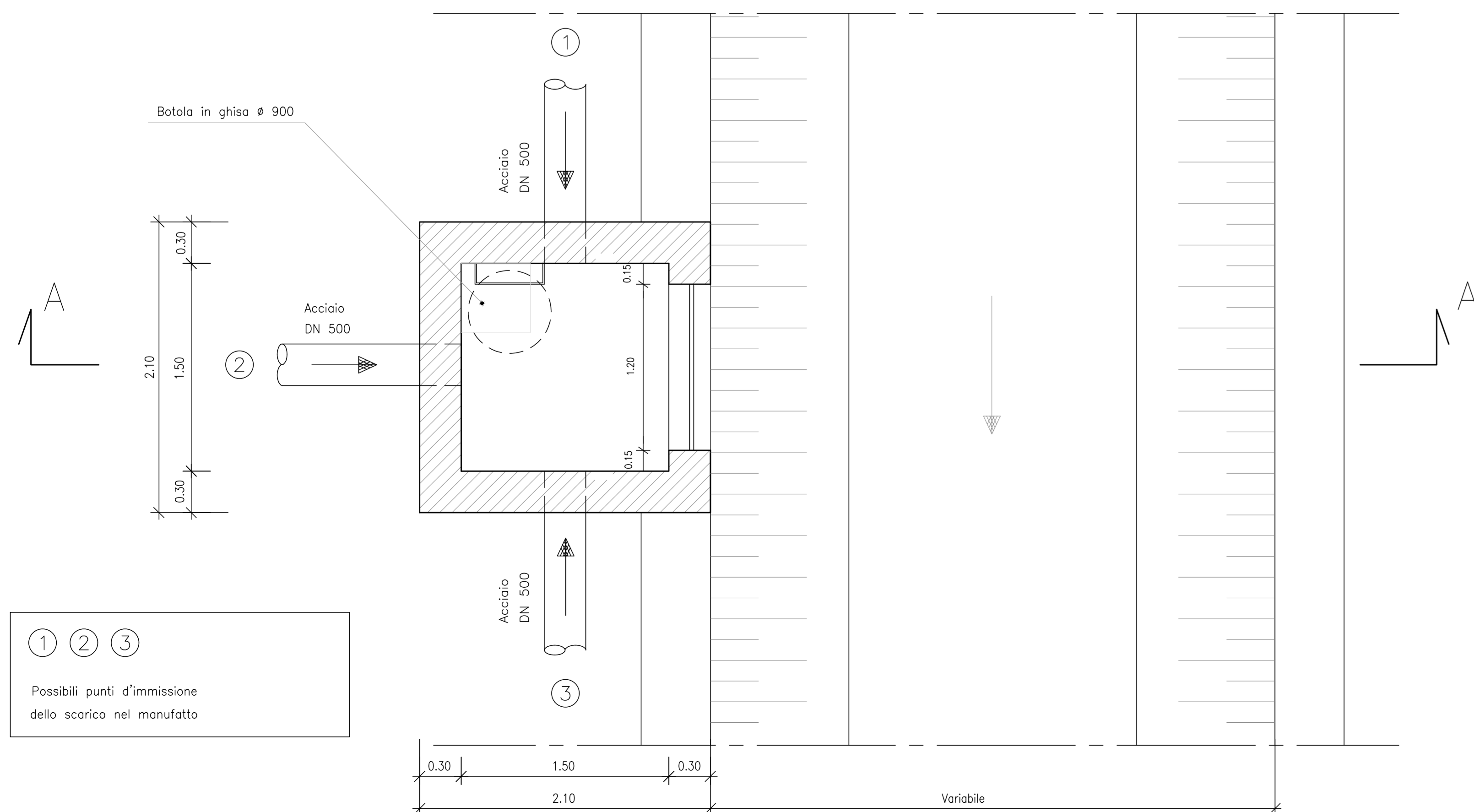
PIANTA Scala 1:25
