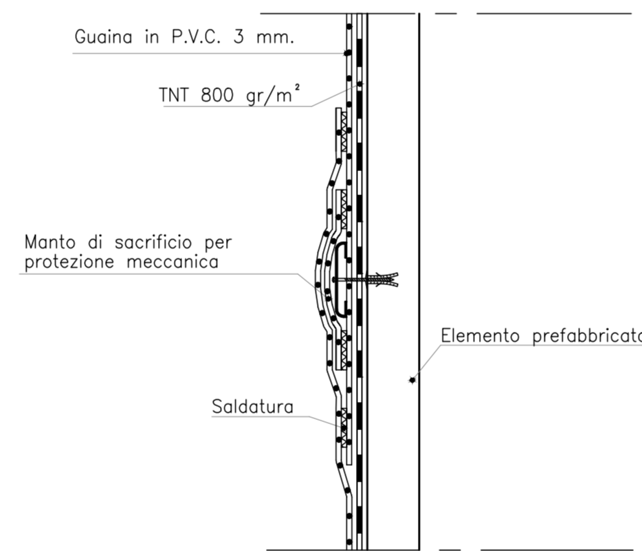
PARTICOLARE "B"
