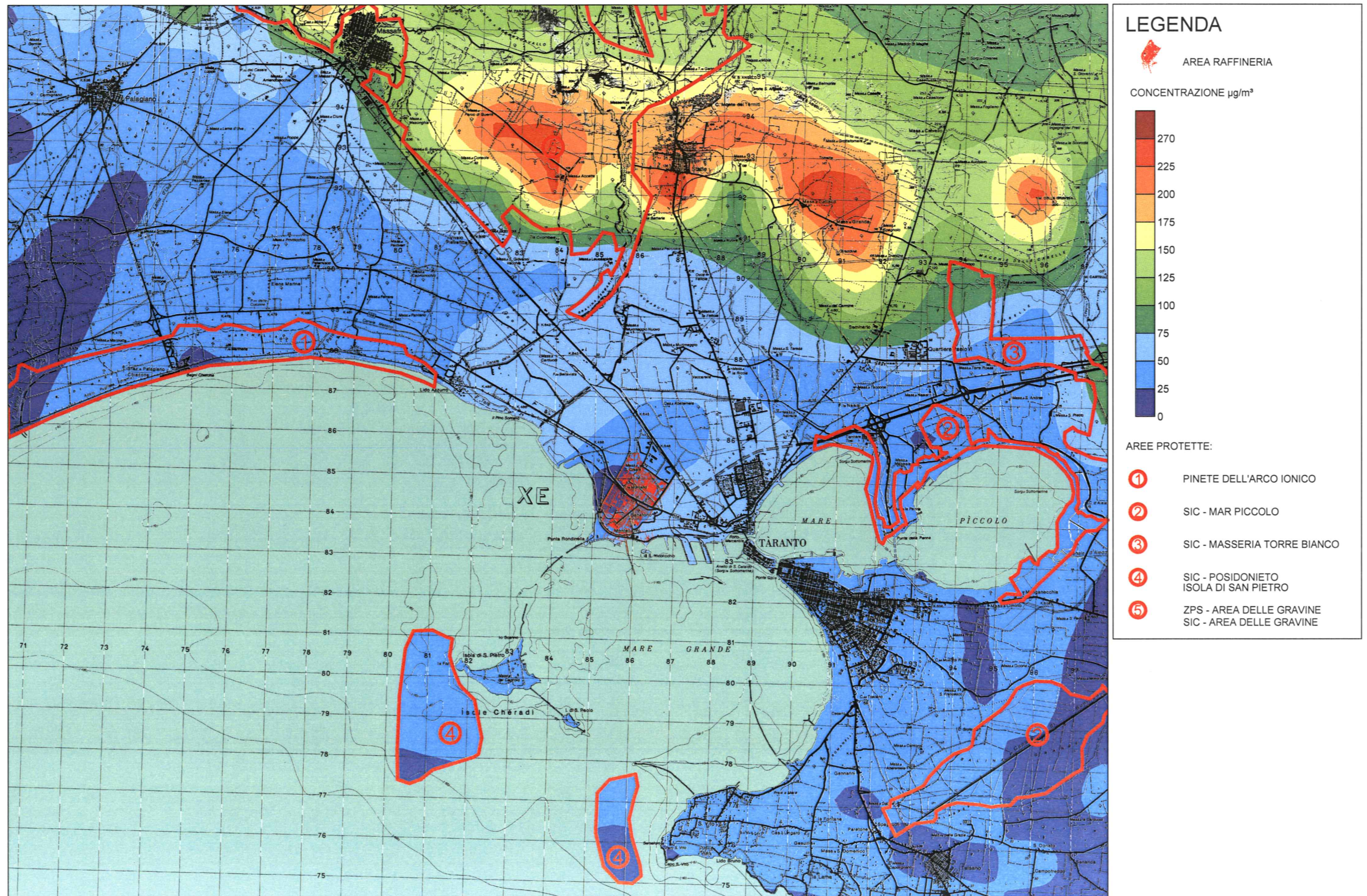
Figura 5.3.1.2f 99,73° Percentile delle Concentrazioni Medie Orarie di SO 2 nello Scenario Attuale (Scala 1:90.000)
