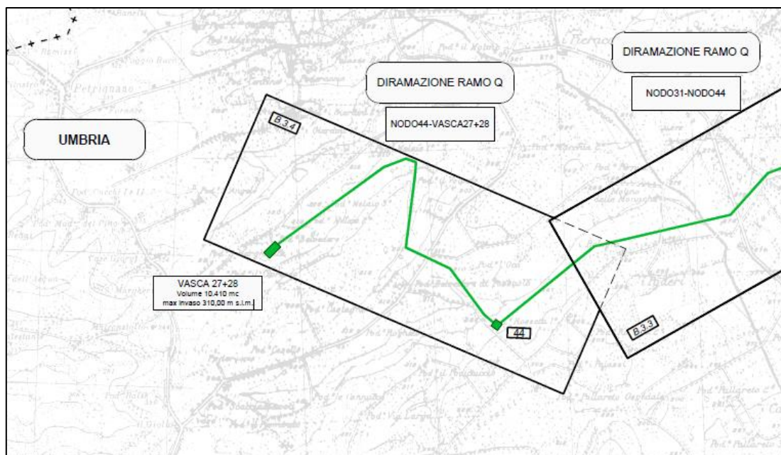
Figura 1 – Stralcio planimetria generale di intervento – fuori scala- (Tav. B.2).
