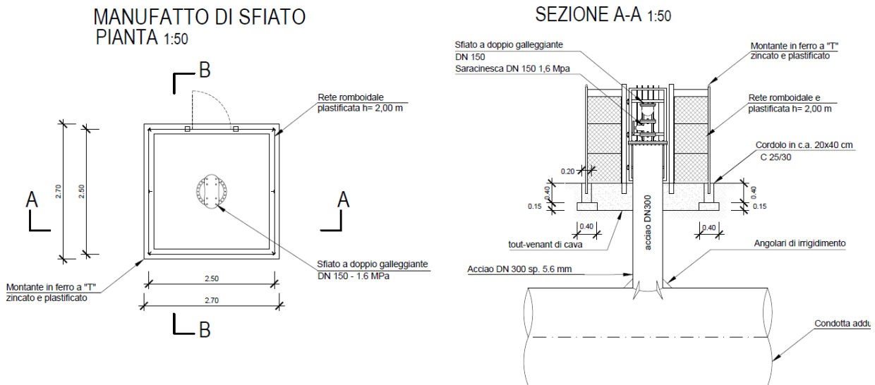
Figura 13 – Manufatto di sfiato – fuori scala (Tav. B8)
