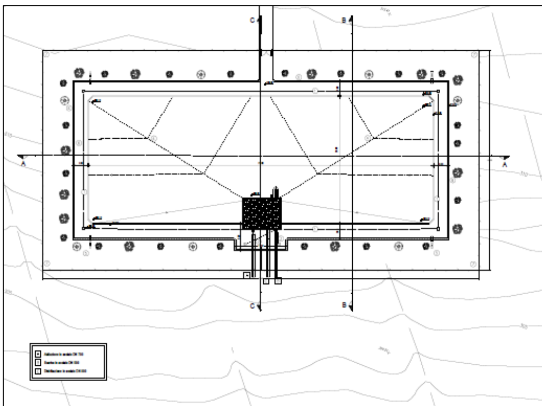
Figura 3 – Stralcio Tav B6.0 – fuori scala.
