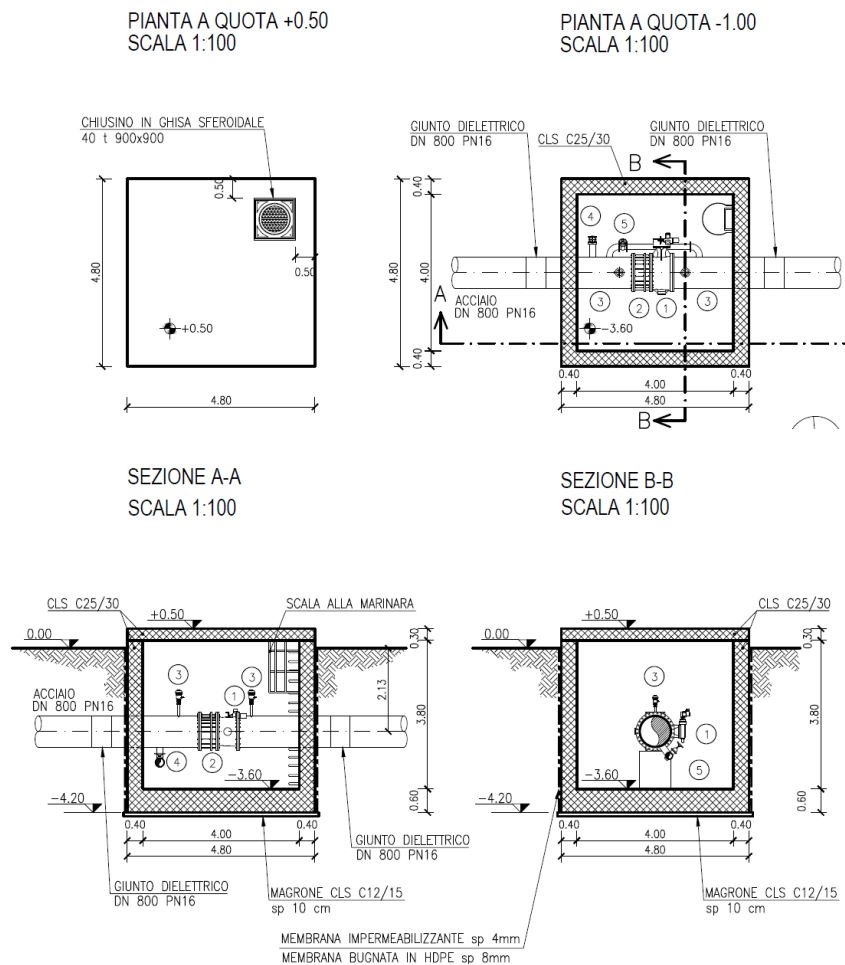
Figura 10 – Schema architettonico tipico dei Nodi di sezionamento – fuori scala (Tav. da B5.5 a B5.9)
