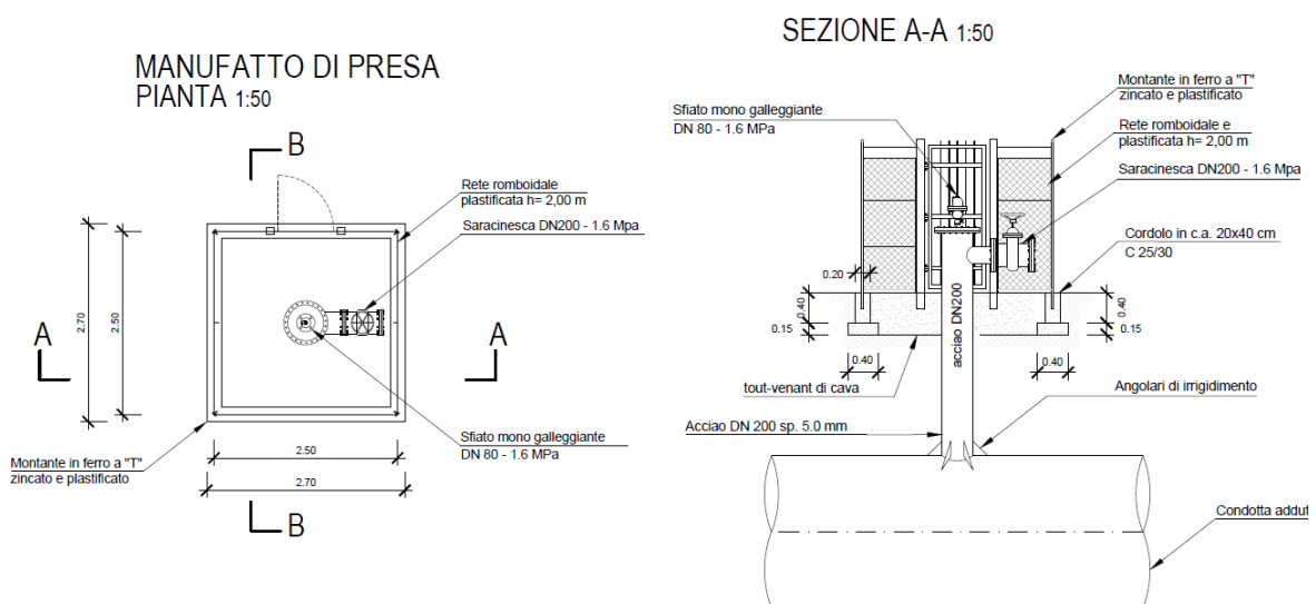
Figura 14 - Manufatto di presa – fuori scala (Tav. B8)
