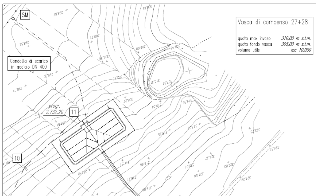
Figura 2 - Stralcio planimetria- fuori scala – (Tav. B3.4)
