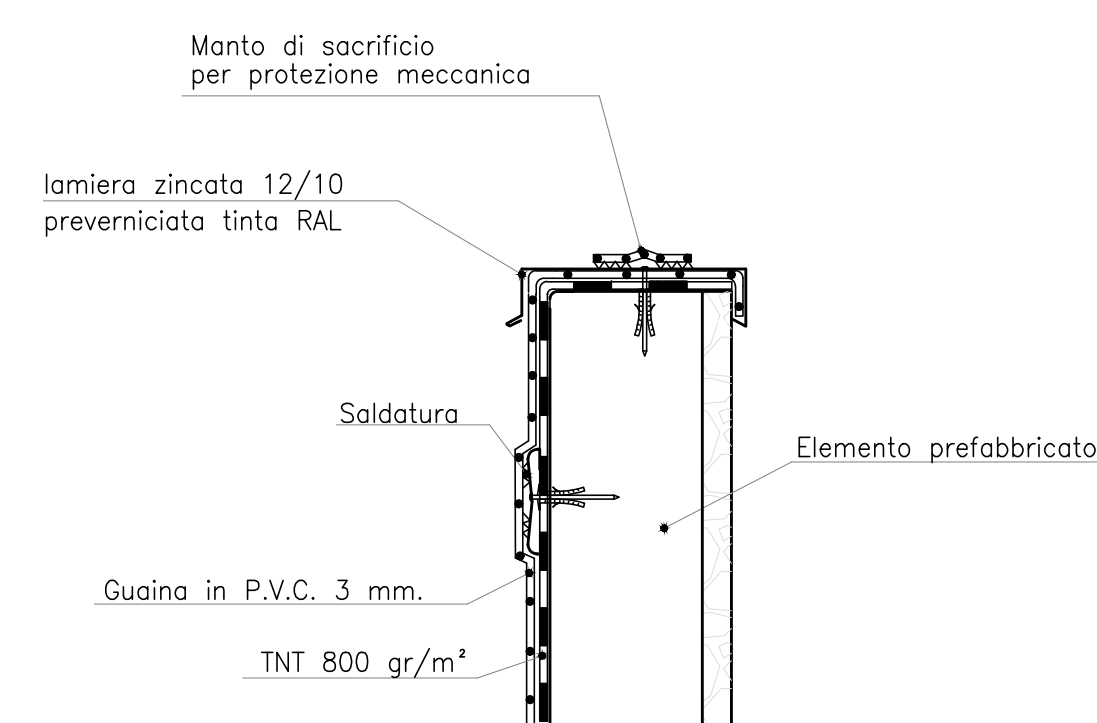
PARTICOLARE "A"
