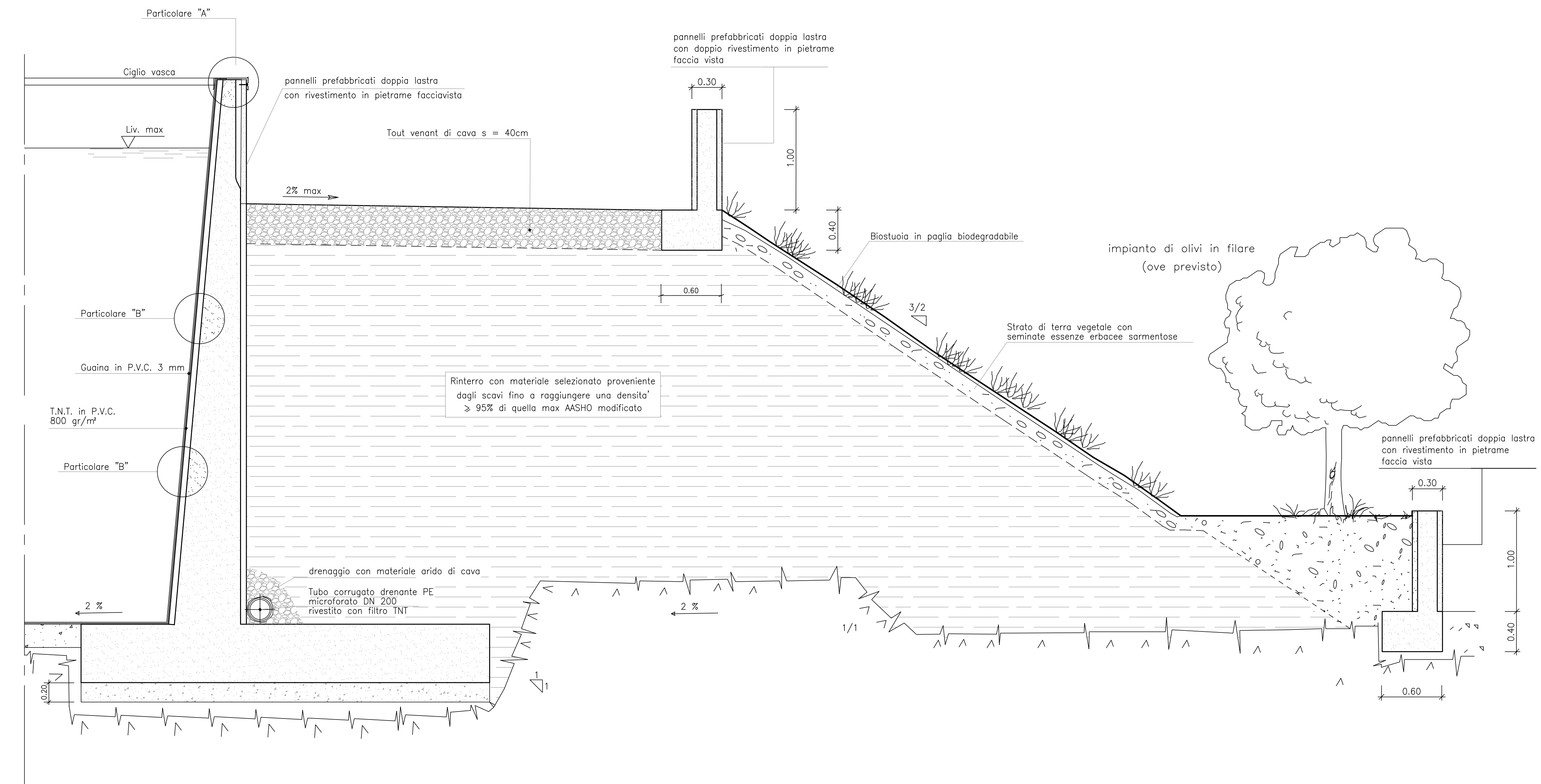
PARTICOLARE SISTEMAZIONE IN RILEVATO Scala 1:25
