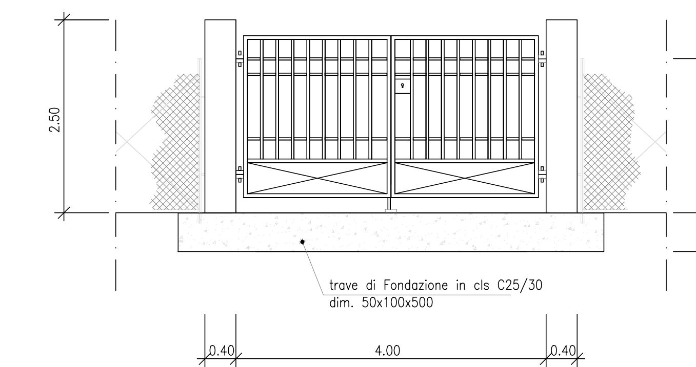
PARTICOLARE CANCELLO D'INGRESSO Scala 1:50
