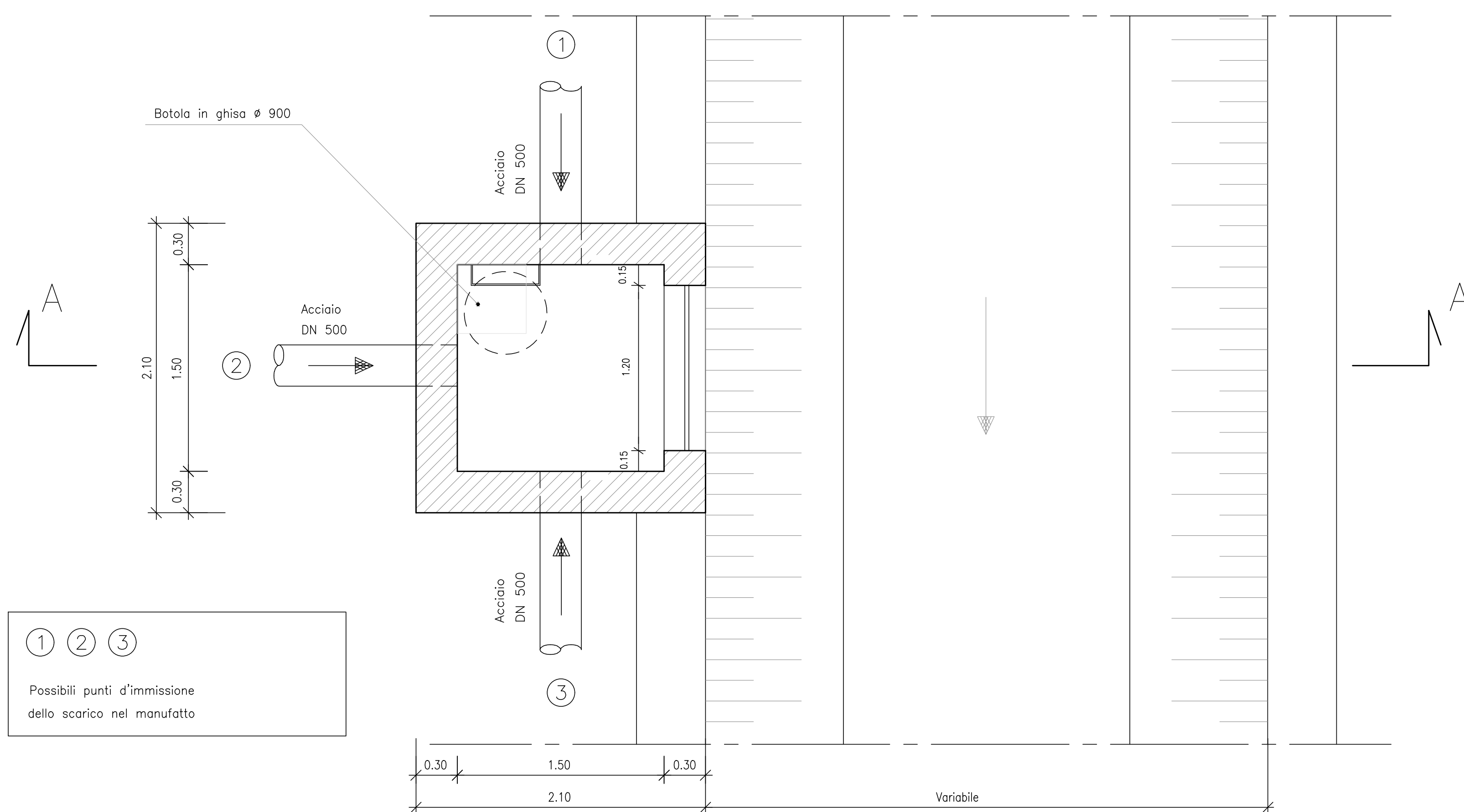
PIANTA Scala 1:25
