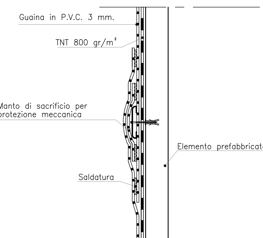
PARTICOLARE "B"
