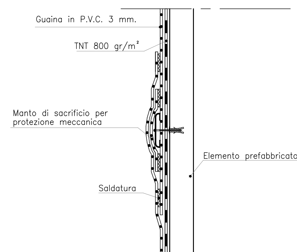
PARTICOLARE "B"
