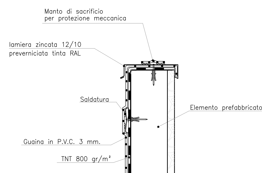
PARTICOLARE "A"
