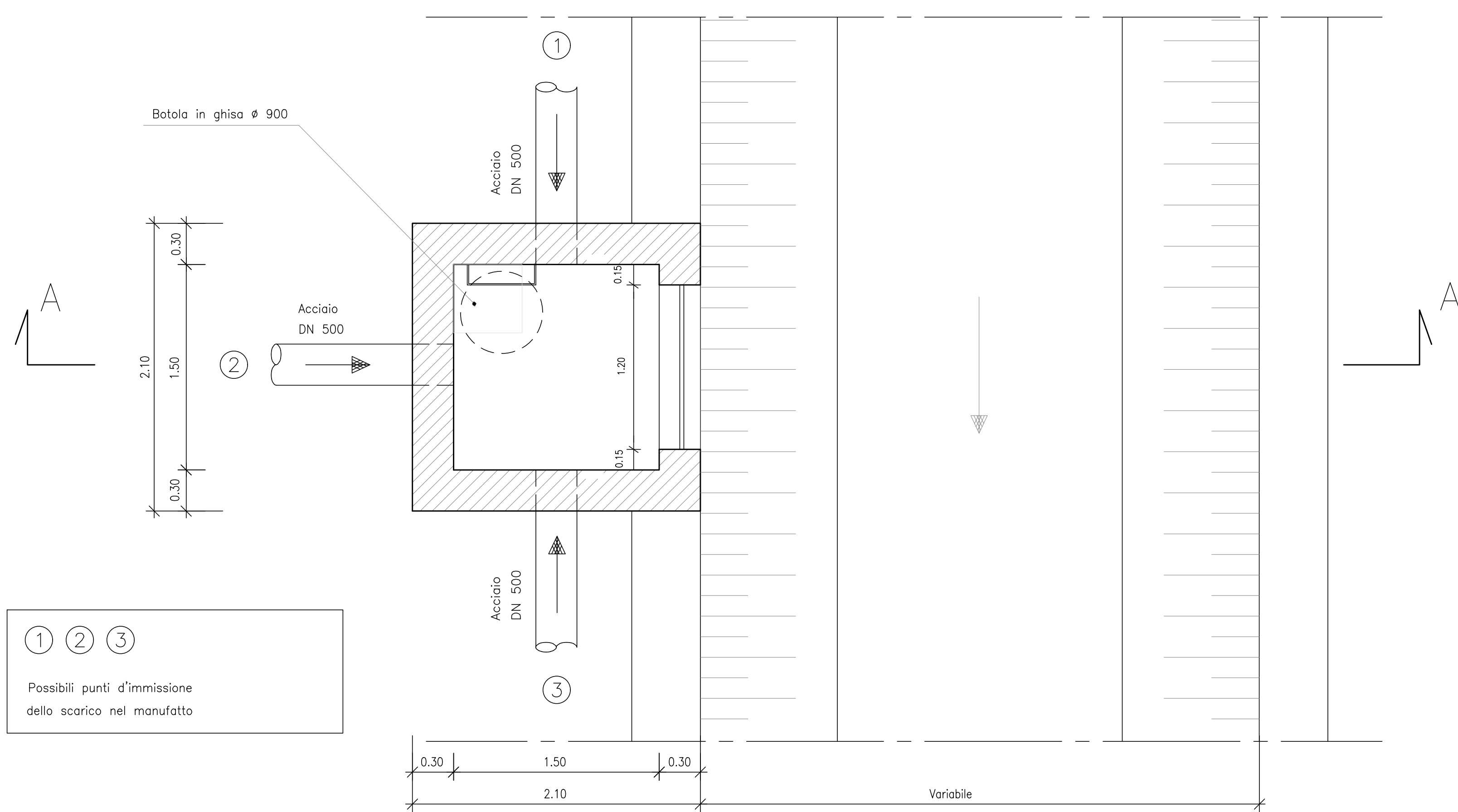
PIANTA Scala 1:25
