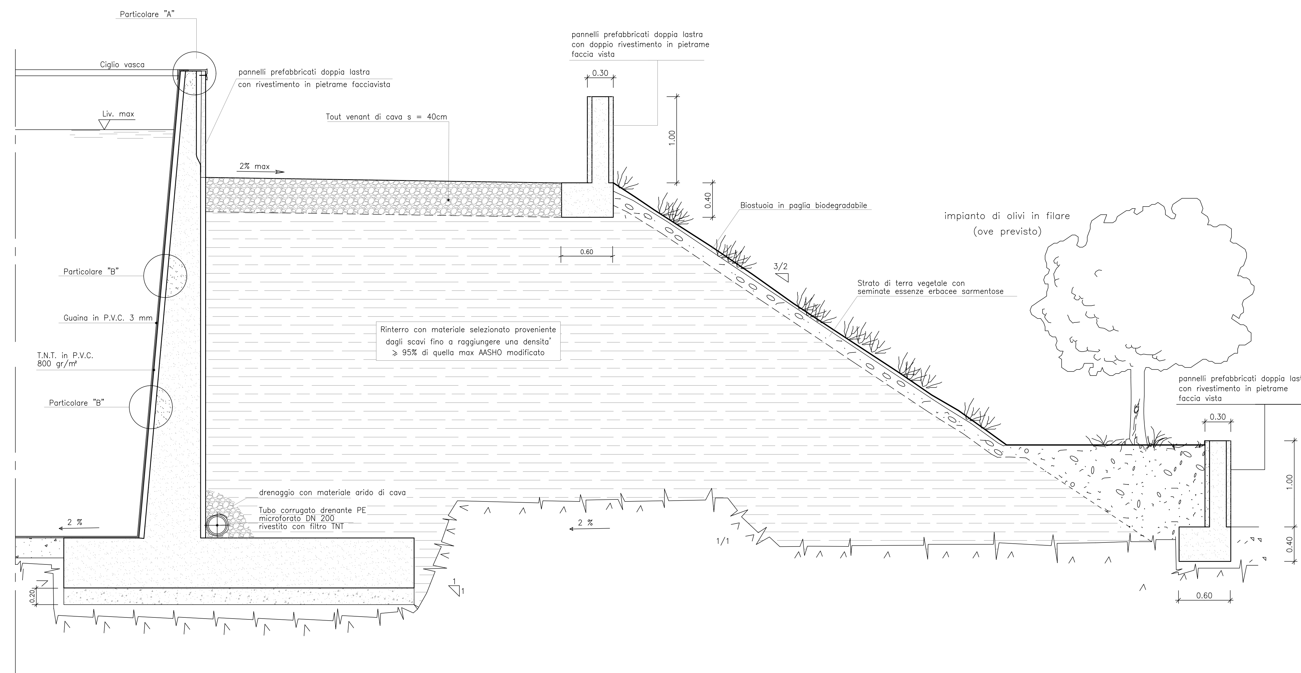
PARTICOLARE SISTEMAZIONE IN RILEVATO Scala 1:25
