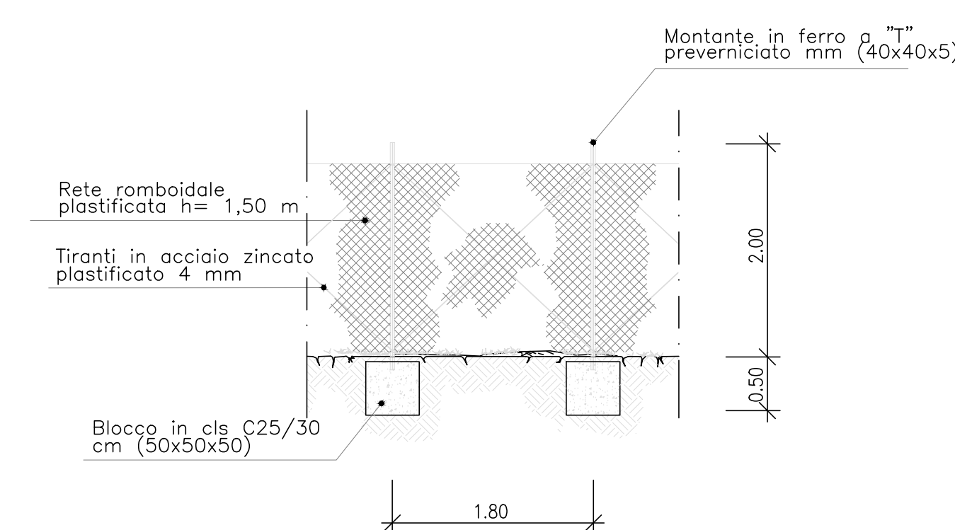
PARTICOLARE RECINZIONE Scala 1:50
