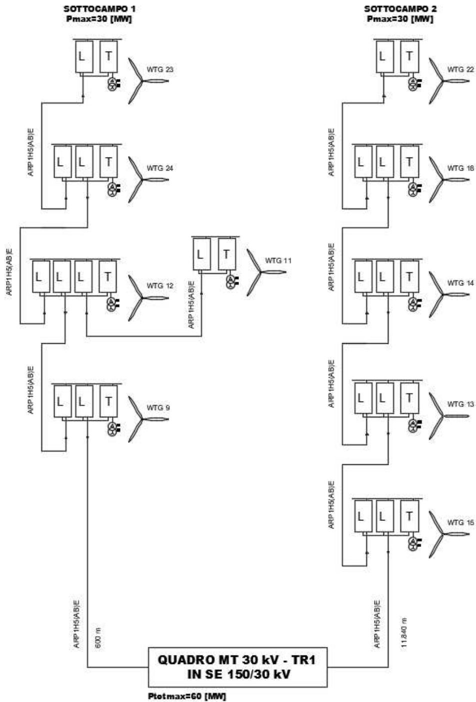
Schema a blocchi del parco eolico TR1
