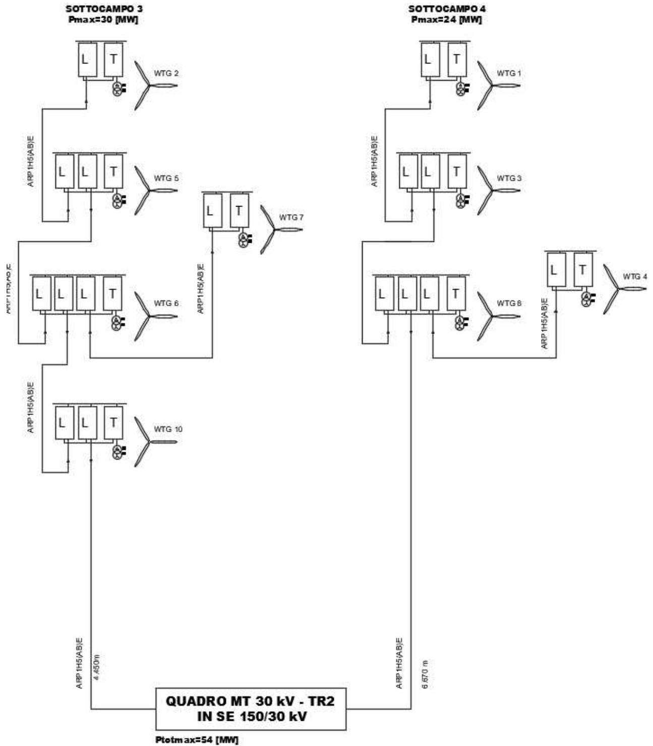
Schema a blocchi del parco eolico TR2
