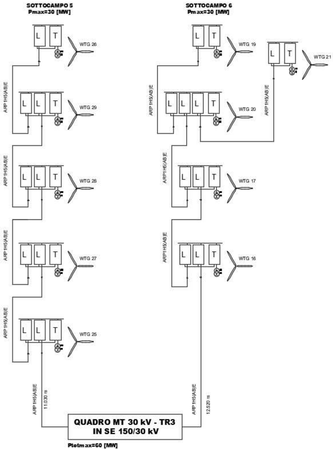
Schema a blocchi del parco eolico TR3
