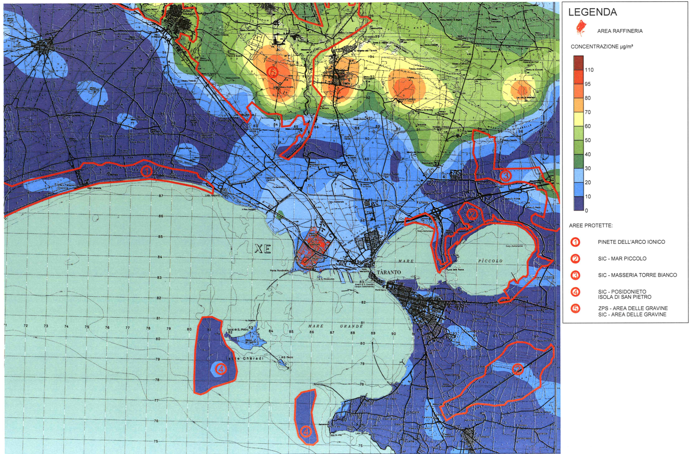
Figura 5.3.1.2m 99,8° Percentile delle Concentrazioni Medie Orarie di NOx nello Scenario Futuro (Scala 1:90.000)
