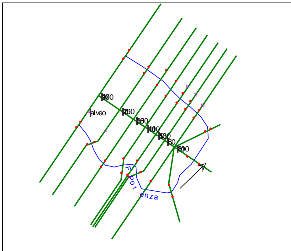
Fig.5.2/B: Modellazione geometrica in Hec Ras (RS170 a monte e RS10 a valle)
