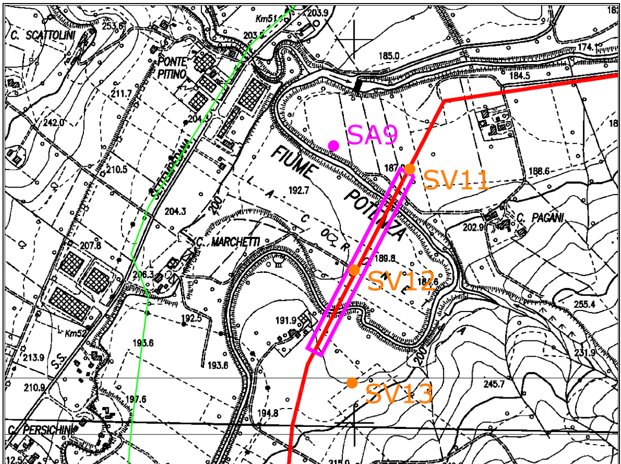
Fig.3.3/A: Planimetria aree 2° e 3° Attraversamento in scala 1:10000, con ubicazione sondaggi 2° attrav. prog. km 30,595 e 3° attrav. prog. km 30,910
