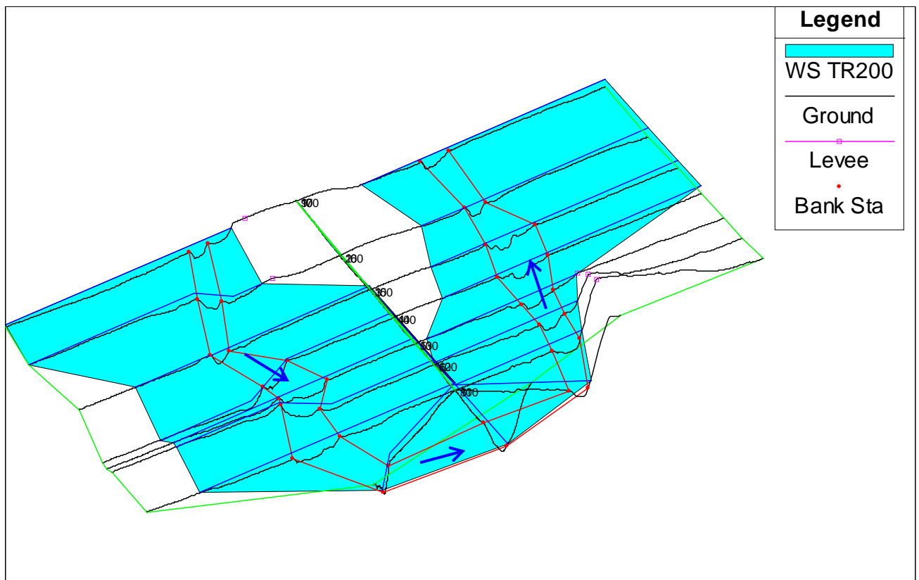
Fig.5.3/A: Schermata di Output del programma – visione prospettica (RS170: monte /RS10: valle)
