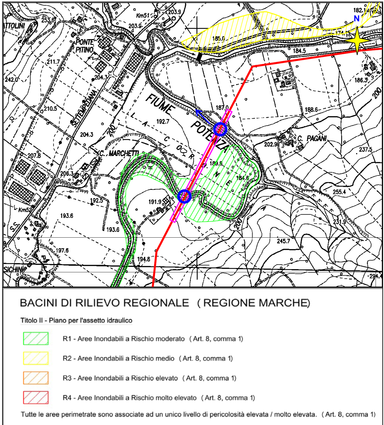
Fig.9.2/A: Interferenze tra metanodotto in progetto con le Aree inondabili del corso d'acqua 2° attrav. prog. km 30,595 e 3° attrav. prog. km 30,910
