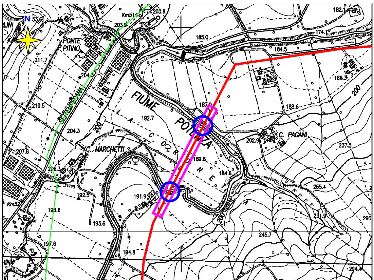
Fig.2.1/B: Stralcio planimetrico in scala 1:10.000 (C.T.R. Regionali) 2° attrav. prog. km 30,595 e 3° attrav. prog. km 30,910
