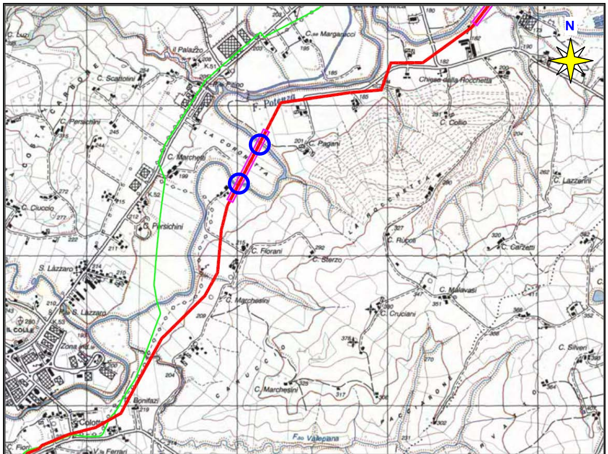
Fig.2.1/A: Corografia generale in scala 1:25.000 (dalle tavolette IGM) 2° attrav. prog. km 30,595 e 3° attrav. prog. km 30,910
