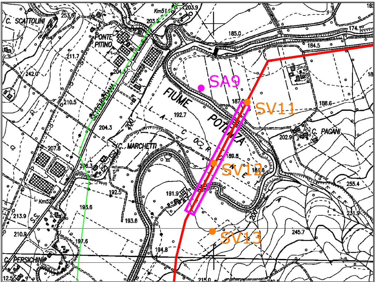
Planimetria aree 2° e 3° Attraversamento in scala 1:10000, con ubicazione sondaggi 2° attrav. prog. km 30,595 e 3° attrav. prog. km 30,910
