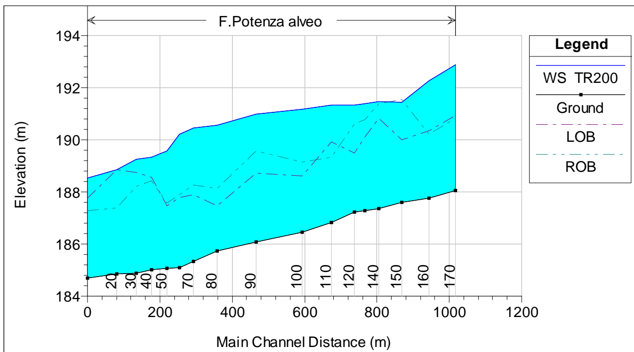
Fig.5.3/B: Schermata di Output del programma – Profilo longitudinale (RS170: monte /RS10: valle)
