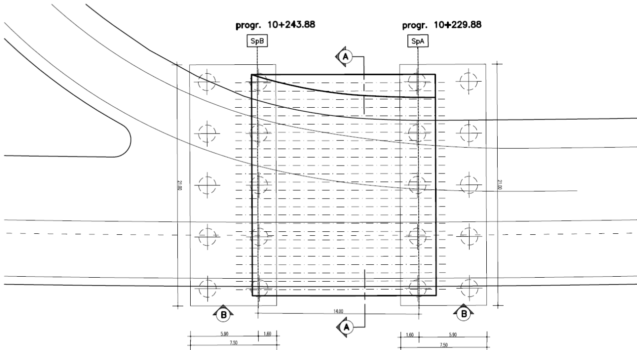
Figura 5.1 – Planimetria viadotto svincolo Annunziata direzione Messina.
