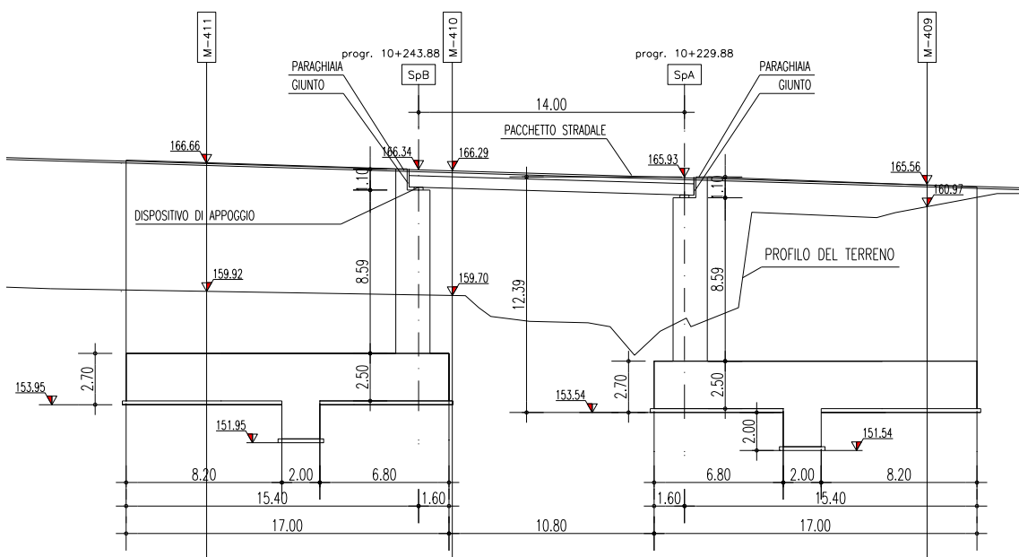
Figura 5.2 – Profilo longitudinale viadotto svincolo Annunziata direzione Messina.
