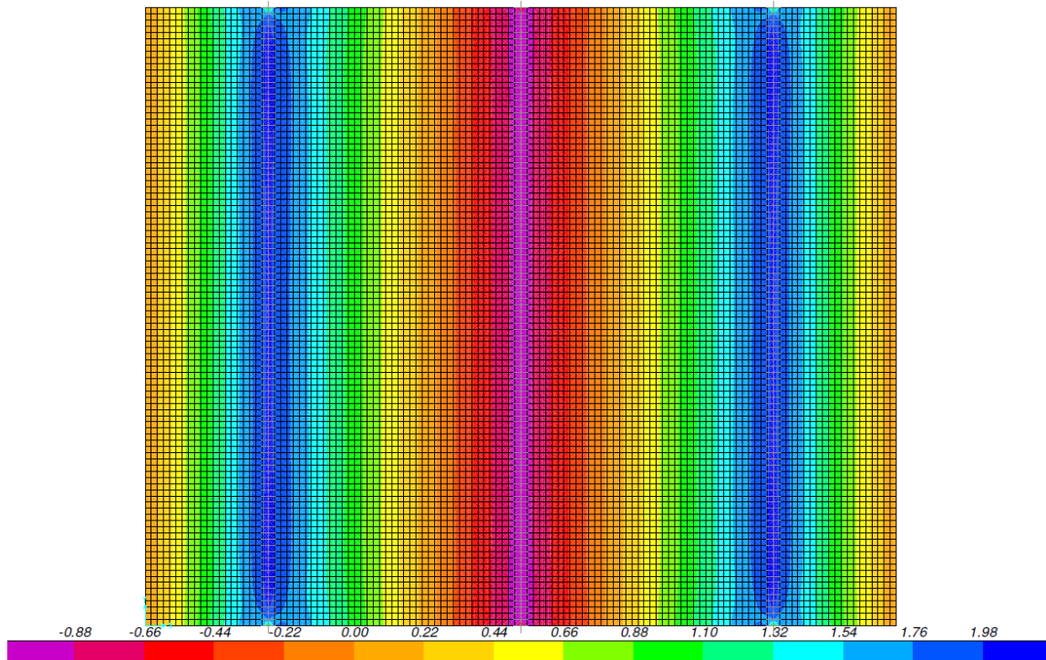
Figura 29 – Momento flettente M_x [kNm/m]
