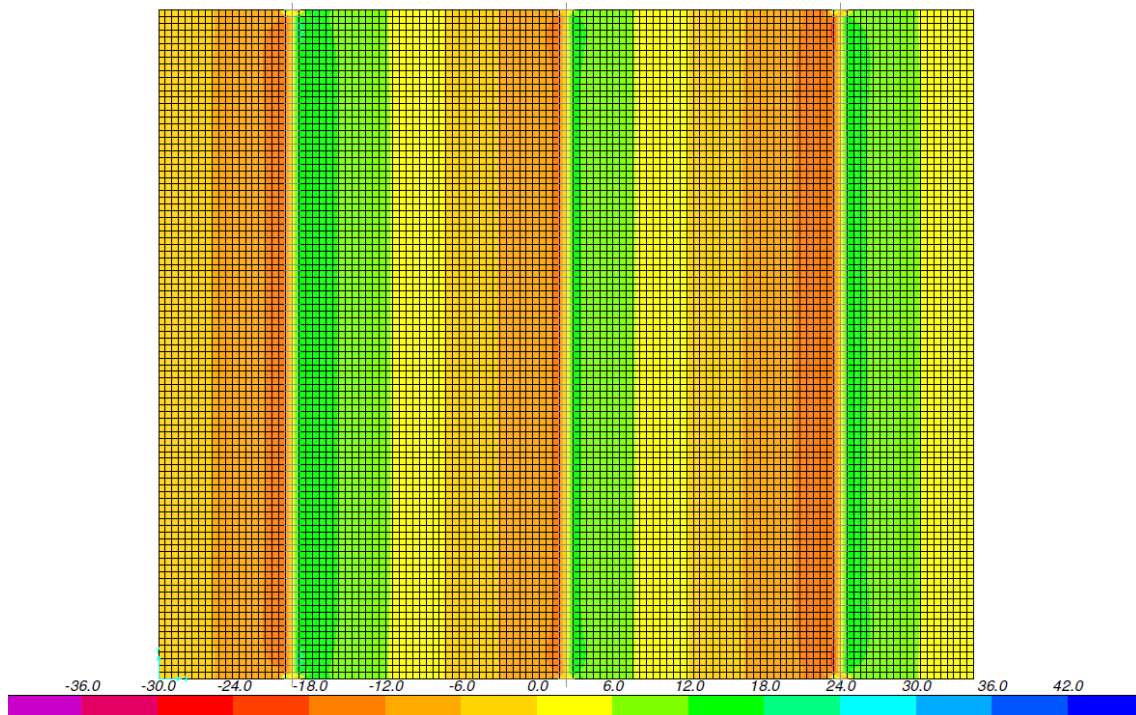
Figura 22 – Taglio V_x [kN/m]
