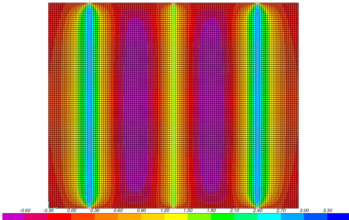
Figura 21 – Momento flettente M_y [kNm/m]
