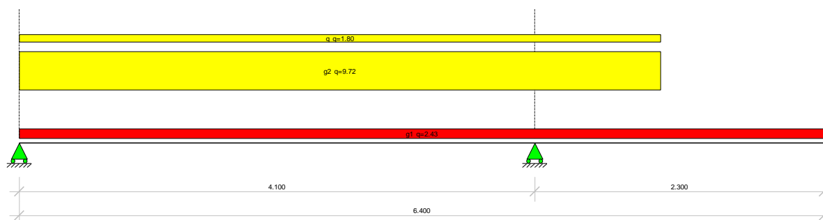
Figura 17 – Schema statico in prima fase
