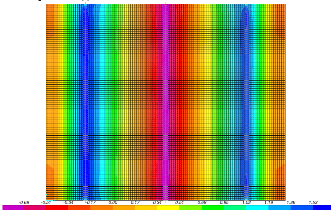
Figura 32 – Momento flettente M_x [kNm/m]
