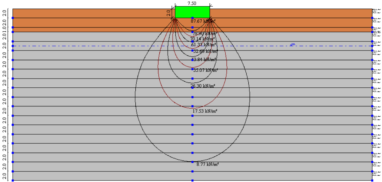
Figura 52 – Bulbi di pressione
