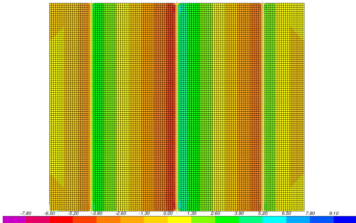
Figura 25 – Taglio V_x [kN/m]
