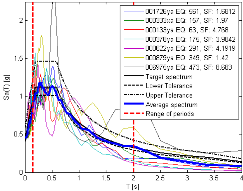
Figura 8 – Spettri orizzontali
