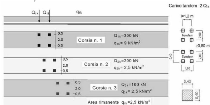
Figura 4 – Schema di carico 1 (dimensioni in [m])
