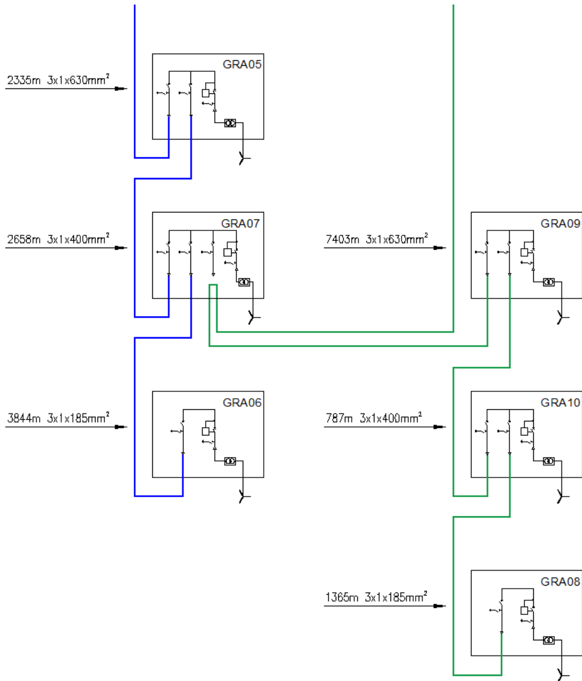
Figura 1: schema a blocchi parco eolico (circuiti 1 e 2)
