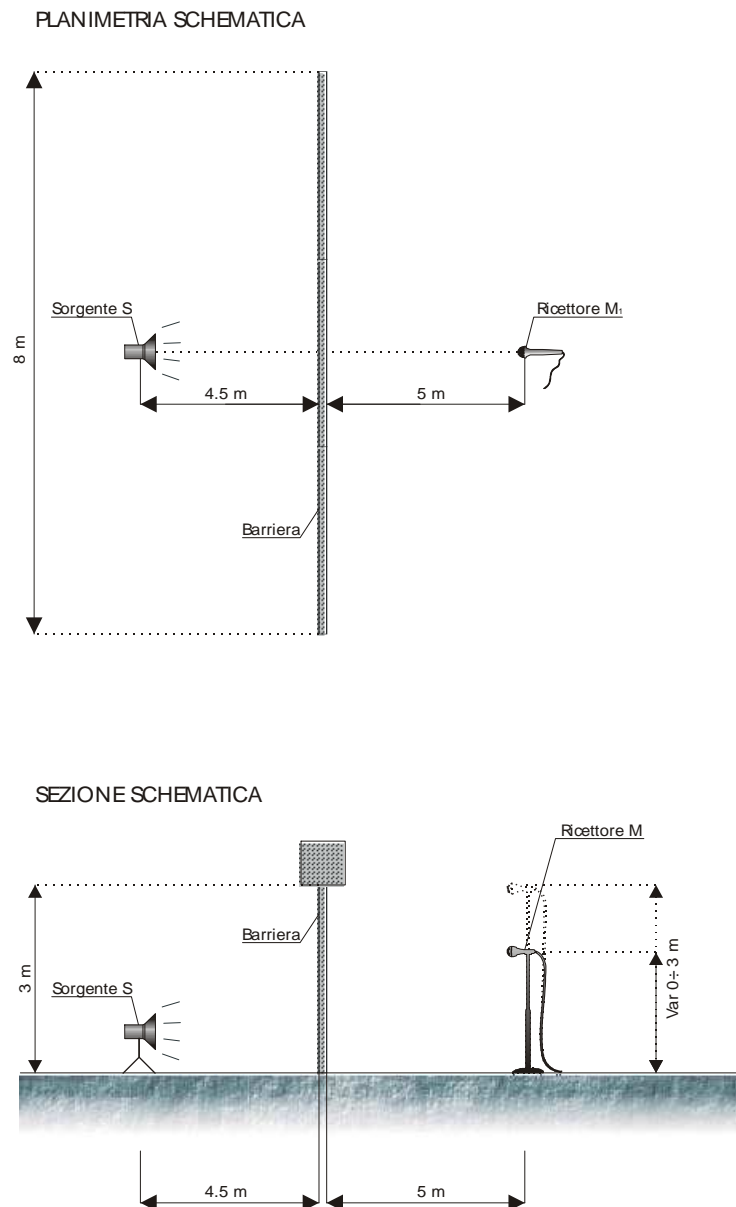
Figura F: schema della prova su elementi antidiffrattivi
