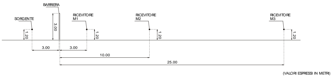
Figura C: schema della prova in campo libero
