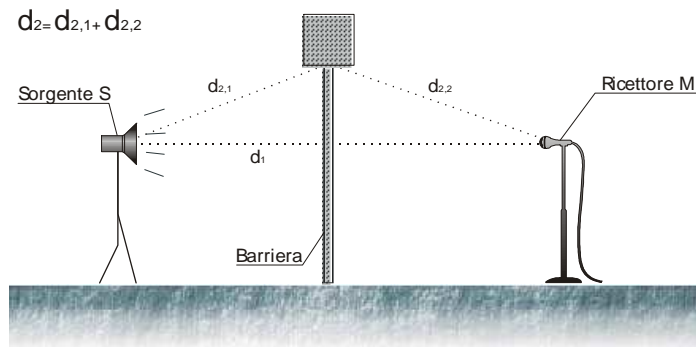
Figura E: schema per il calcolo dei valori di IL
