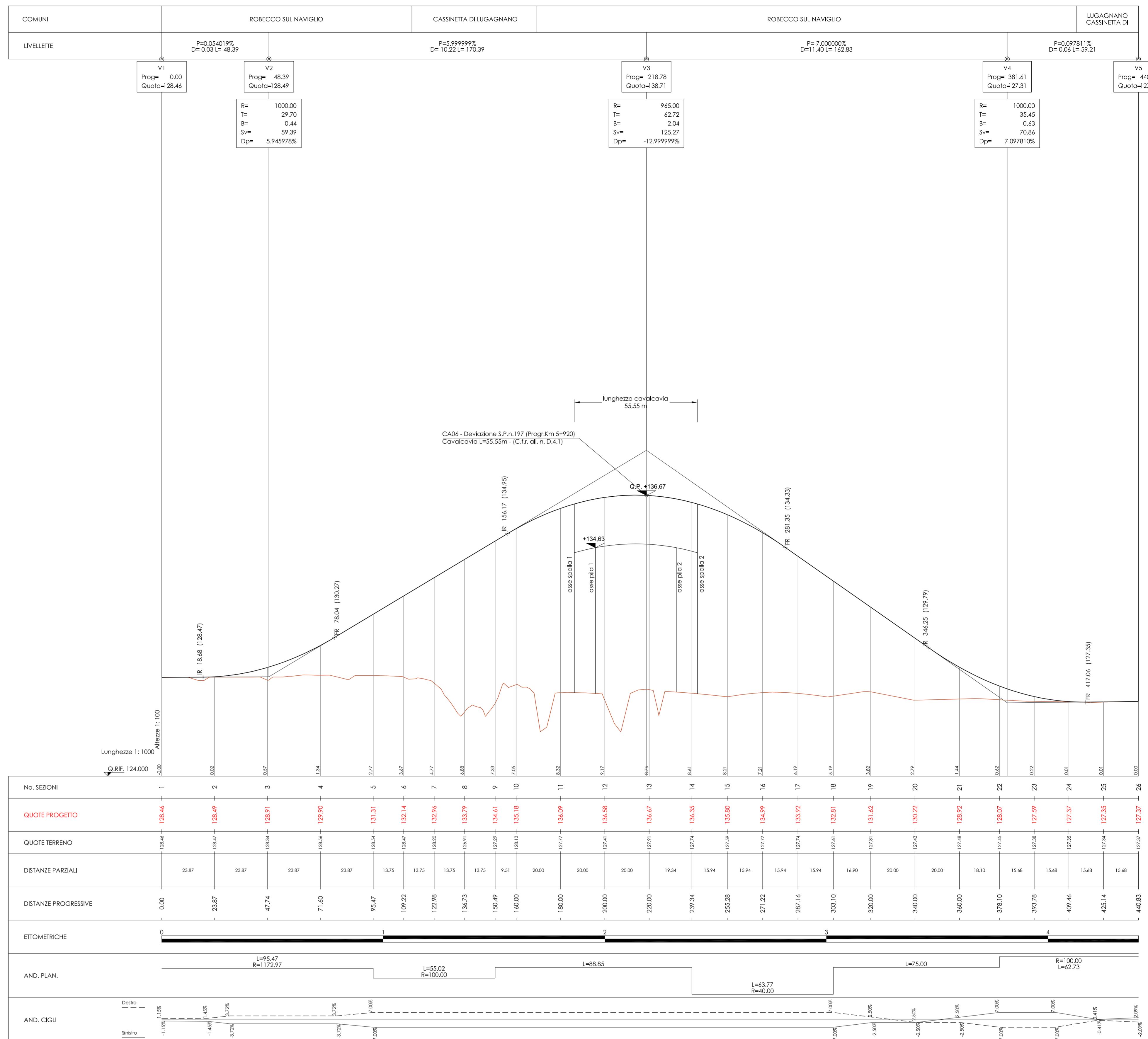
Profilo longitudinale Scala 1:1000/100
