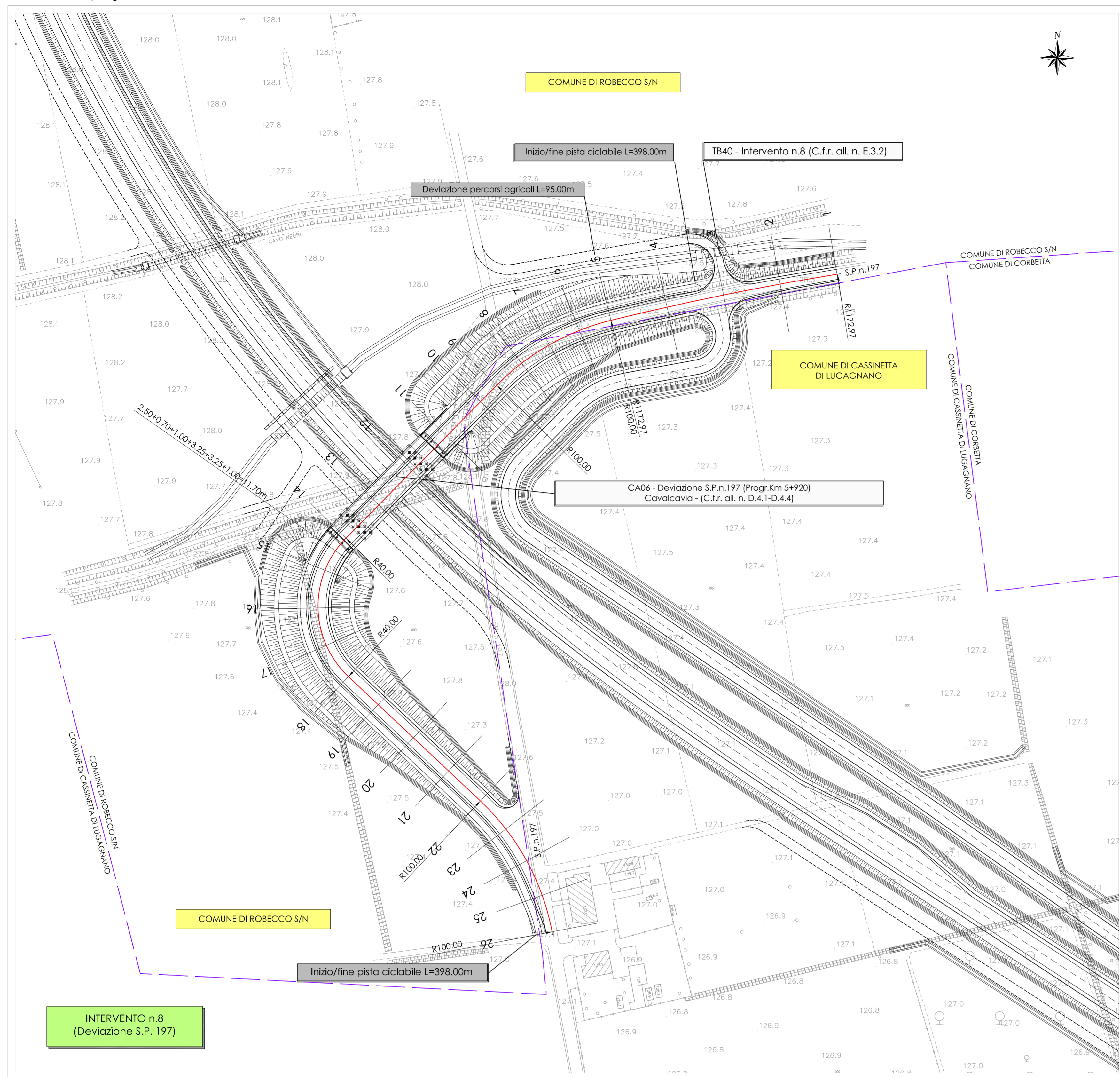
Planimetria di progetto Scala 1:1000
