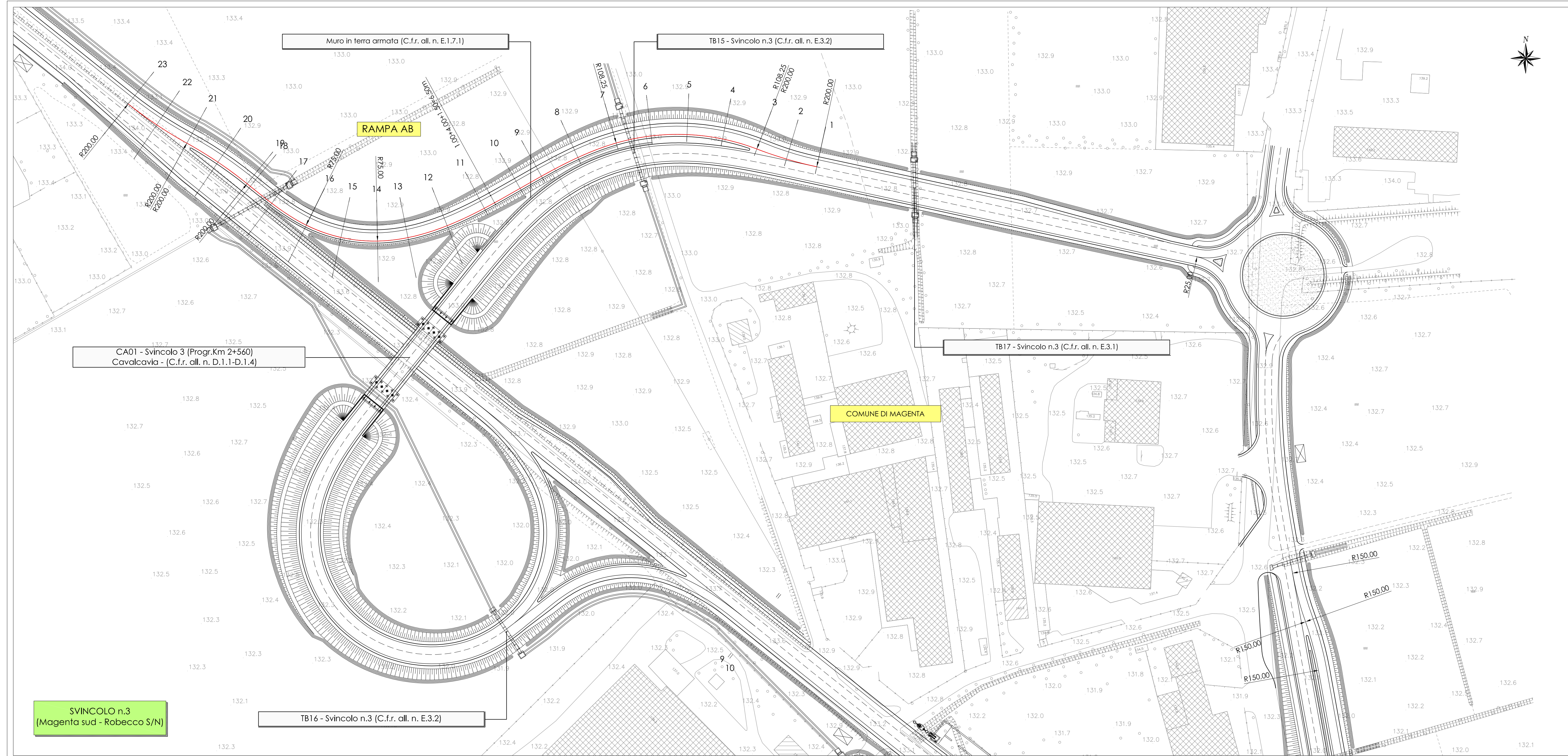
Planimetria di progetto Scala 1:1000
