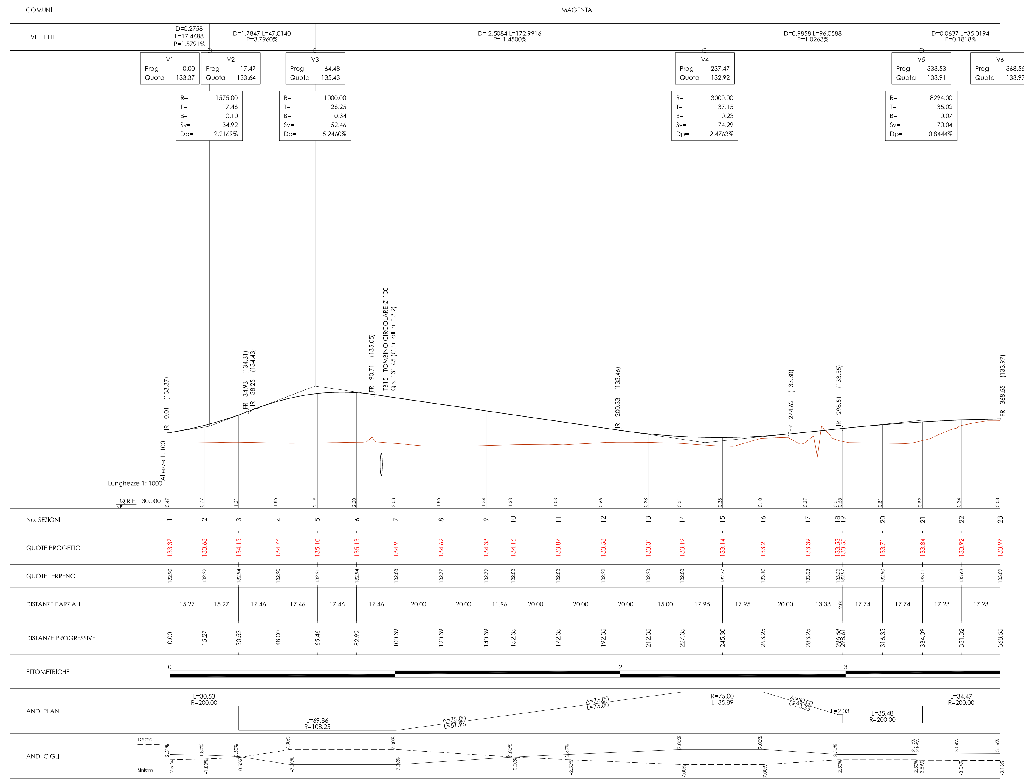
Profilo longitudinale rampa AB Scala 1:1000/100
