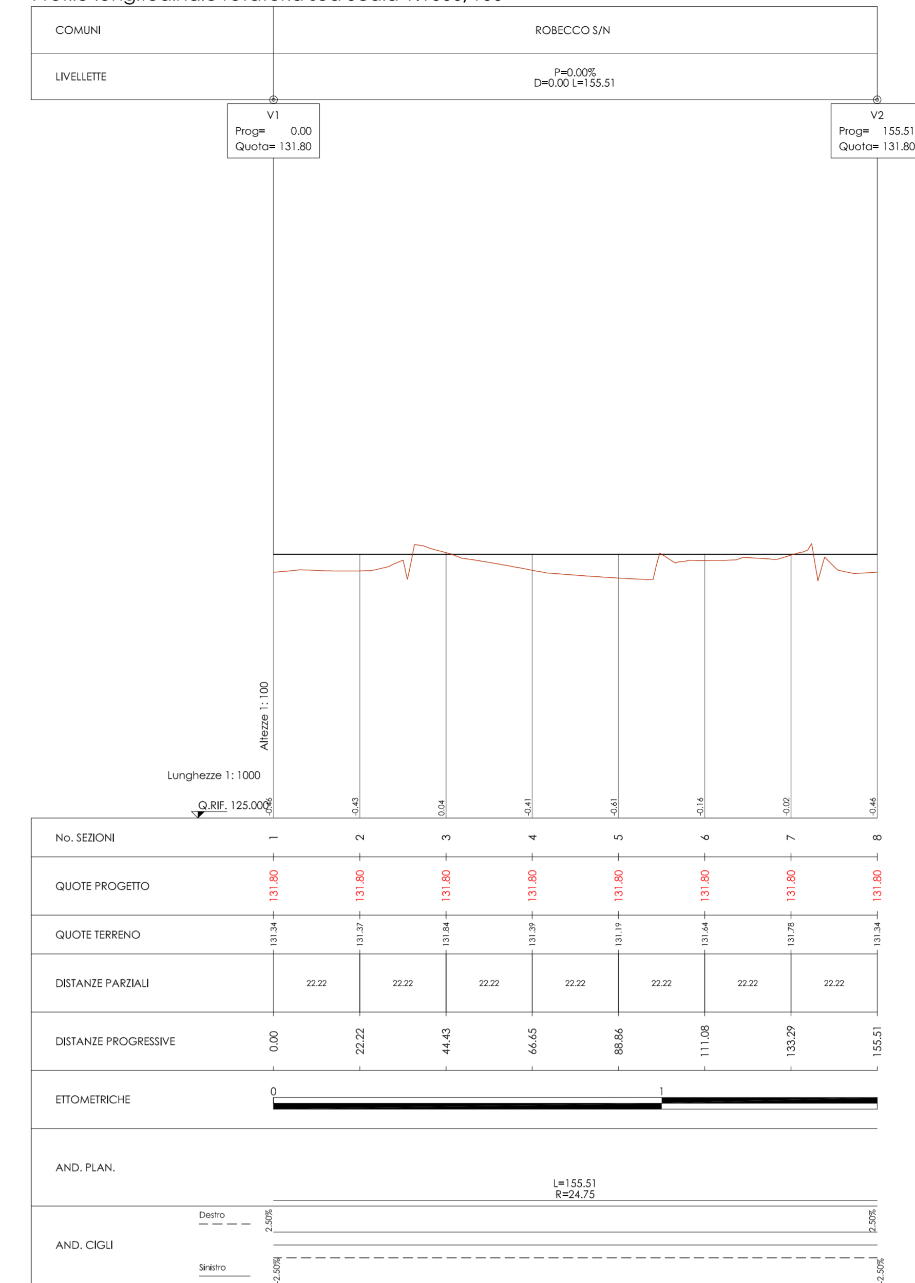
Profilo longitudinale rotondella sud Scala 1:1000/100
