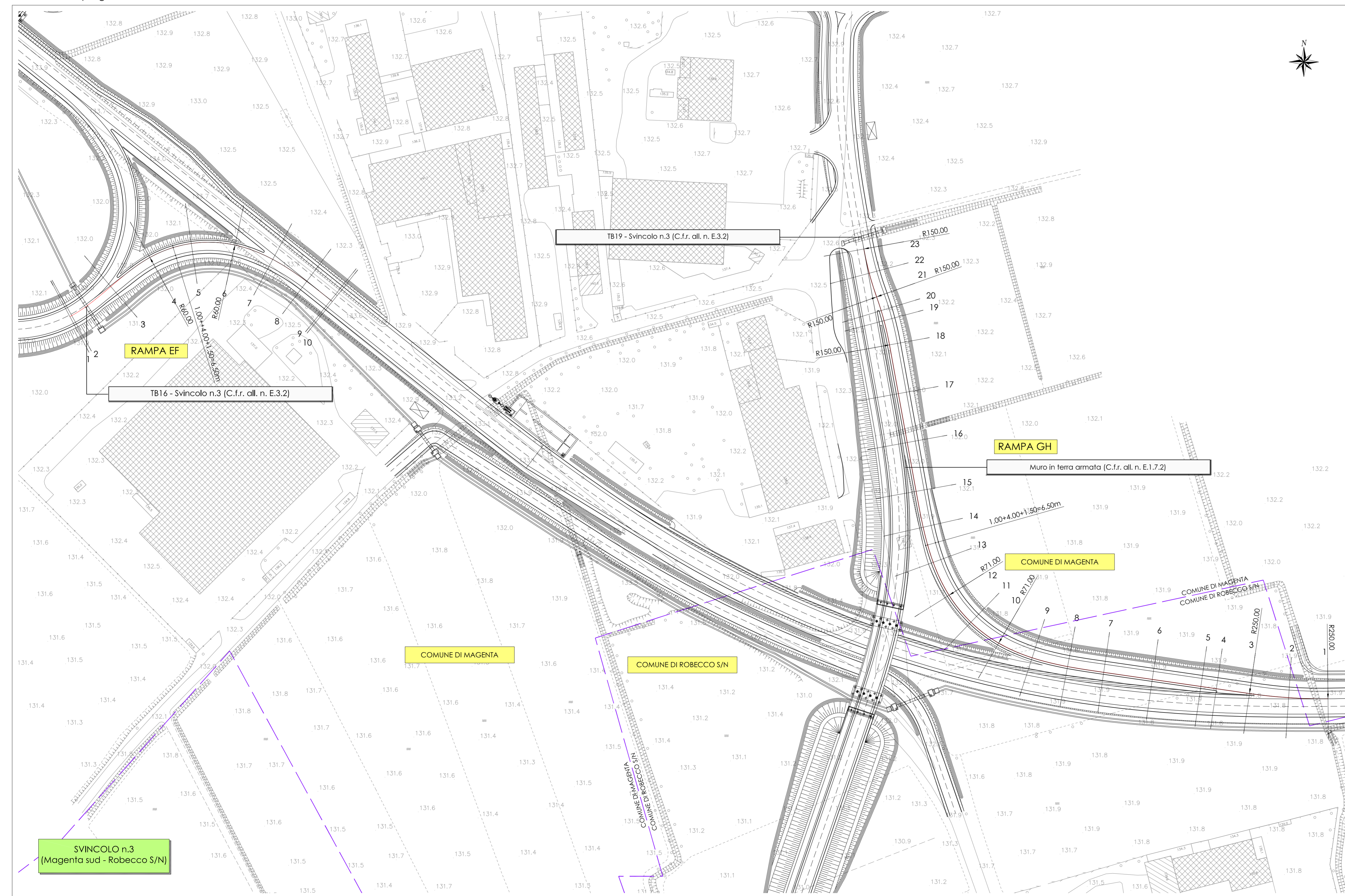
Planimetria di progetto Scala 1:1000
