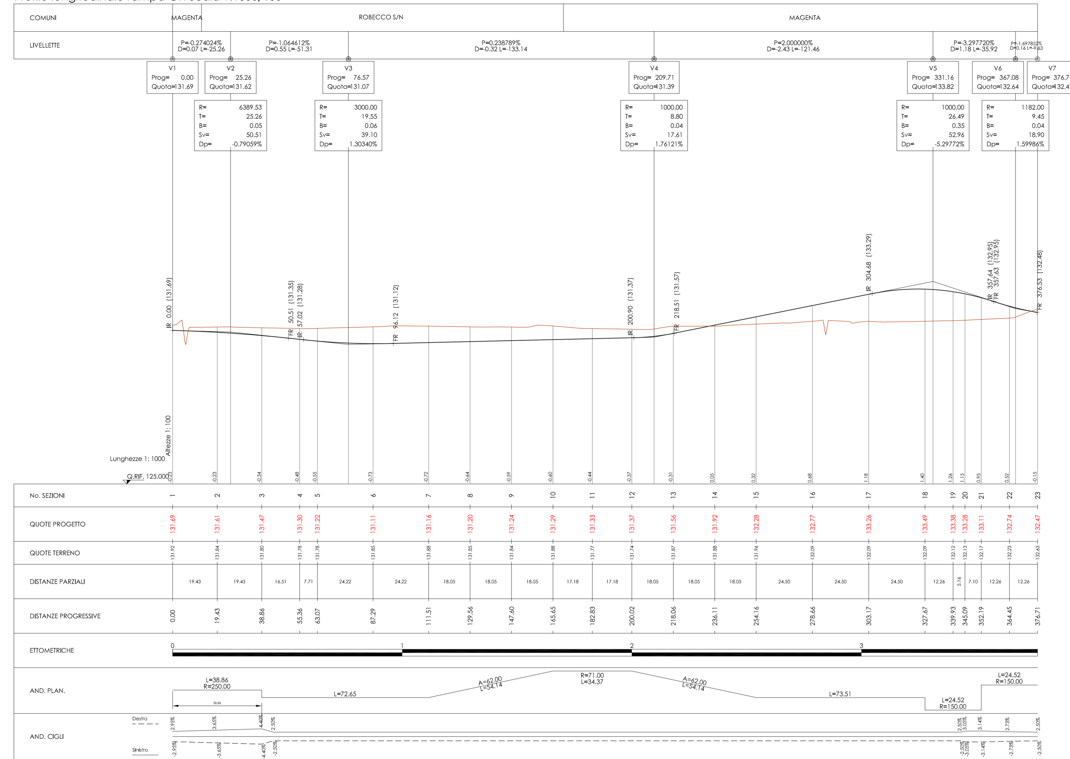
Profilo longitudinale rampa GH Scala 1:1000/100
