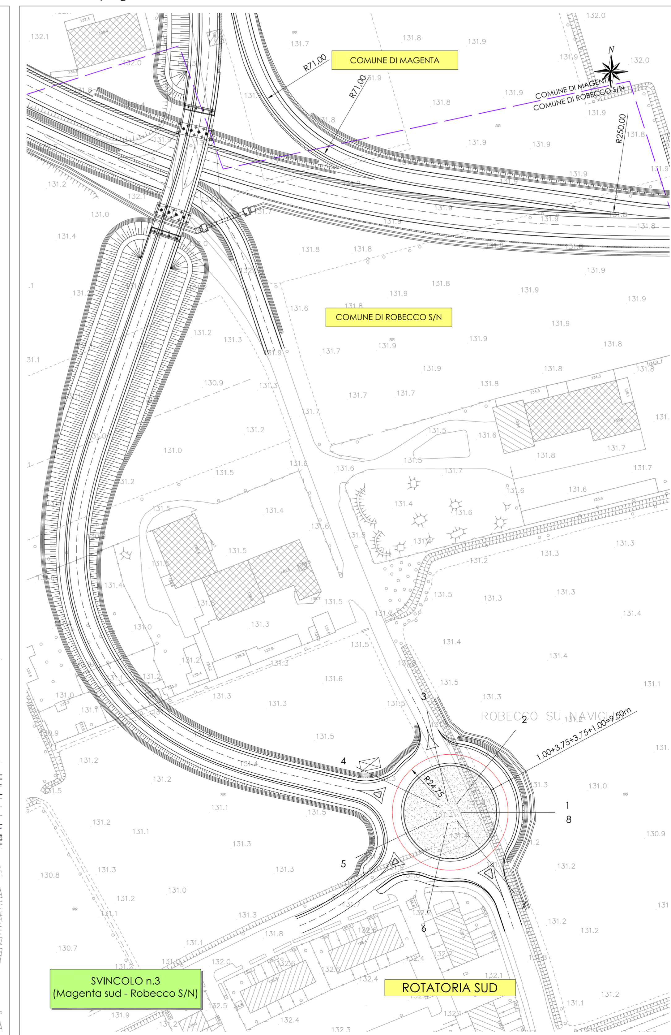
Planimetria di progetto Scala 1:1000
