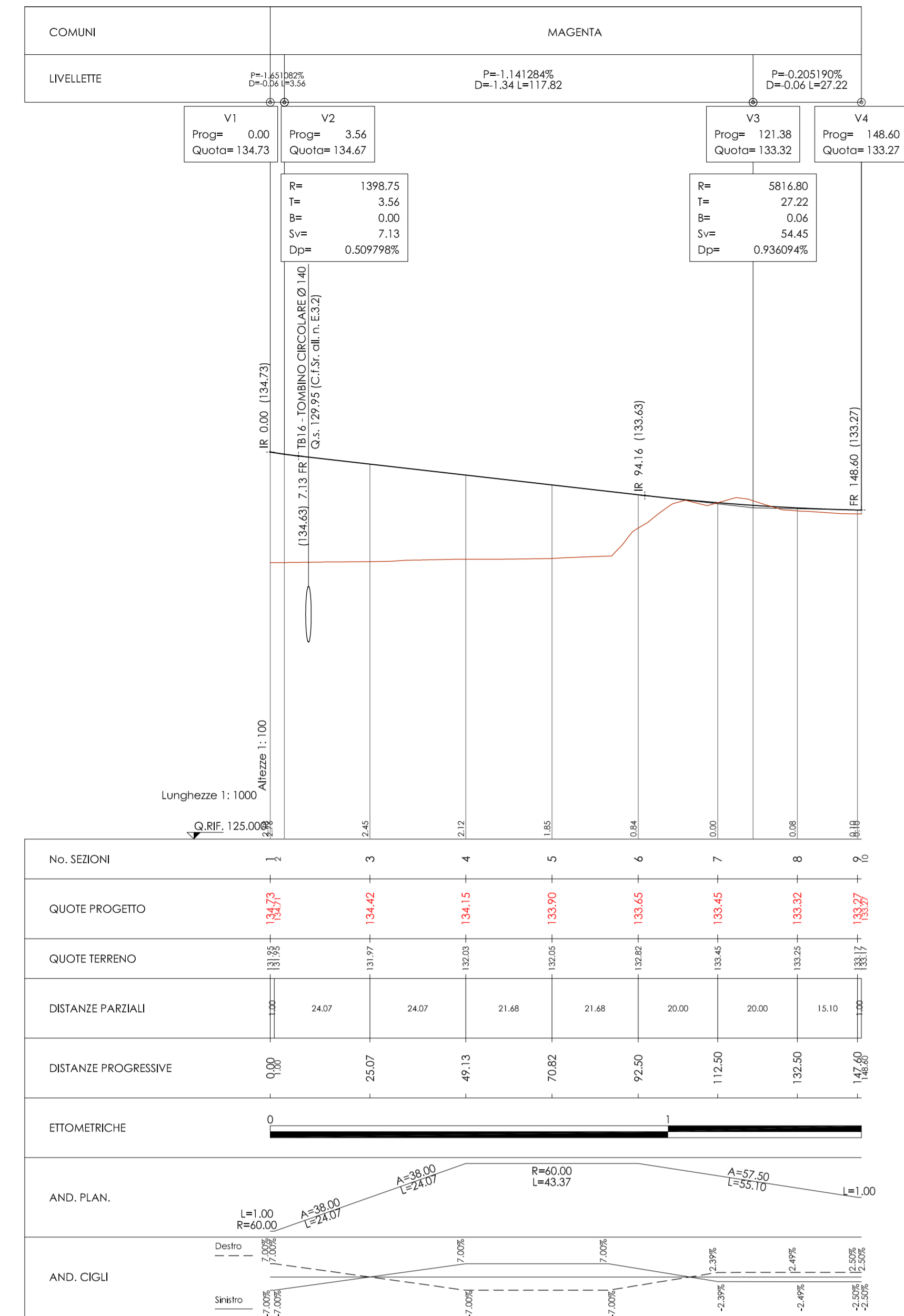
Profilo longitudinale rampa EF Scala 1:1000/100
