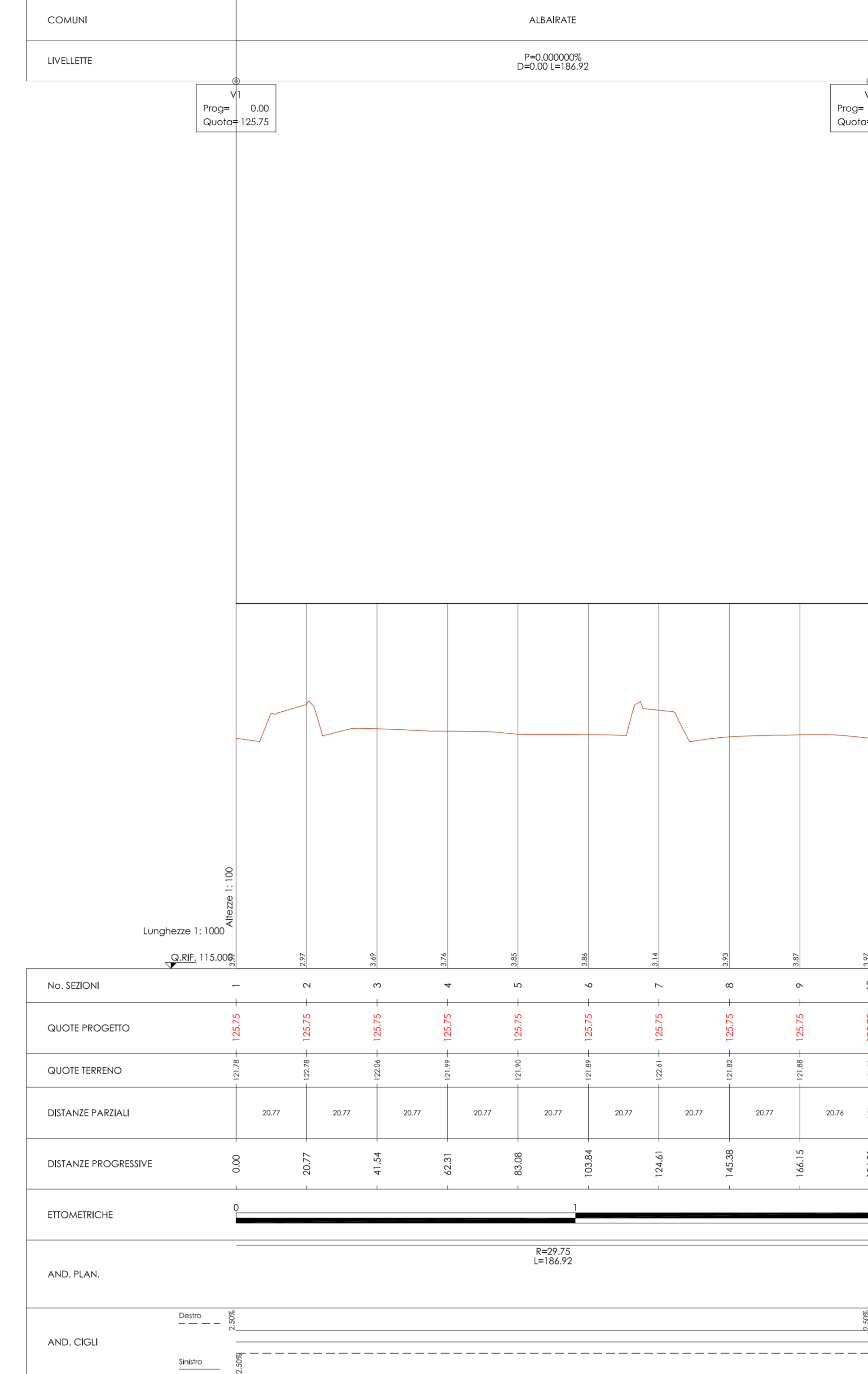
Profilo longitudinale rotonda Scala 1:1000/100
