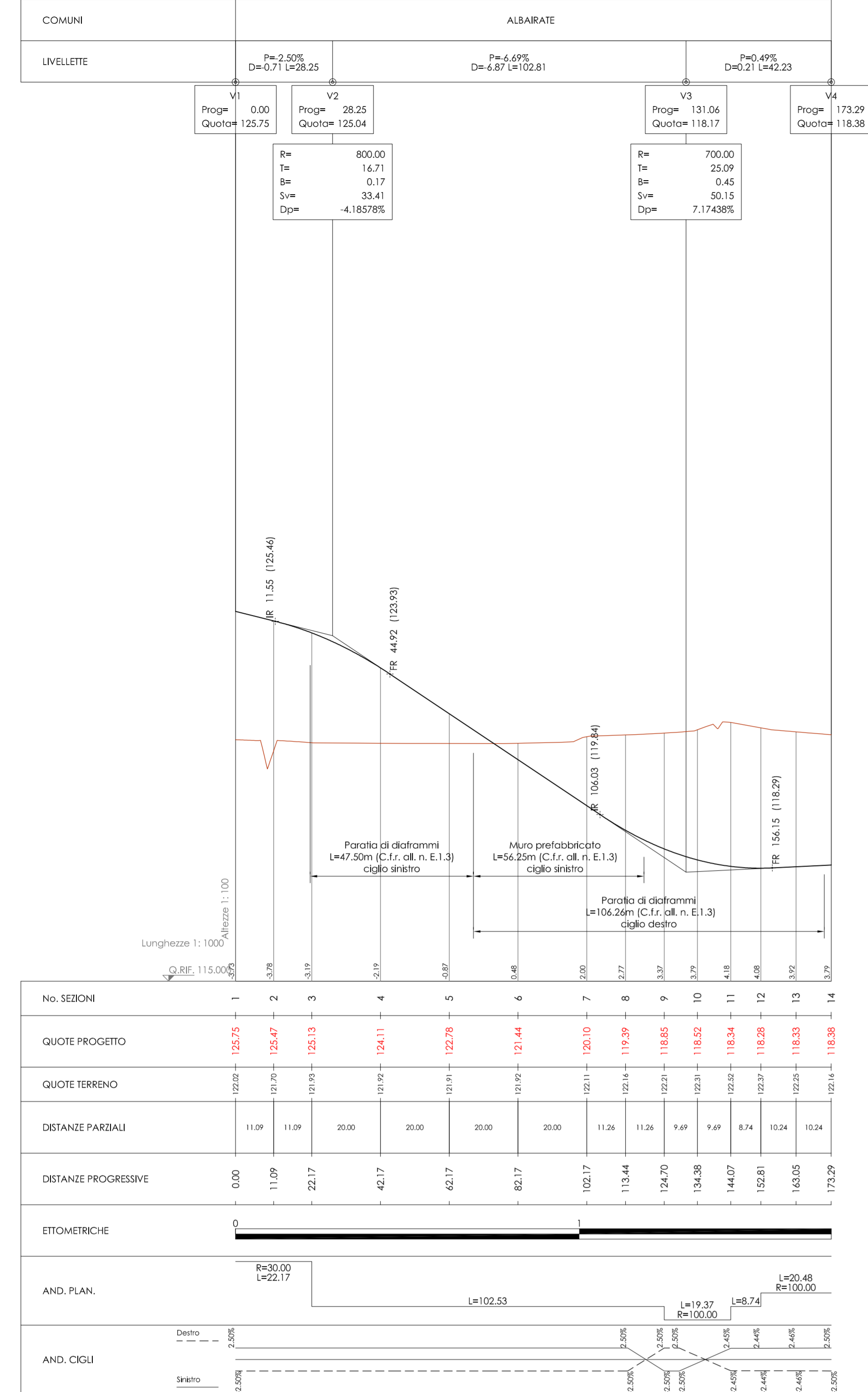
Profilo longitudinale rampa AB Scala 1:1000/100
