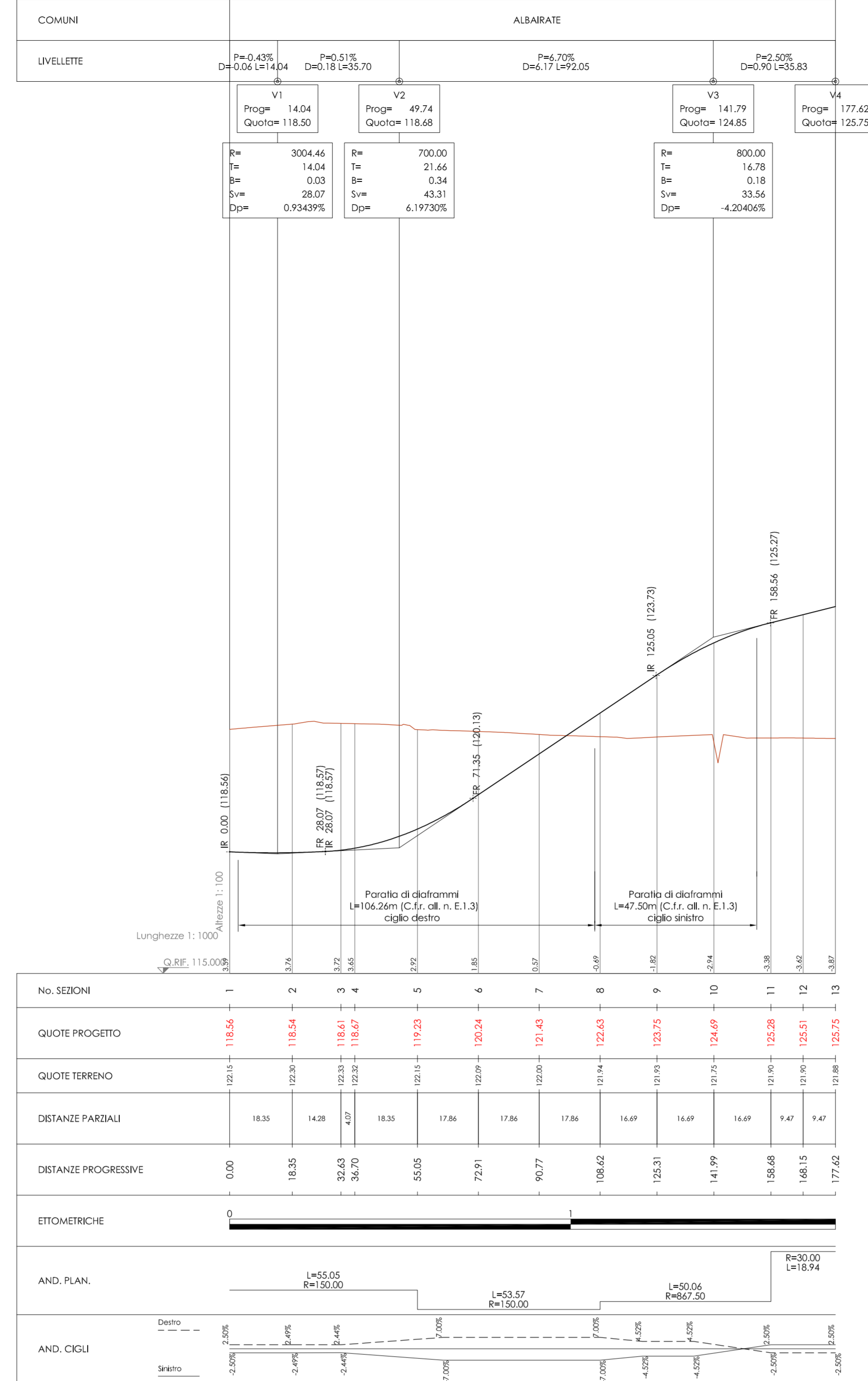
Profilo longitudinale rampa CD Scala 1:1000/100
