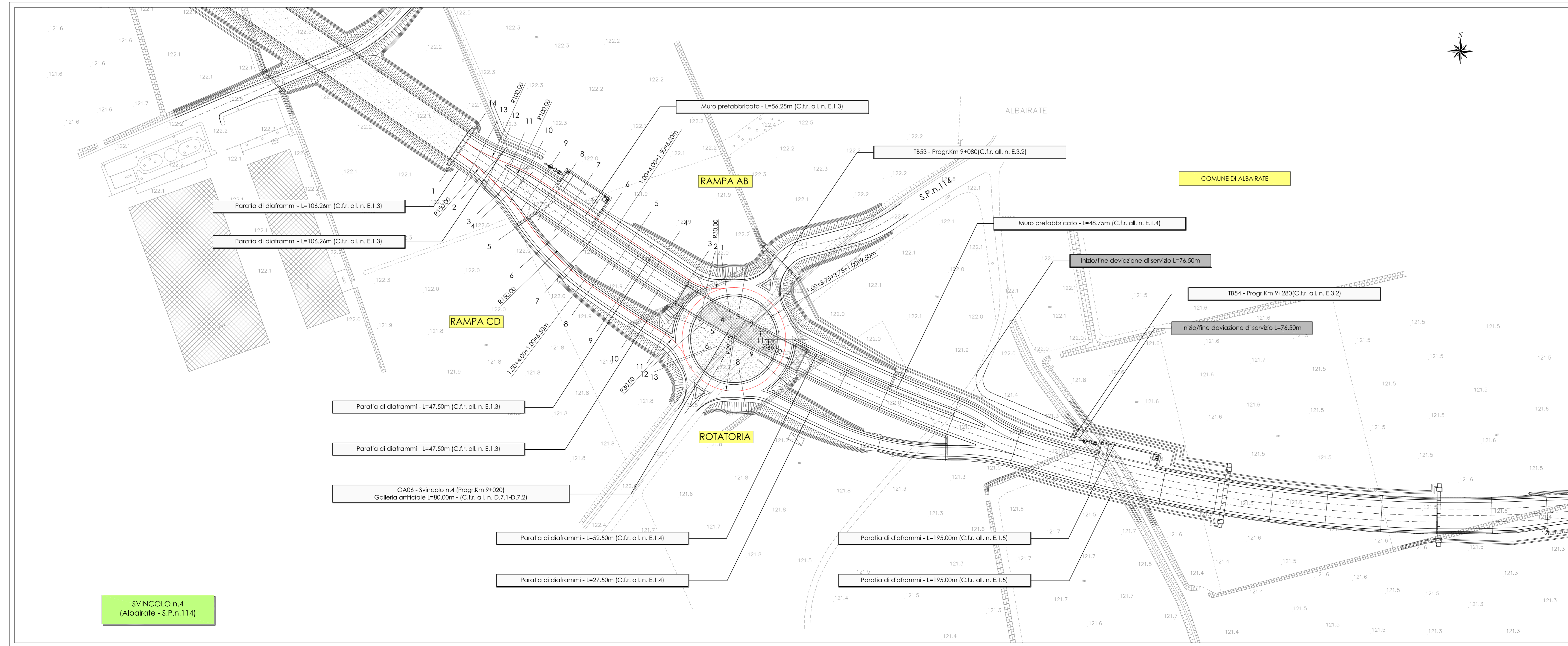
Planimetria di progetto Scala 1:1000
