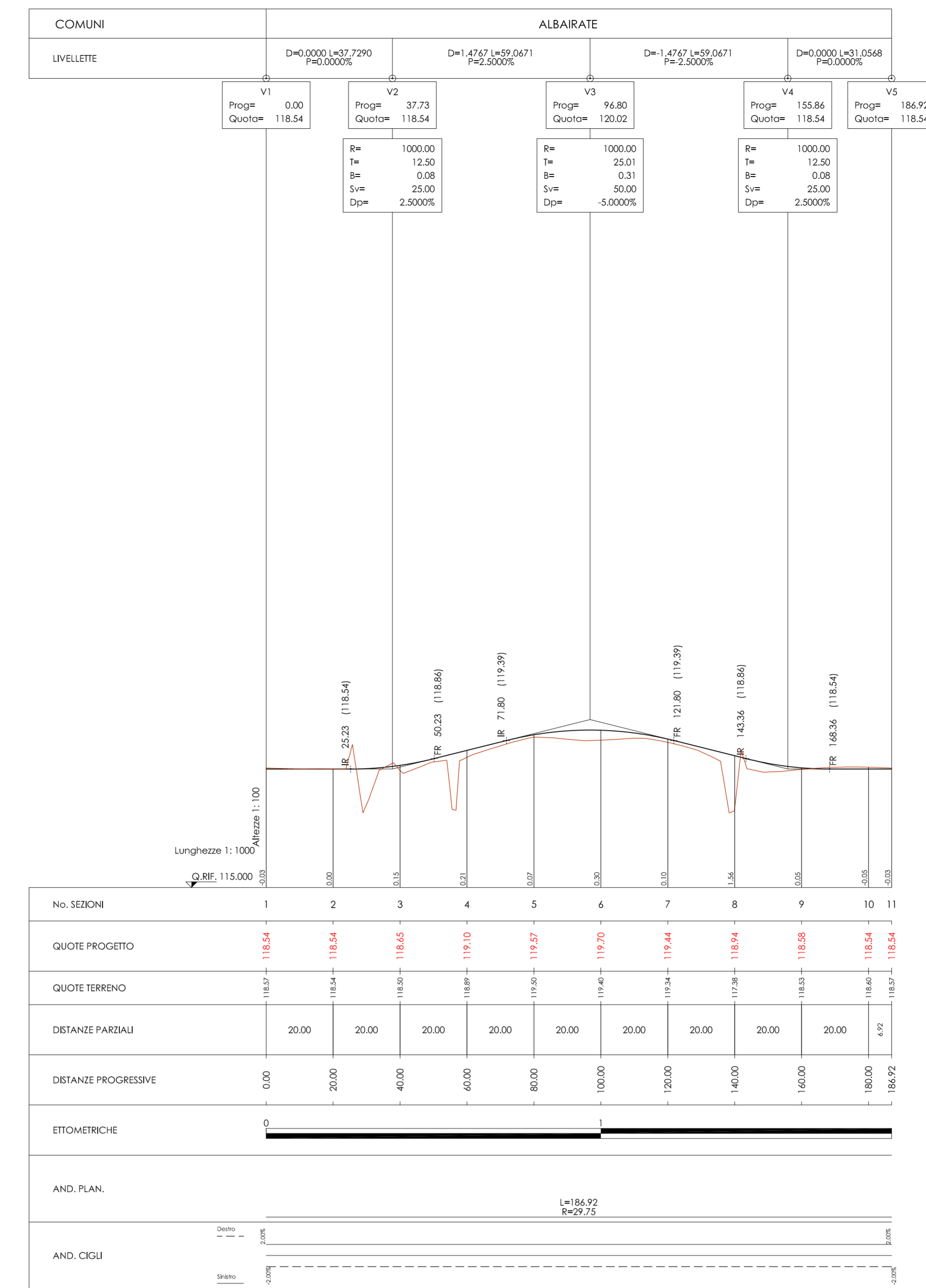
Profilo longitudinale rotatoria Scala 1:1000/100
