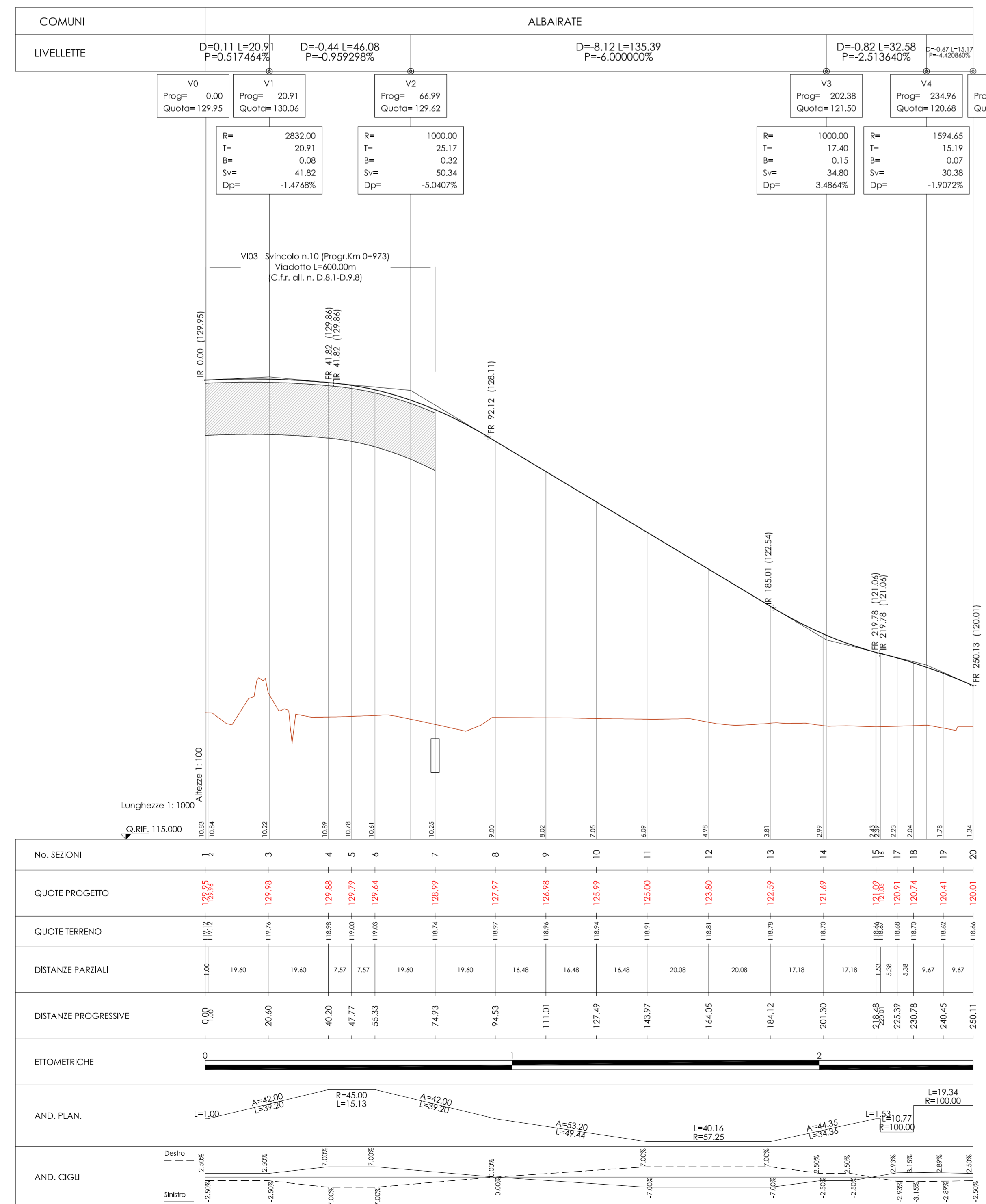
Profilo longitudinale Rampa CD Scala 1:1000/100
