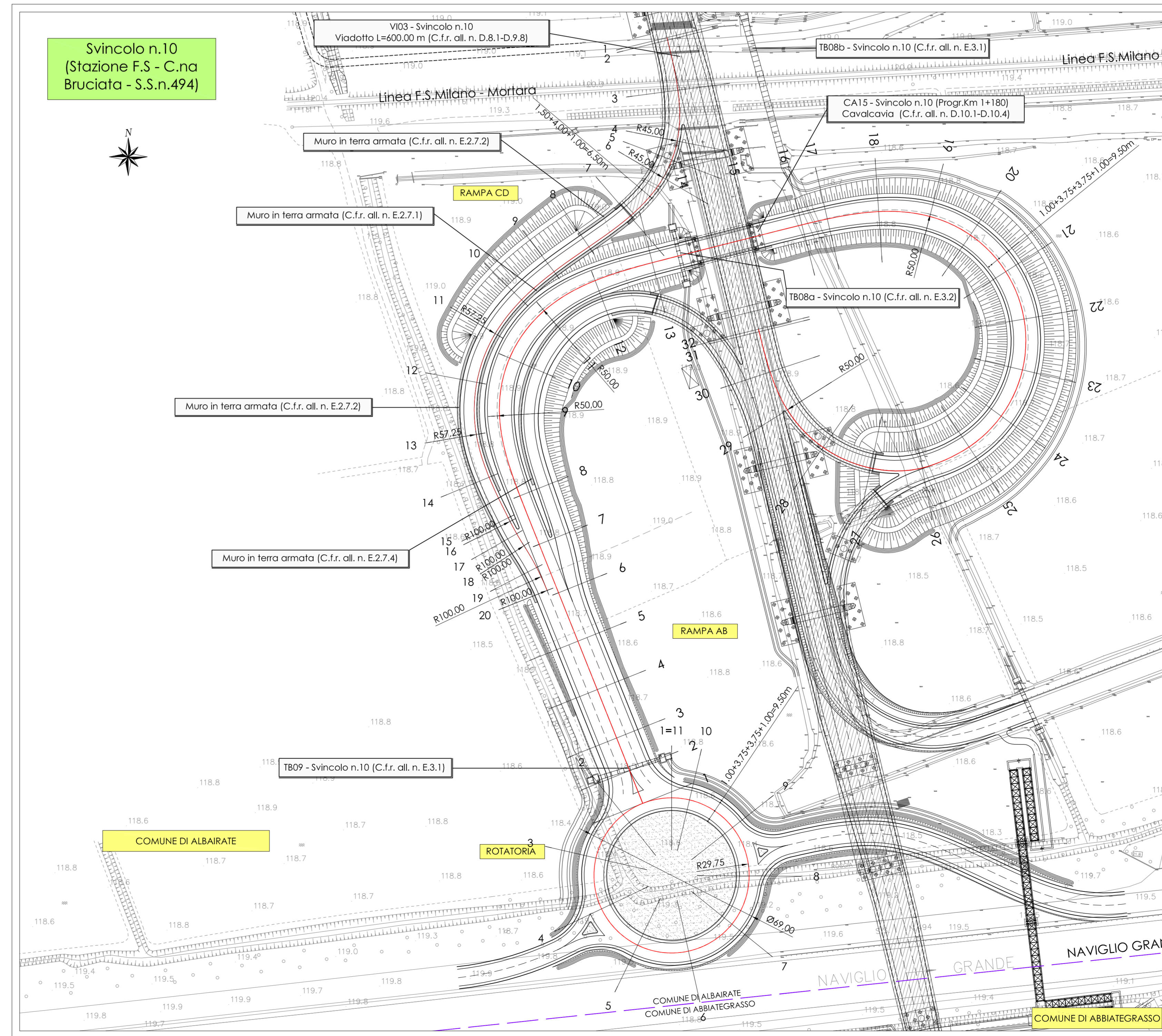
Planimetria di progetto Scala 1:1000
