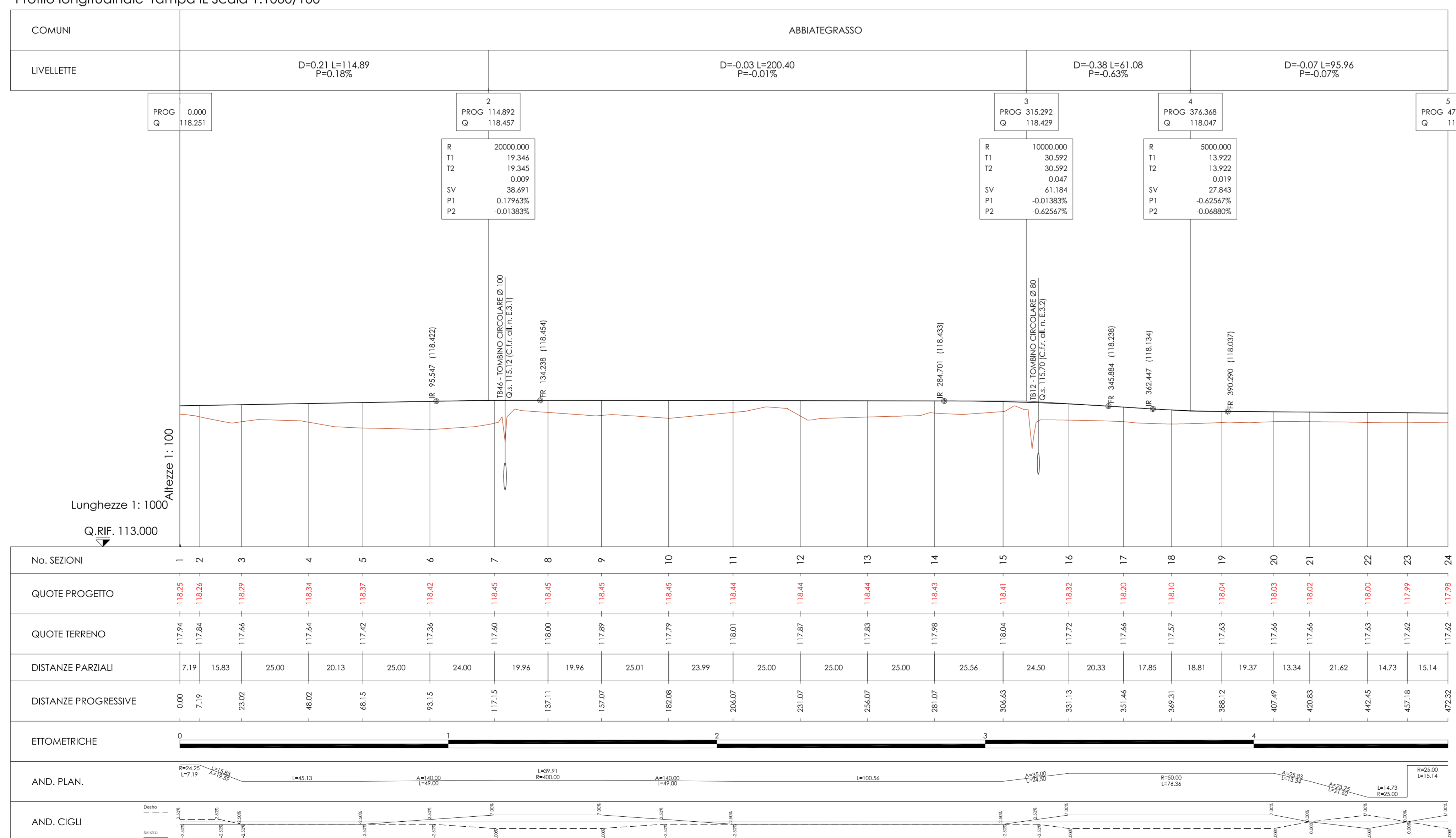
Profilo longitudinale rampa IL Scala 1:1000/100
