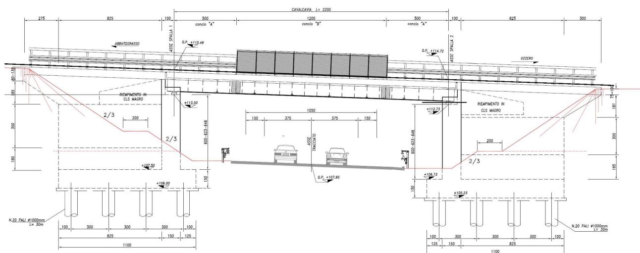
PROSPETTO LONGITUDINALE scala 1:100
