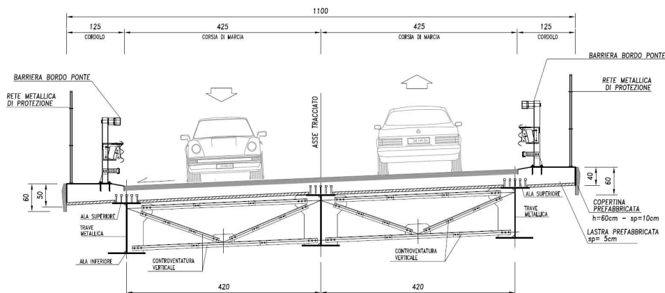
SEZIONE TRASVERSALE IMPALCATO scala 1:50
