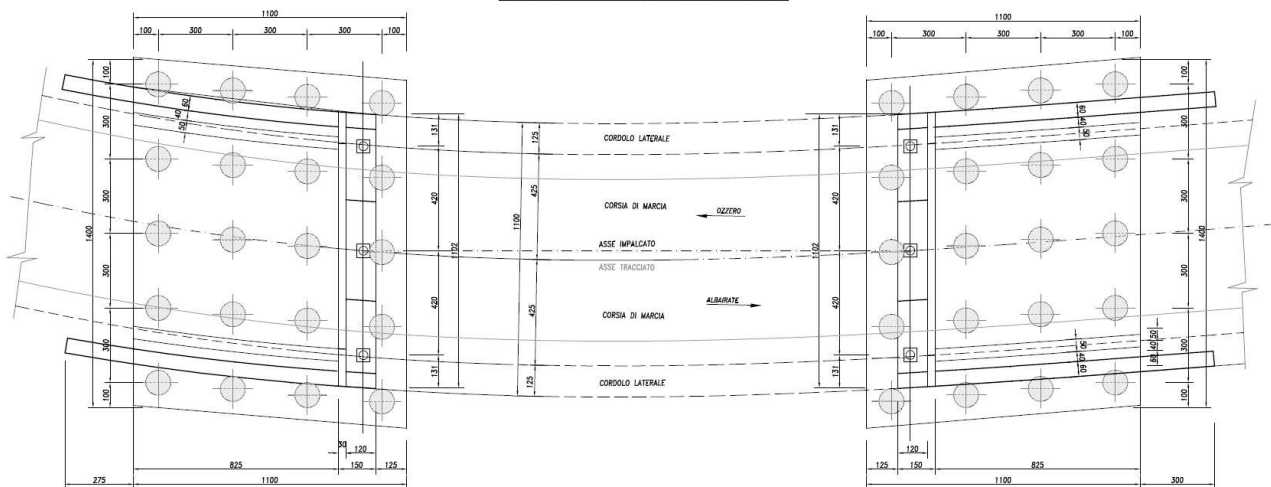
PIANTA SOTTOSTRUTTURE scala 1:100
