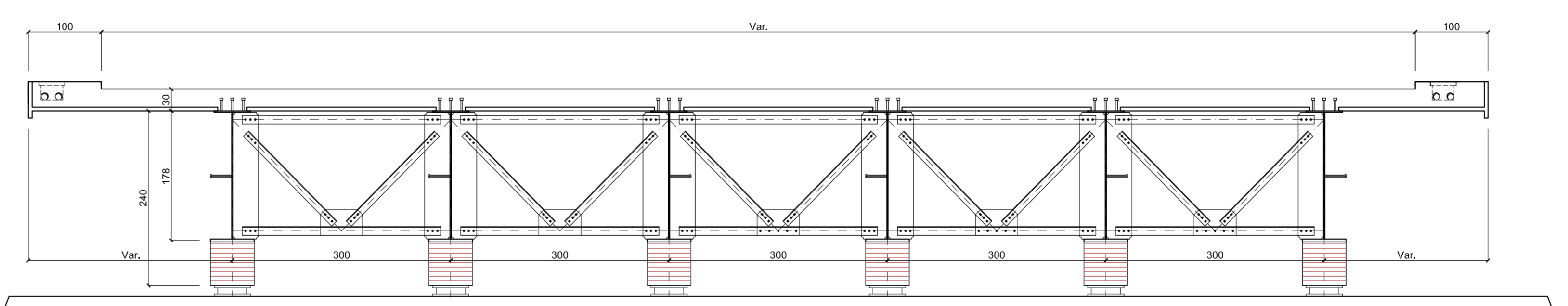
SEZIONE TRASVERSALE B-B (scala 1:50)
