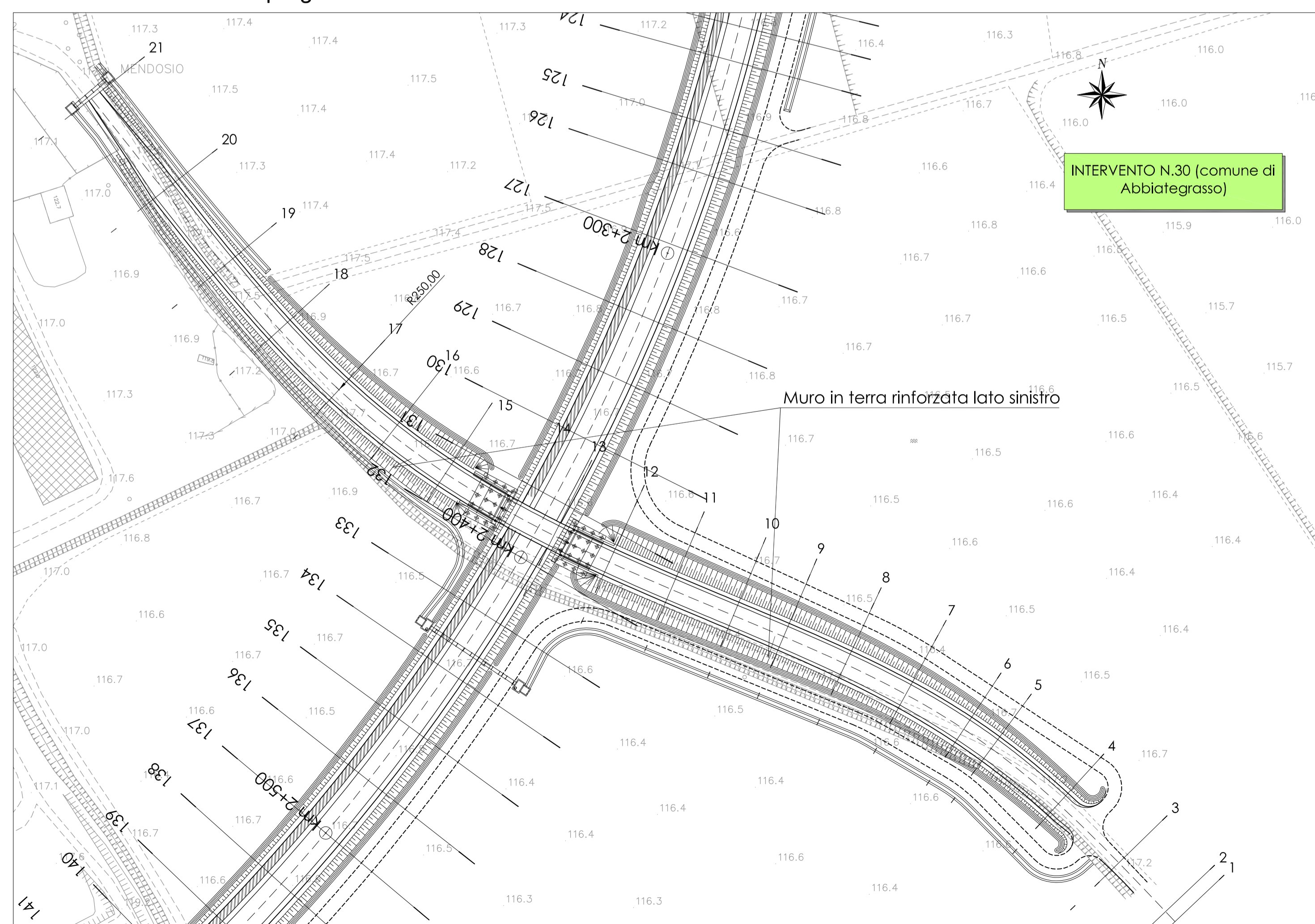
Planimetria di progetto Scala 1:1000
