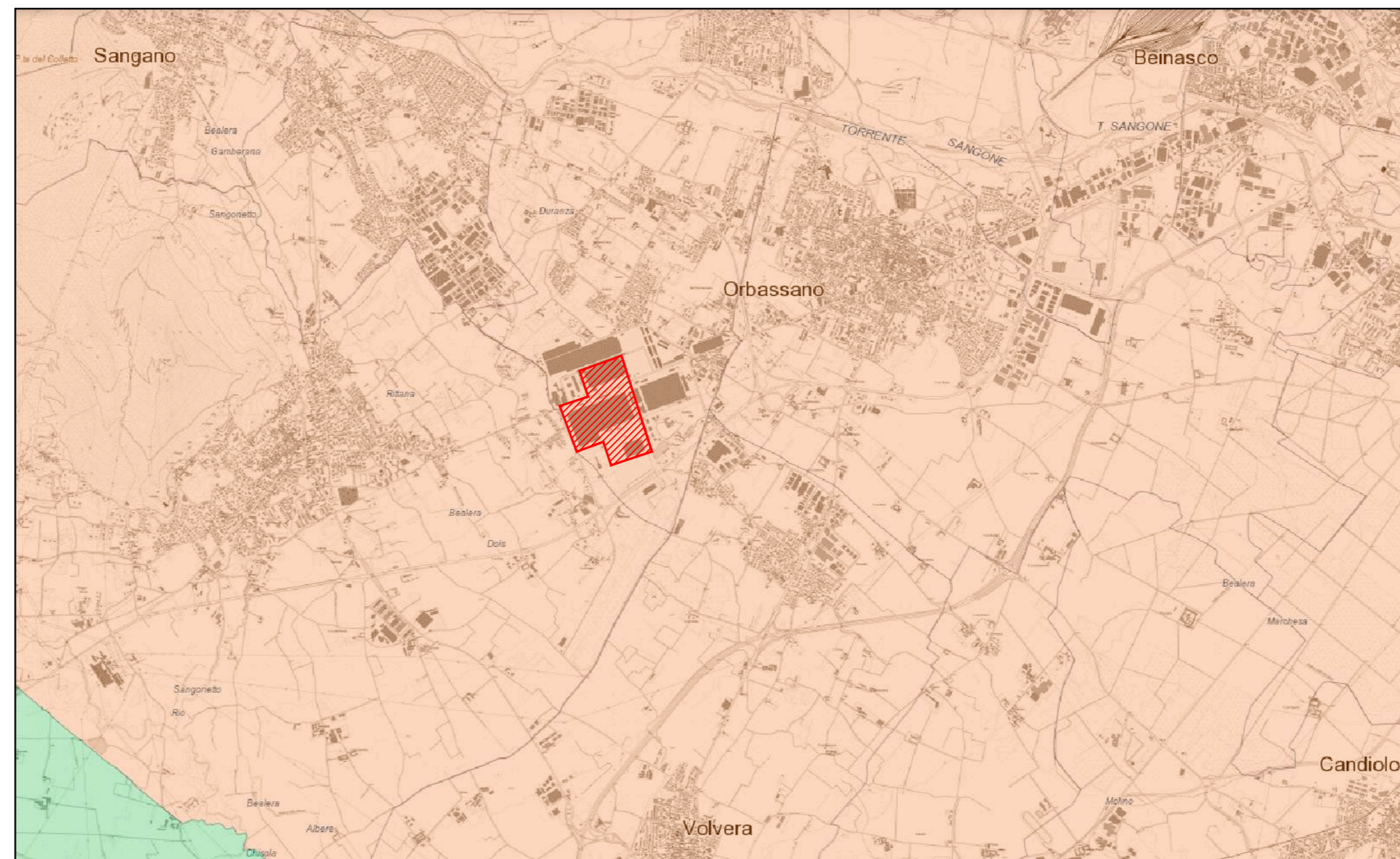
AREE DI SUPERAMENTO DEI LIMITI DI QUALITÀ DELL'ARIA SCALA 1:50.000
