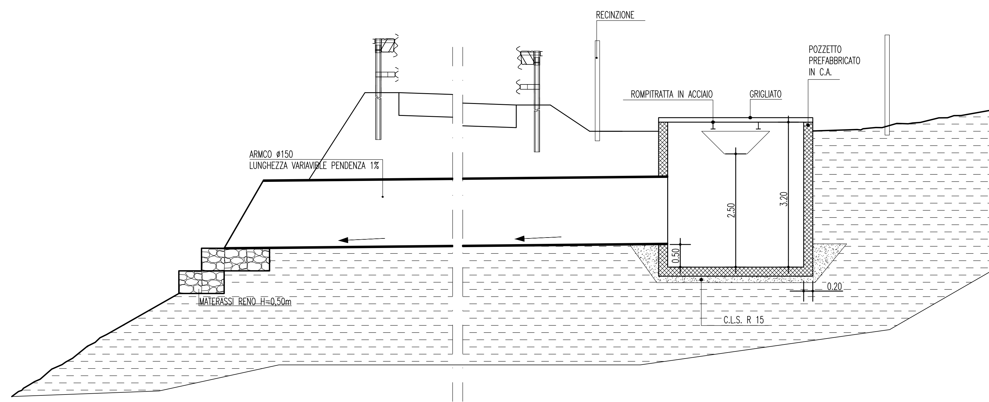
SEZIONE A-A'
