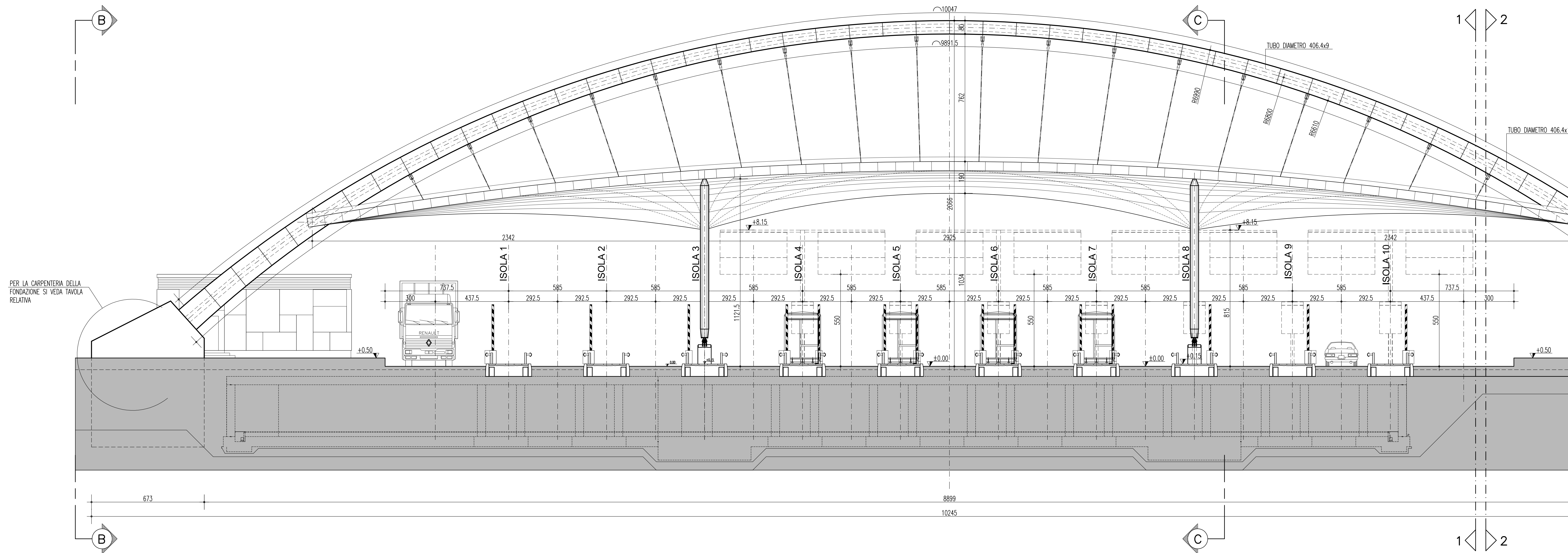
PROSPETTO A-A (1) SCALA 1:100
