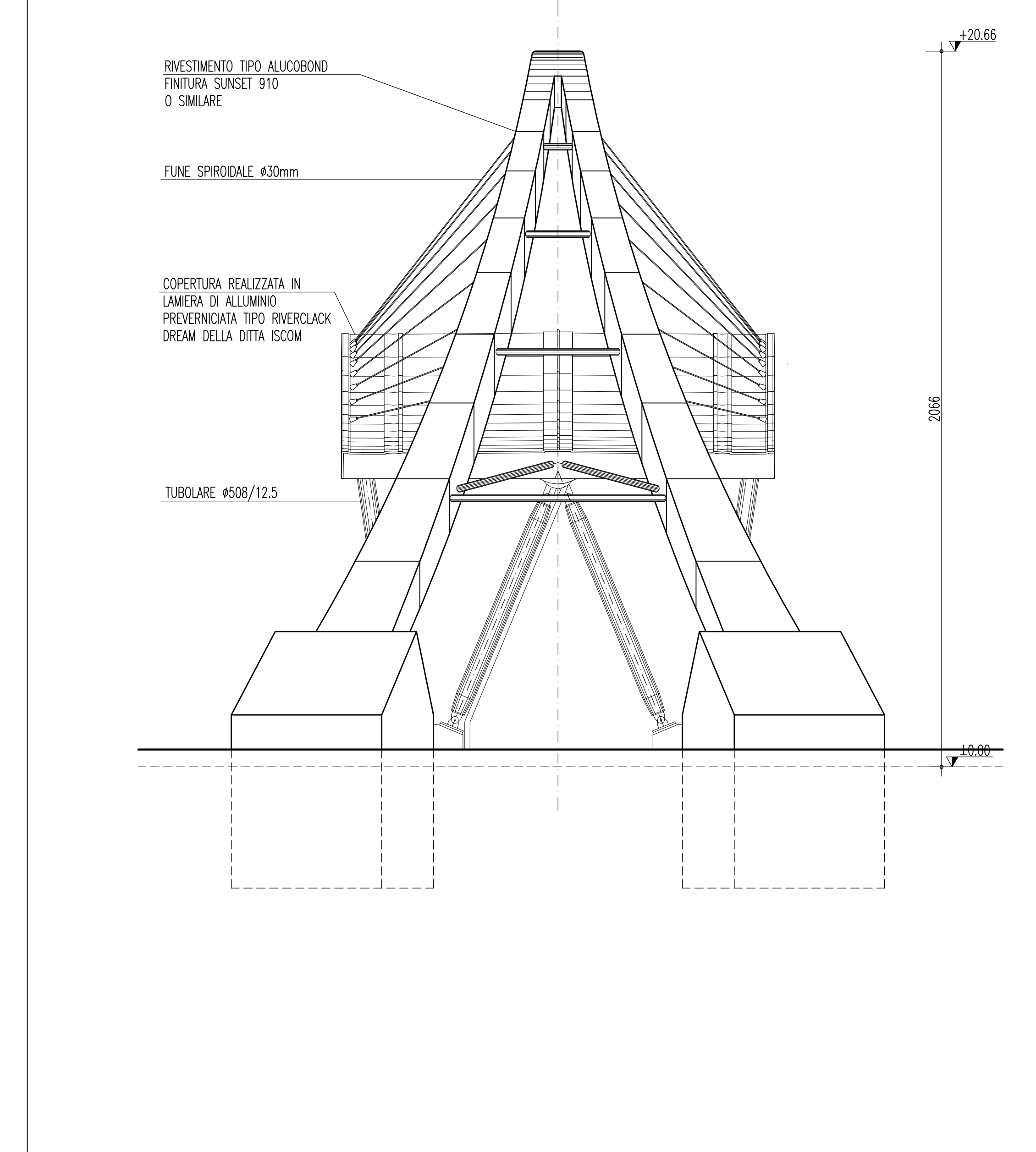
PROSPETTO B-B SCALA 1:100
