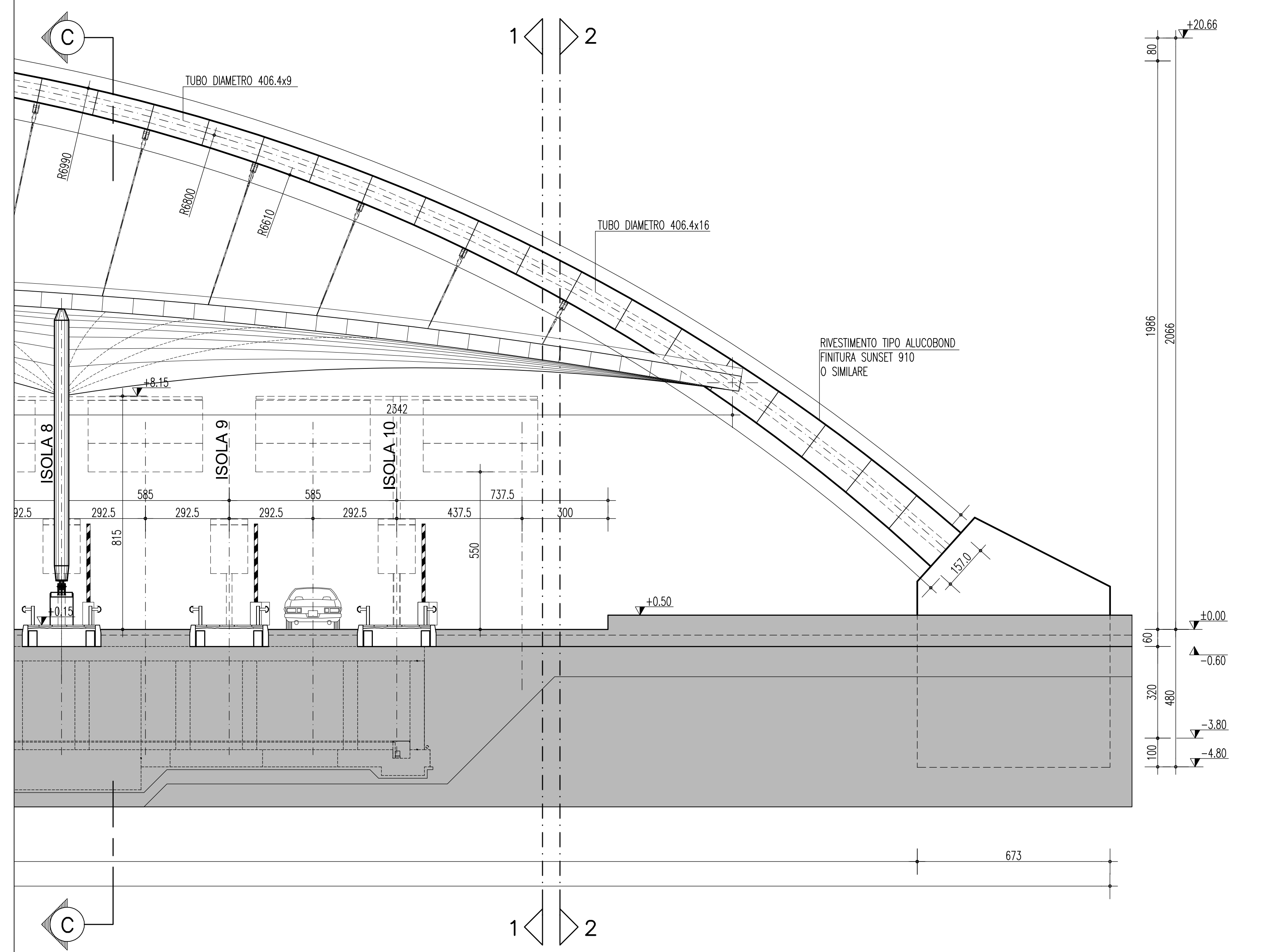
PROSPETTO A-A (2) SCALA 1:100
