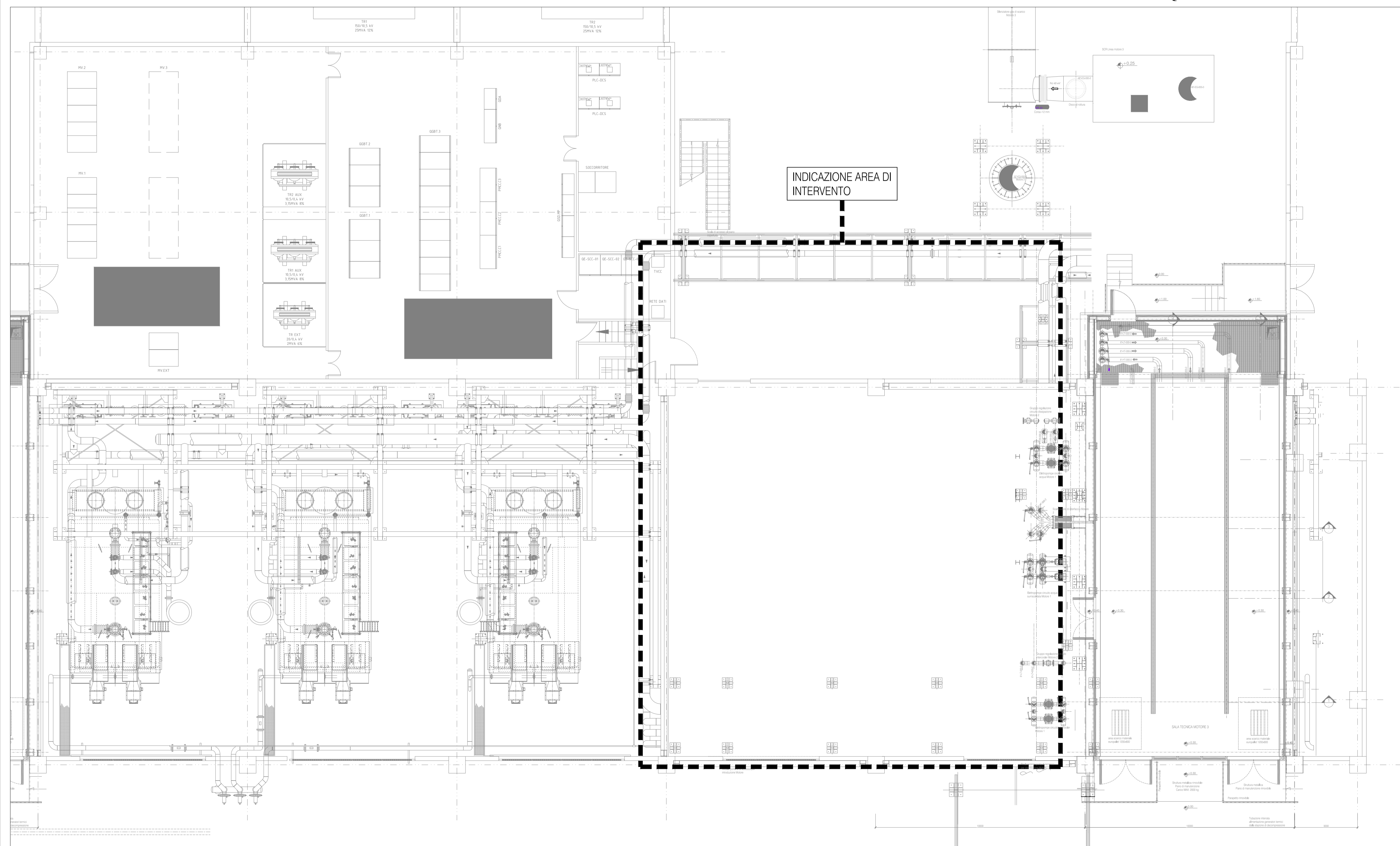
PLANIMETRIA GENERALE EDIFICIO TECNOLOGICO - AREE DI INTERVENTO - PIANI Q.TA +0.30 - SCALA 1:100
