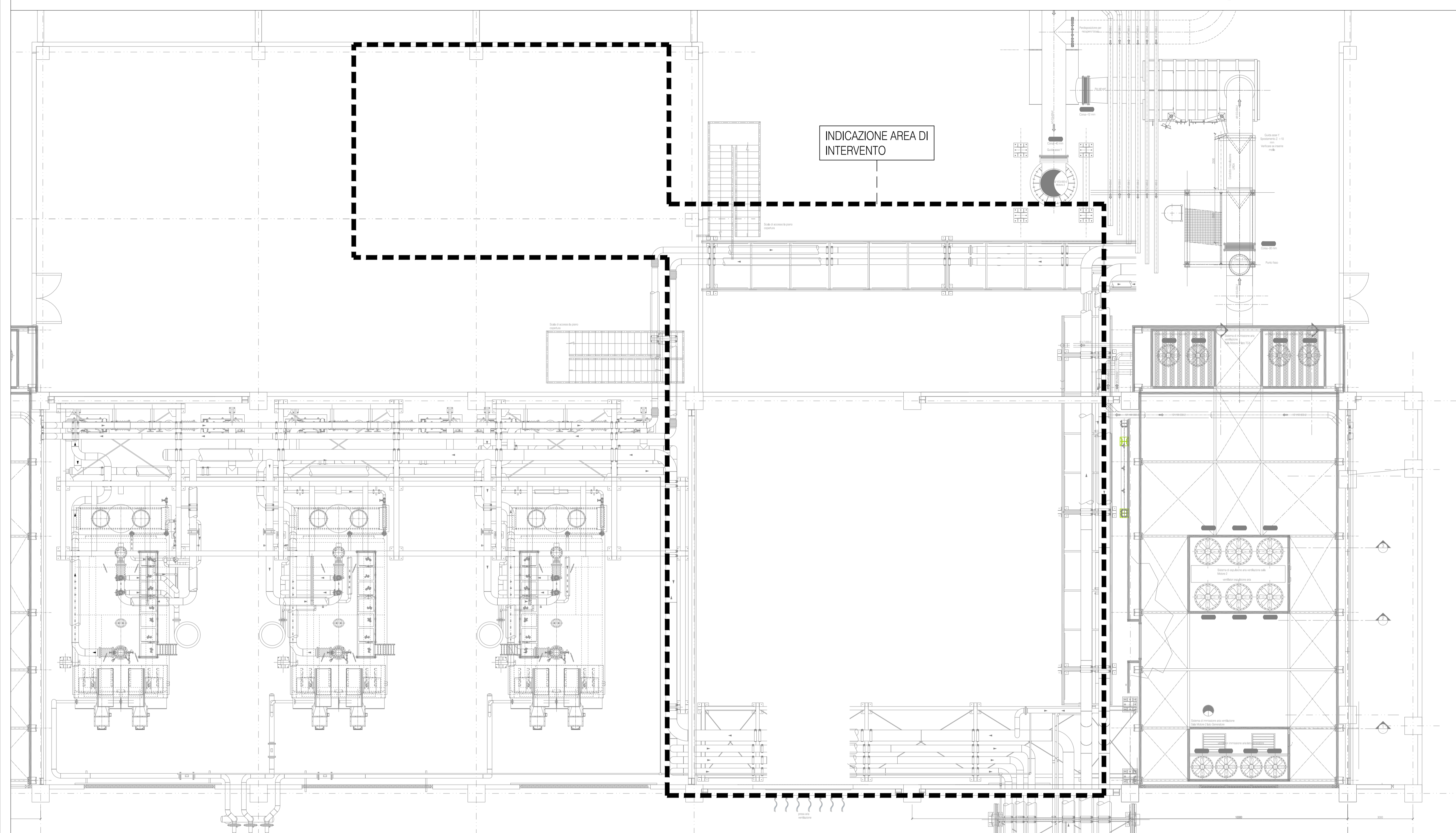
PLANIMETRIA GENERALE EDIFICIO TECNOLOGICO - AREE DI INTERVENTO - PIANI Q.TA +0.30 - SCALA 1:100
