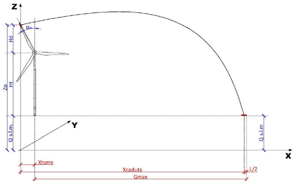
Figura 3 - Modello geometrico della rottura di un frammento di pala
