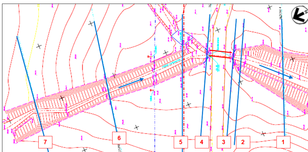
Figura 4.2/B – Planimetria con localizzazione delle sezioni. La sezione n. 5 corrisponde all'attraversamento del metanodotto.
