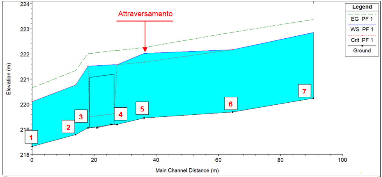
Figura 4.3/A – Output del programma con sezione del tratto modellato
