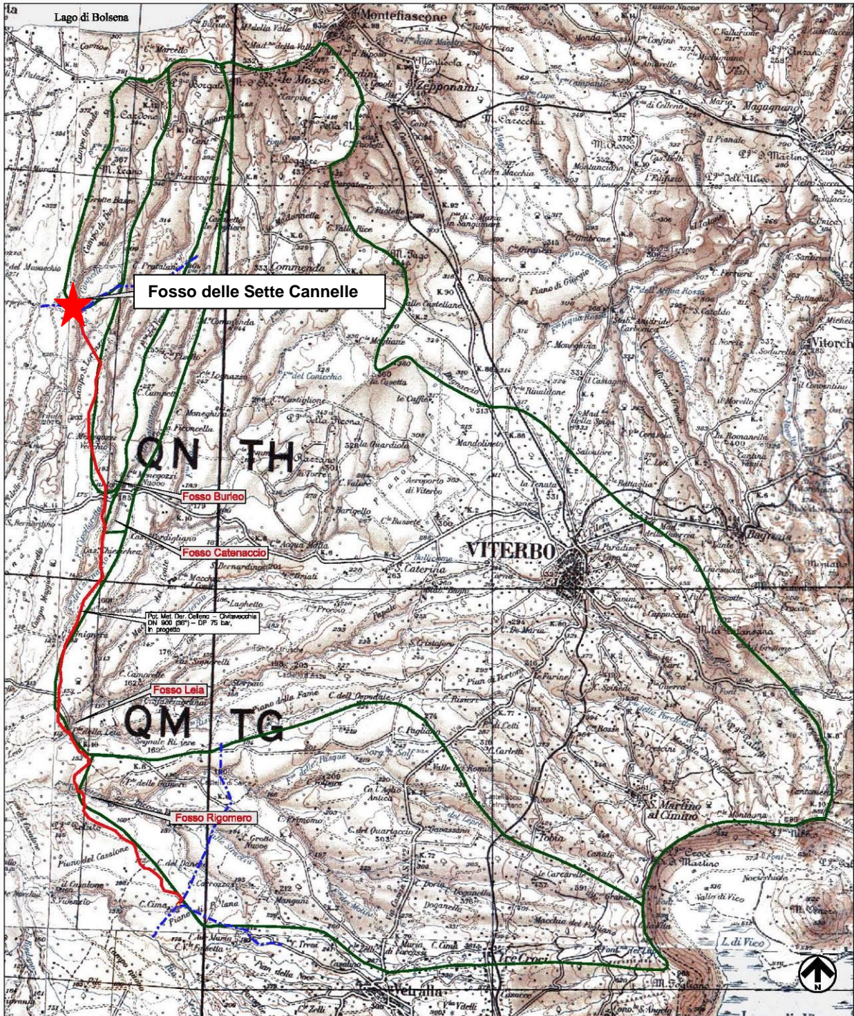
Figura 3.1/A – Corografia con rappresentati i bacini dei corsi d'acqua attraversati dal metanodotto. Evidenziato il F.so delle Sette Cannelle
