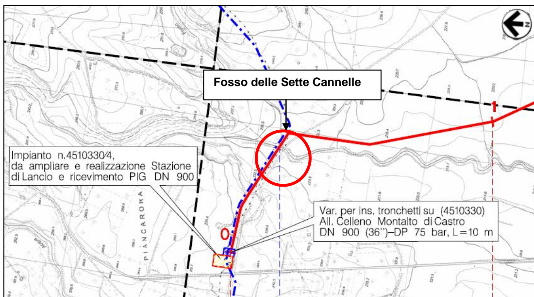
Figura 2/B – Stralcio planimetrico con localizzazione dell'attraversamento del F.sso delle Sette Cannelle
