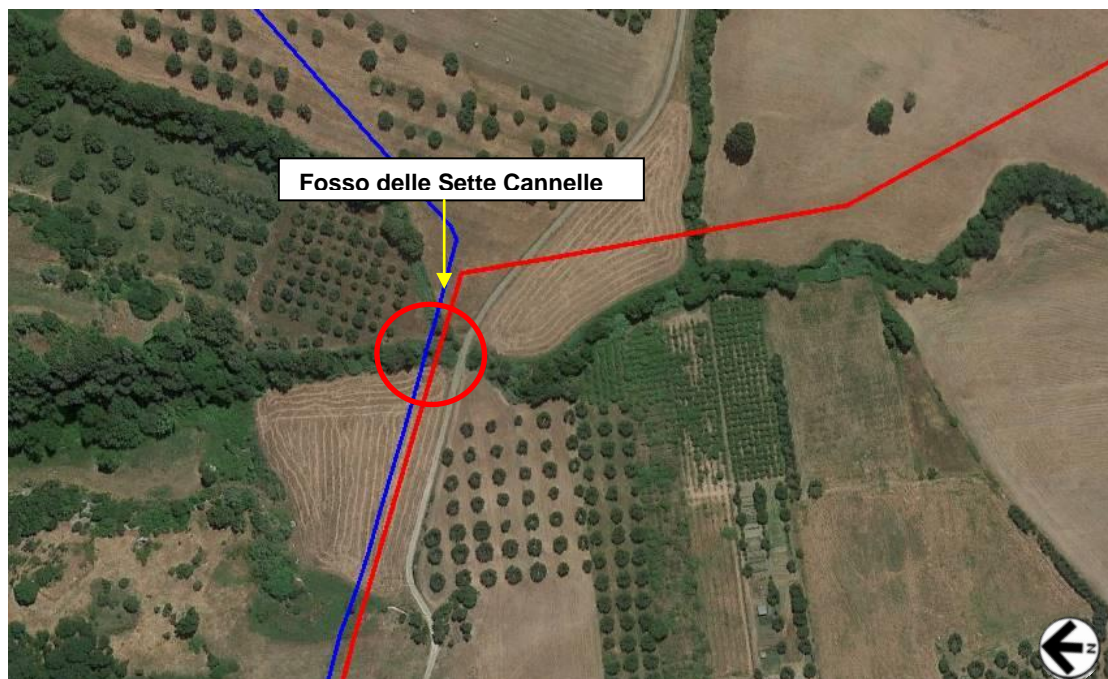
Figura 2/C – Immagine aerea con localizzazione dell'attraversamento del F.sso delle Sette Cannelle (linea rossa: tracciato del metanodotto in progetto) (su base Google Earth)
