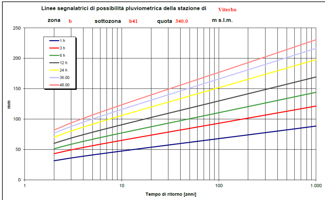
Figura 3.4.2/A – Curve segnalatrici di possibilità pluviometrica della stazione di Viterbo
