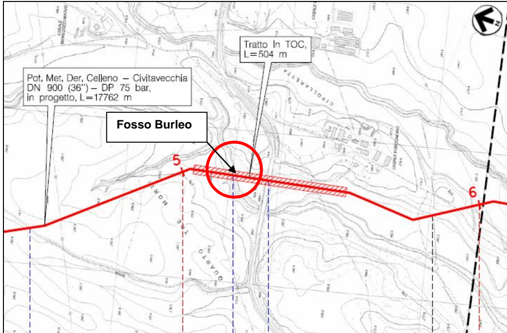
Figura 2/B – Stralcio planimetrico con localizzazione dell'attraversamento in TOC del F.sso Burleo
