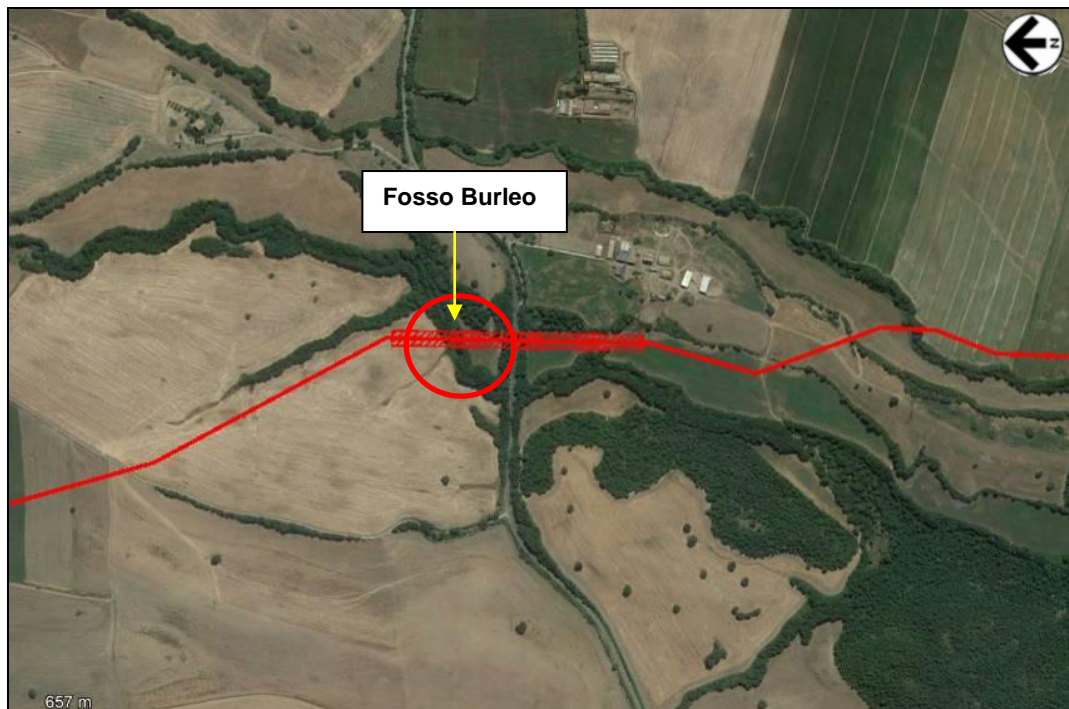
Figura 2/C – Immagine aerea con localizzazione dell'attraversamento in TOC del F.sso Burleo (su base Google Earth)
