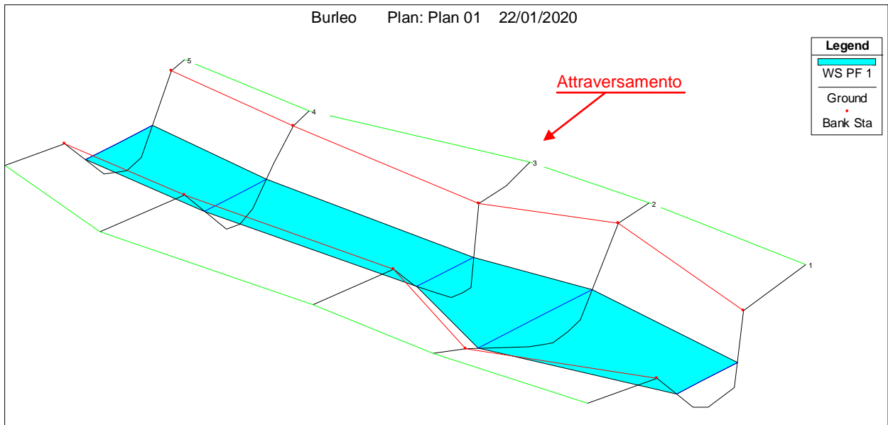
Figura 4.1.3/A – Vista assometrica del tratto modellato
