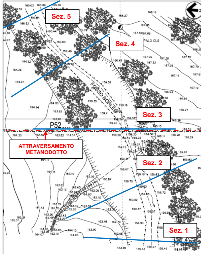
Figura 4.1.2/B – Planimetria del tratto di corso modellato con riportate le sezioni di studio
