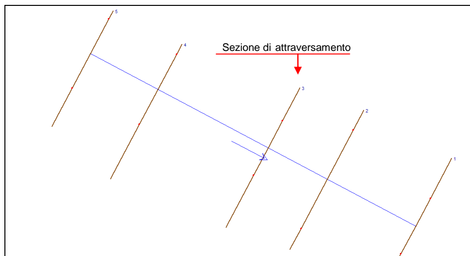
Figura 4.1.2/A – Schema delle sezioni utilizzate nella modellazione idraulica
