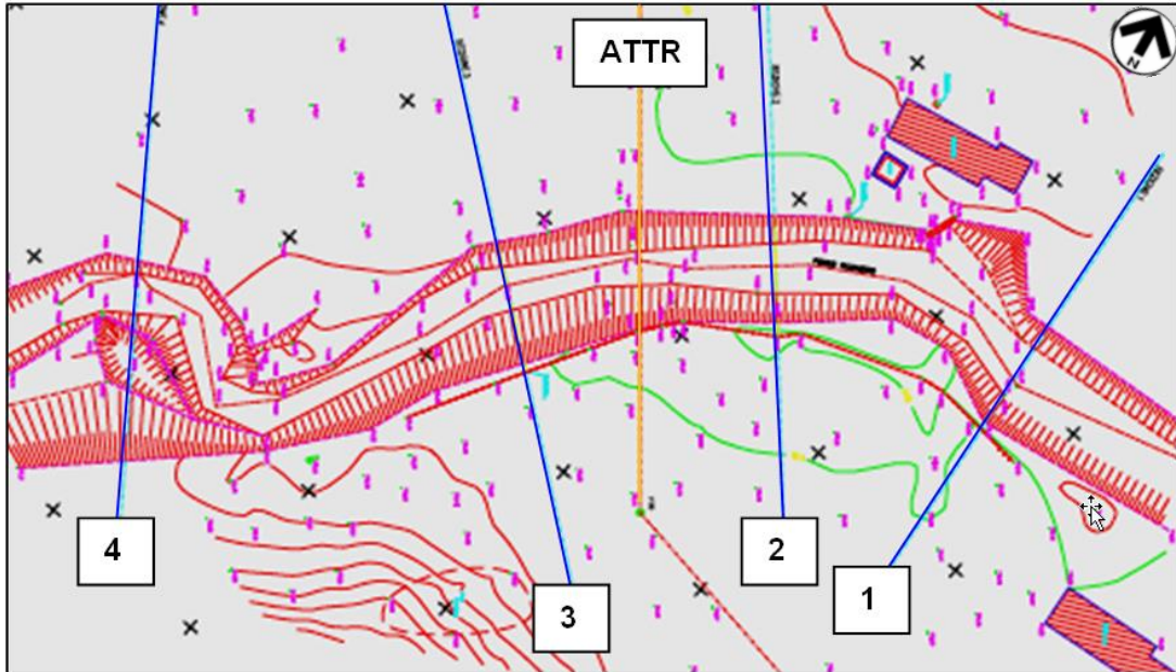
Figura 4.2/A – Schema planimetrico delle sezioni utilizzate per la modellazione
