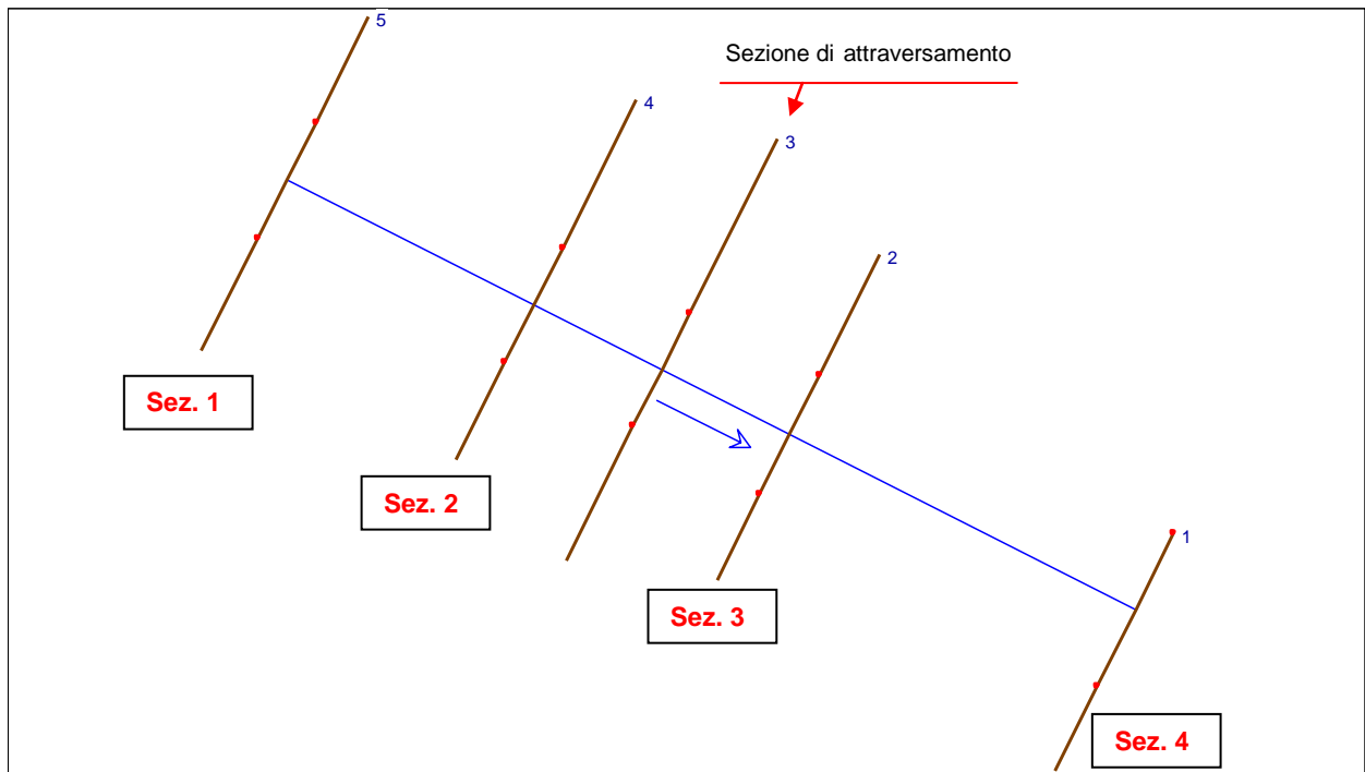
Figura 4.2/B – Schema delle sezioni utilizzate nella modellazione idraulica
