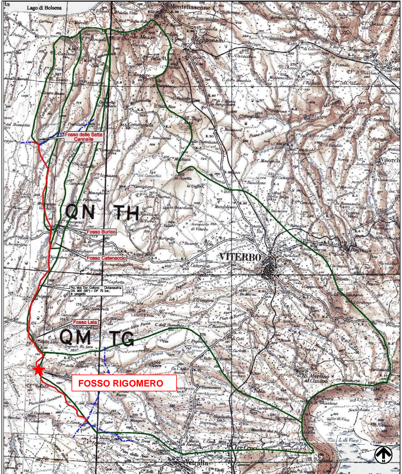
Figura 3.1/A – Planimetria con localizzazione dei fossi interferenti con il tracciato (tratto rosso) e relativi bacini idrografici. Evidenziato il fosso Rigomero.
