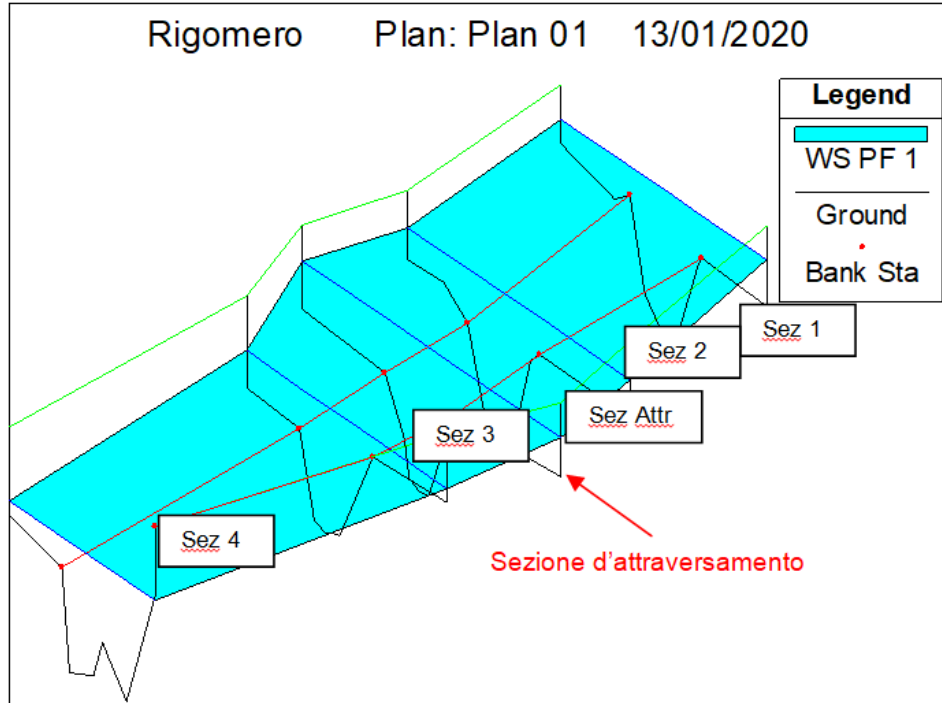
Figura 4.3/A – Vista assometrica del tratto modellato
