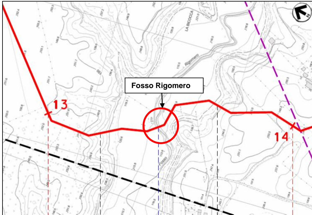
Figura 2/B – Stralcio planimetrico con localizzazione dell'attraversamento (progr. Km 13+436)
