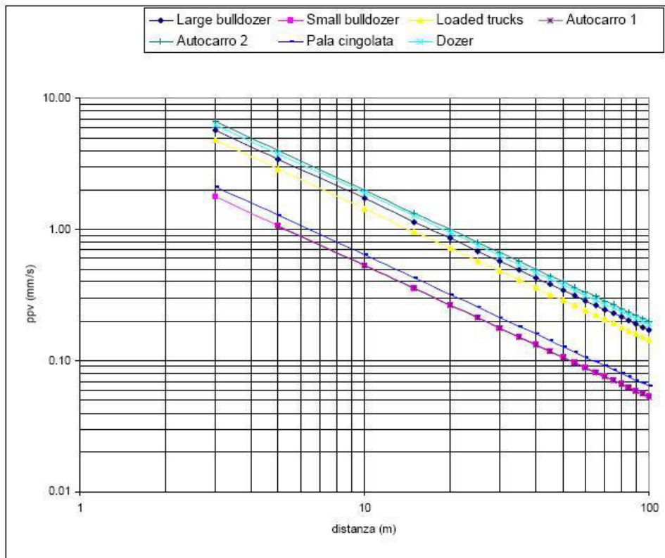
Propagazione della vibrazione indotta mezzi per scavi di scotico e bonifica
