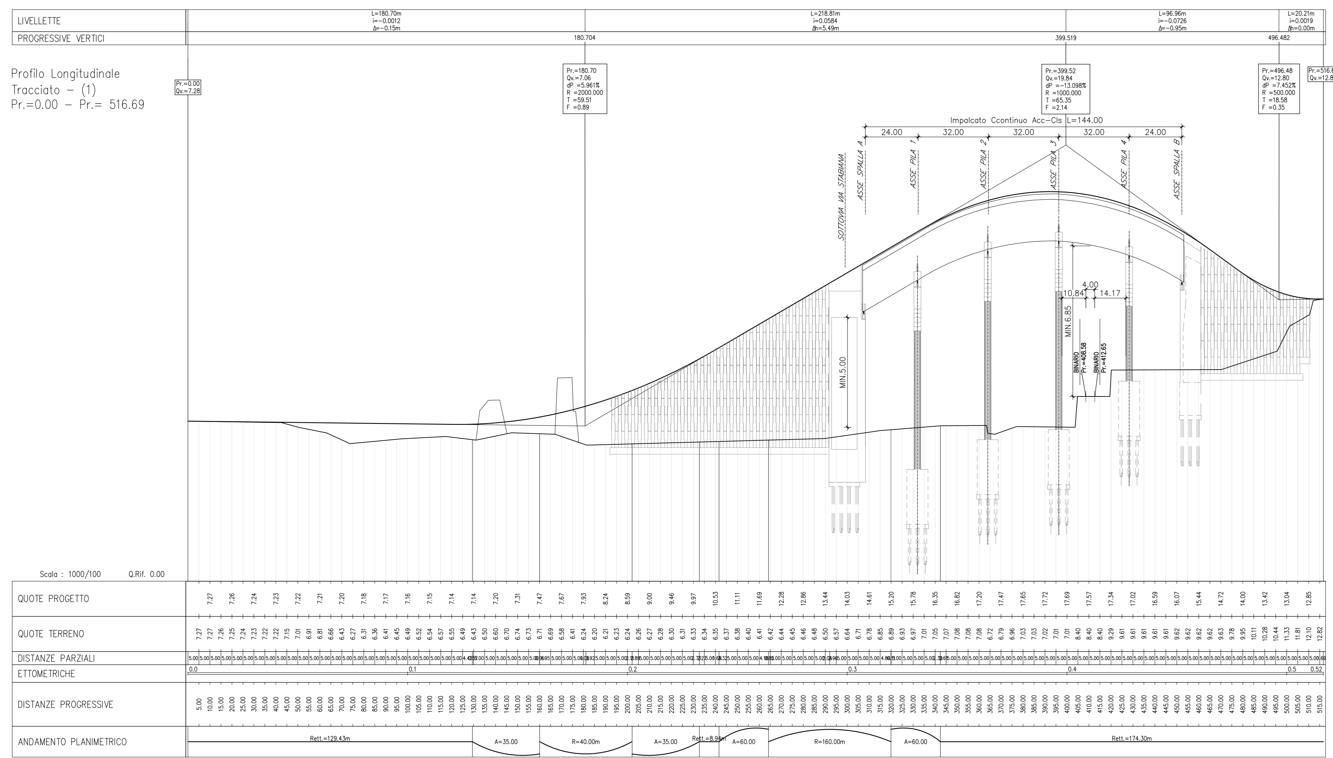
PROFILO DI PROGETTO Scala 1:1000
