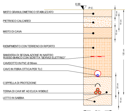
Figura 4: Sezione di scavo per la posa del cavidotto su strada esistente
