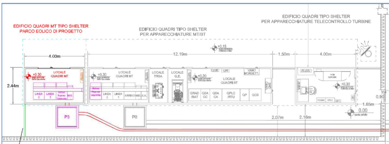
Figura 5: Layout in SSE Produttore in corso di autorizzazione
