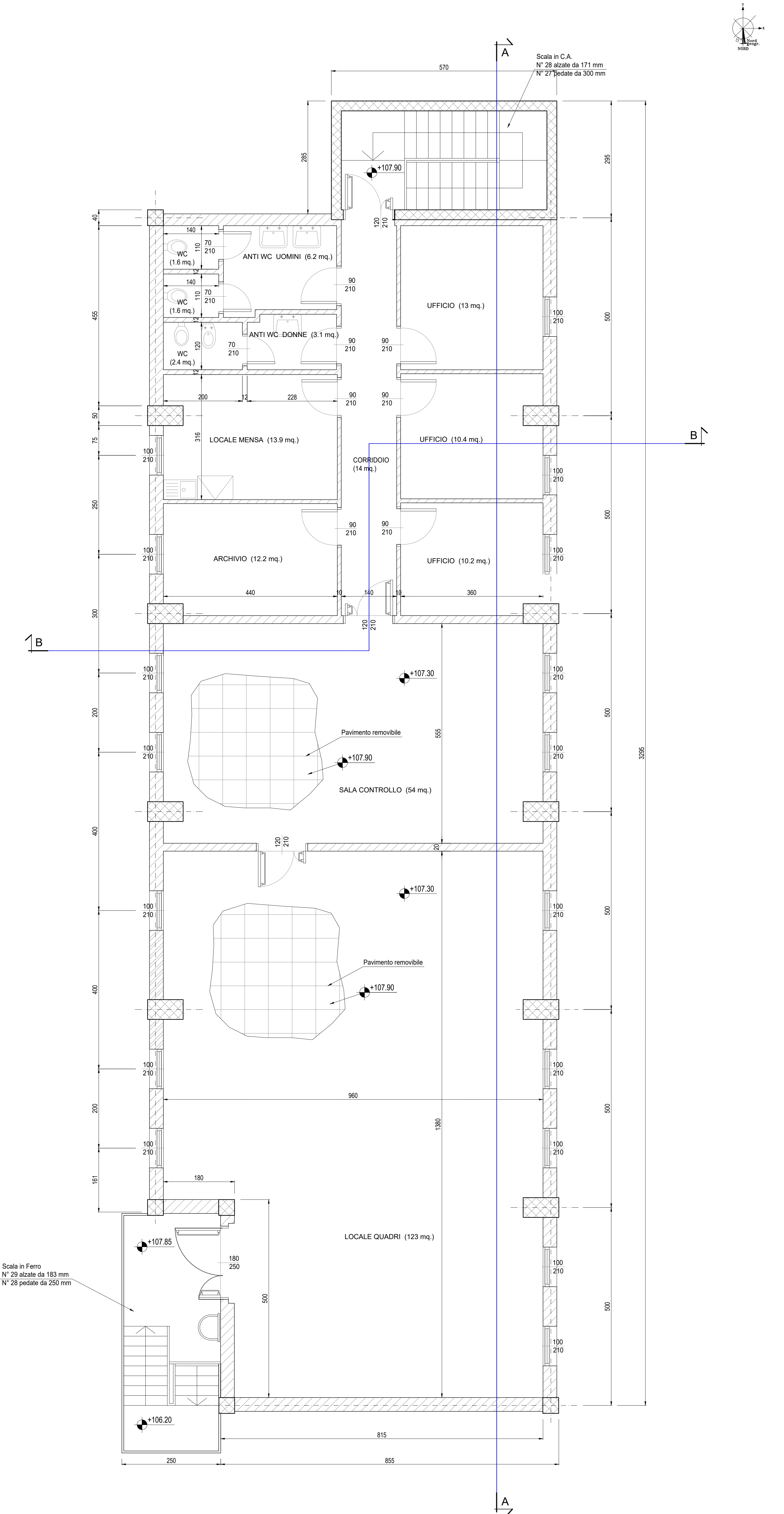
PIANTA LIVELLO +7.90 Scala: 1:50
