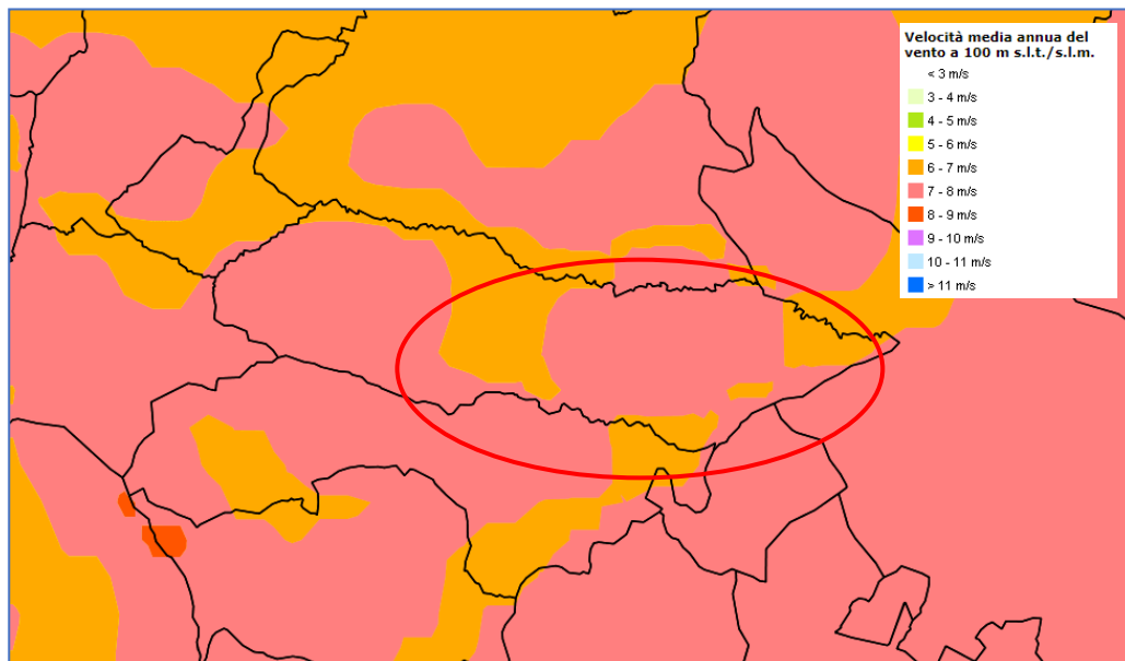
Figura 11 - Velocità media annua del vento a 100 m s.l.m.m - fonte Atlante Eolico
