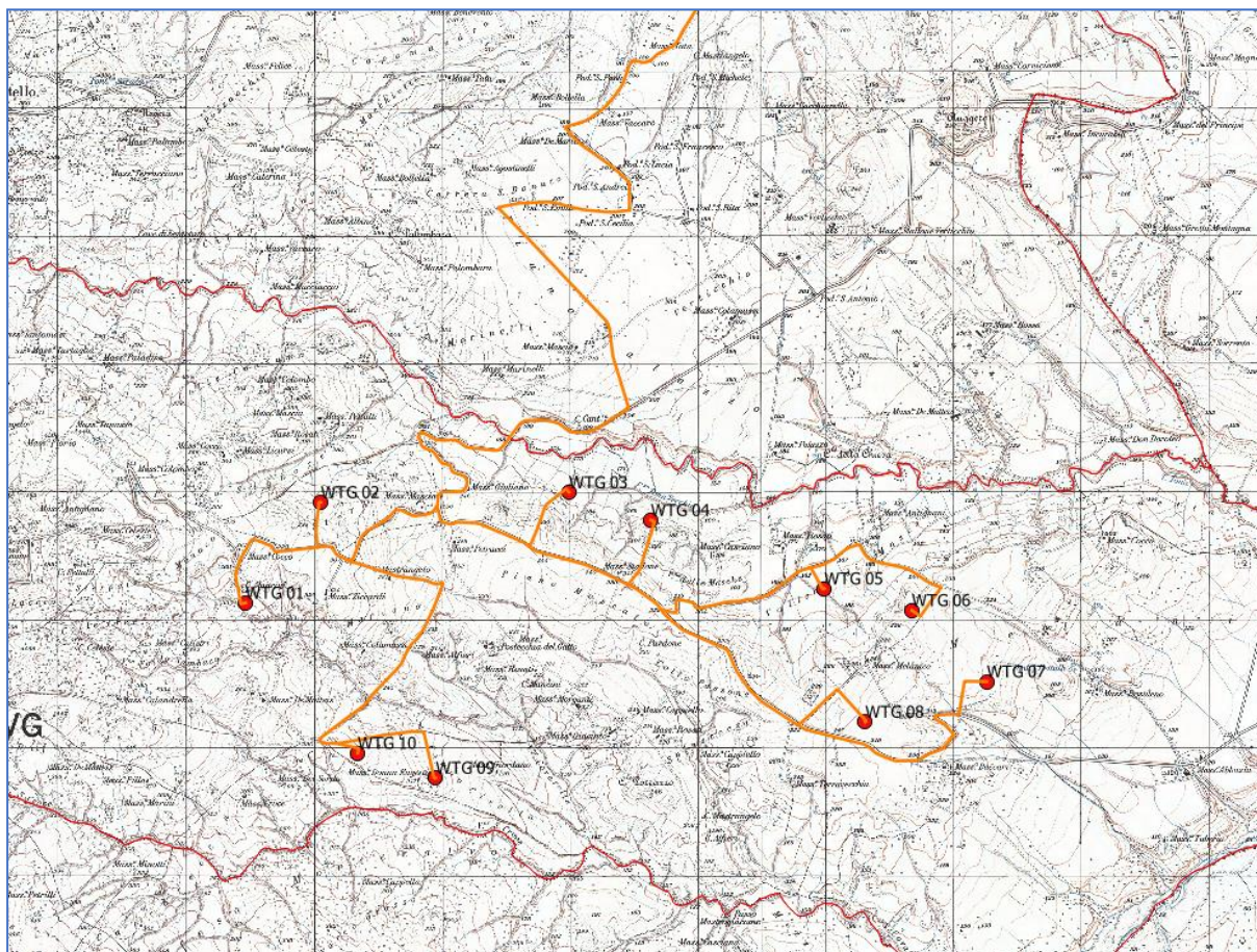
Figura 7 - layout impianto definitivo a n.10 aerogeneratori
