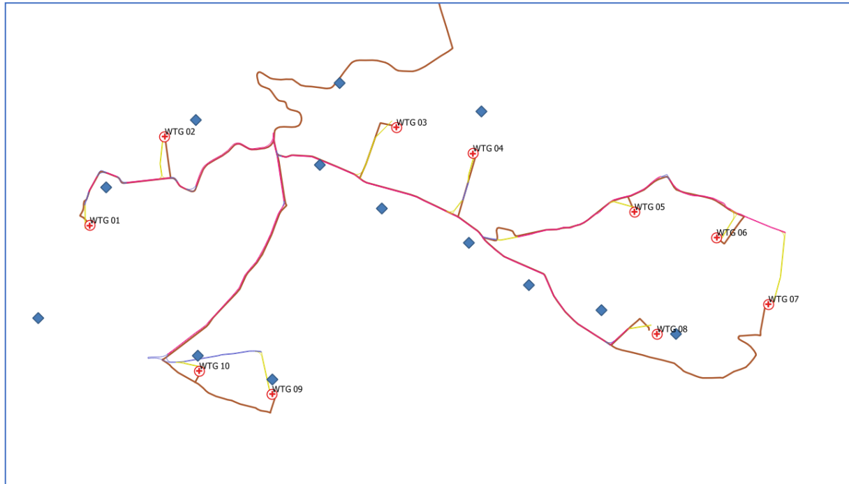
Figura 6 - Sovrapposizione schema layout di partenza a 13 WTG (in blu) e schema definitivo a 10 WTG (in rosso).
