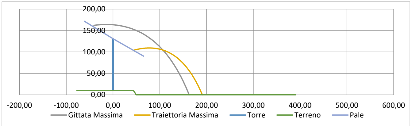
Figura 4 - Traiettoria del moto della pala intera, a seguito del distacco
