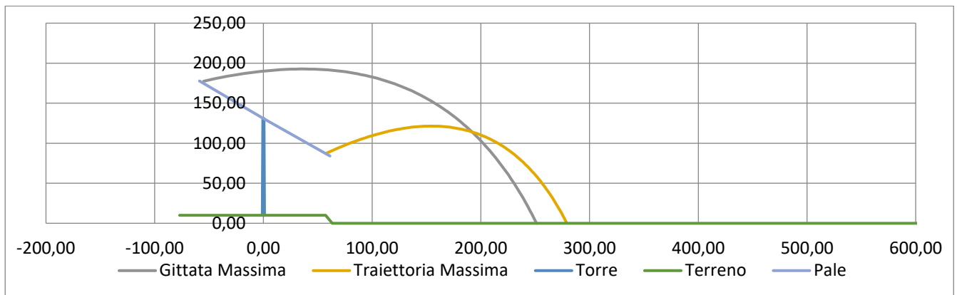
Figura 5 - Traiettoria del moto di un frammento di 10 m, a seguito di rottura
