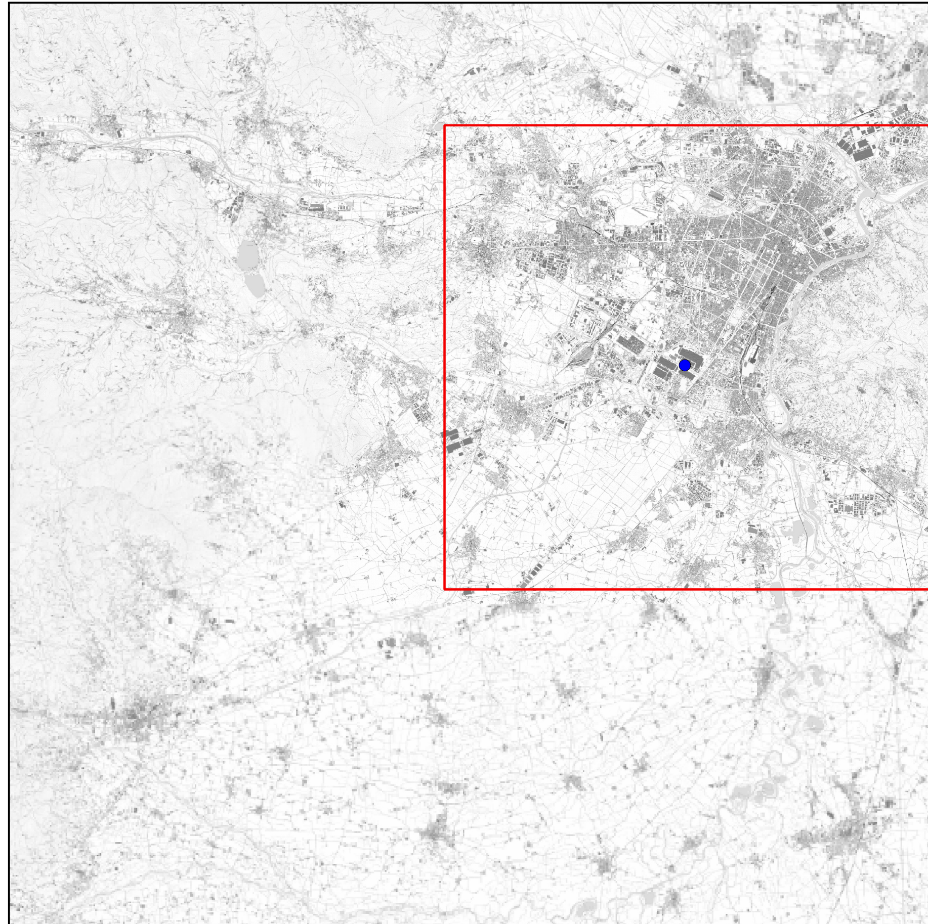
Figura 4.4.2 a Dominio di calcolo di CALMET e dominio di calcolo CALPUFF
