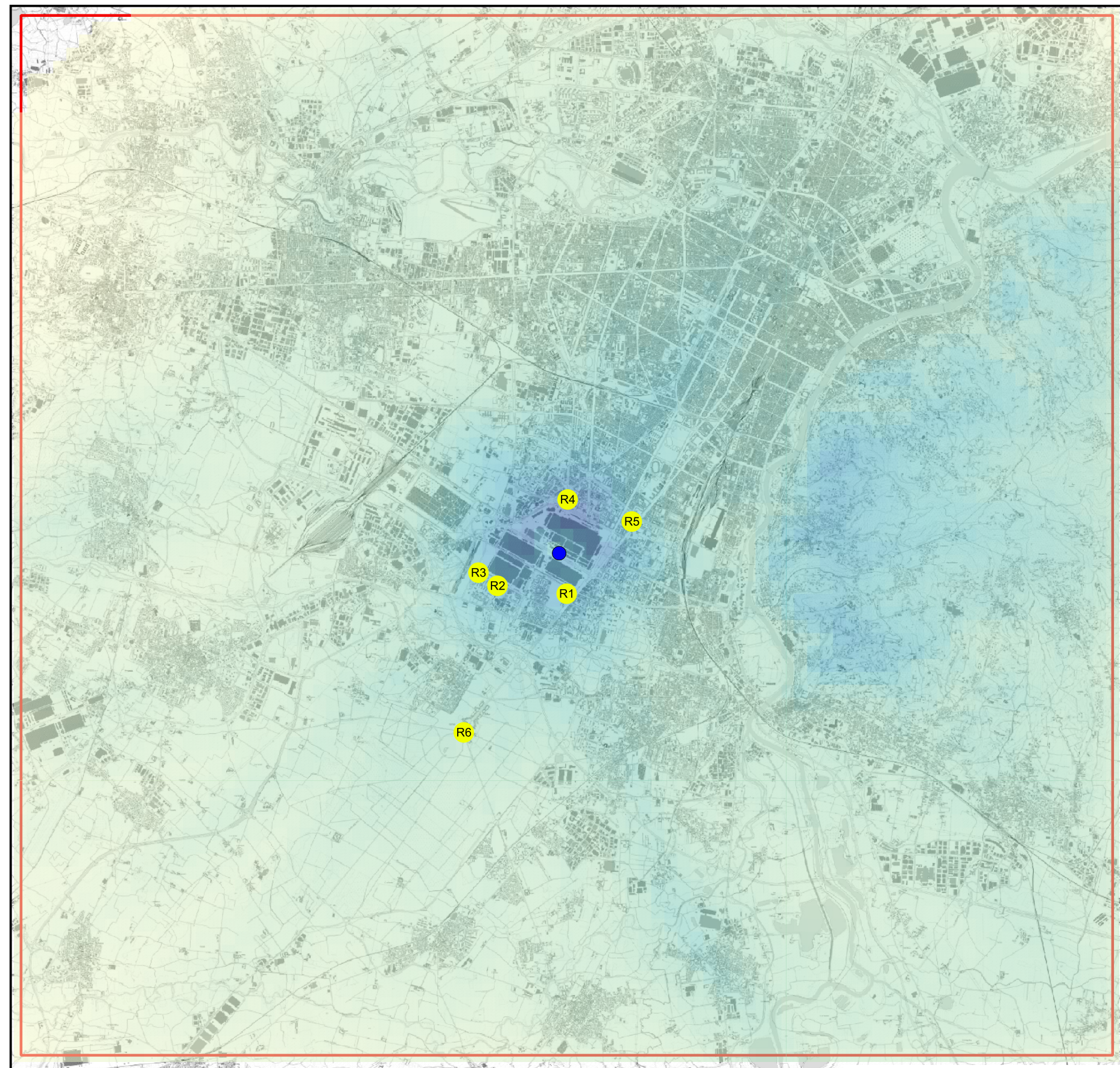
Figura 4.7.2a 99,8° percentile delle concentrazioni medie orarie di NOx scenario FUTURO
