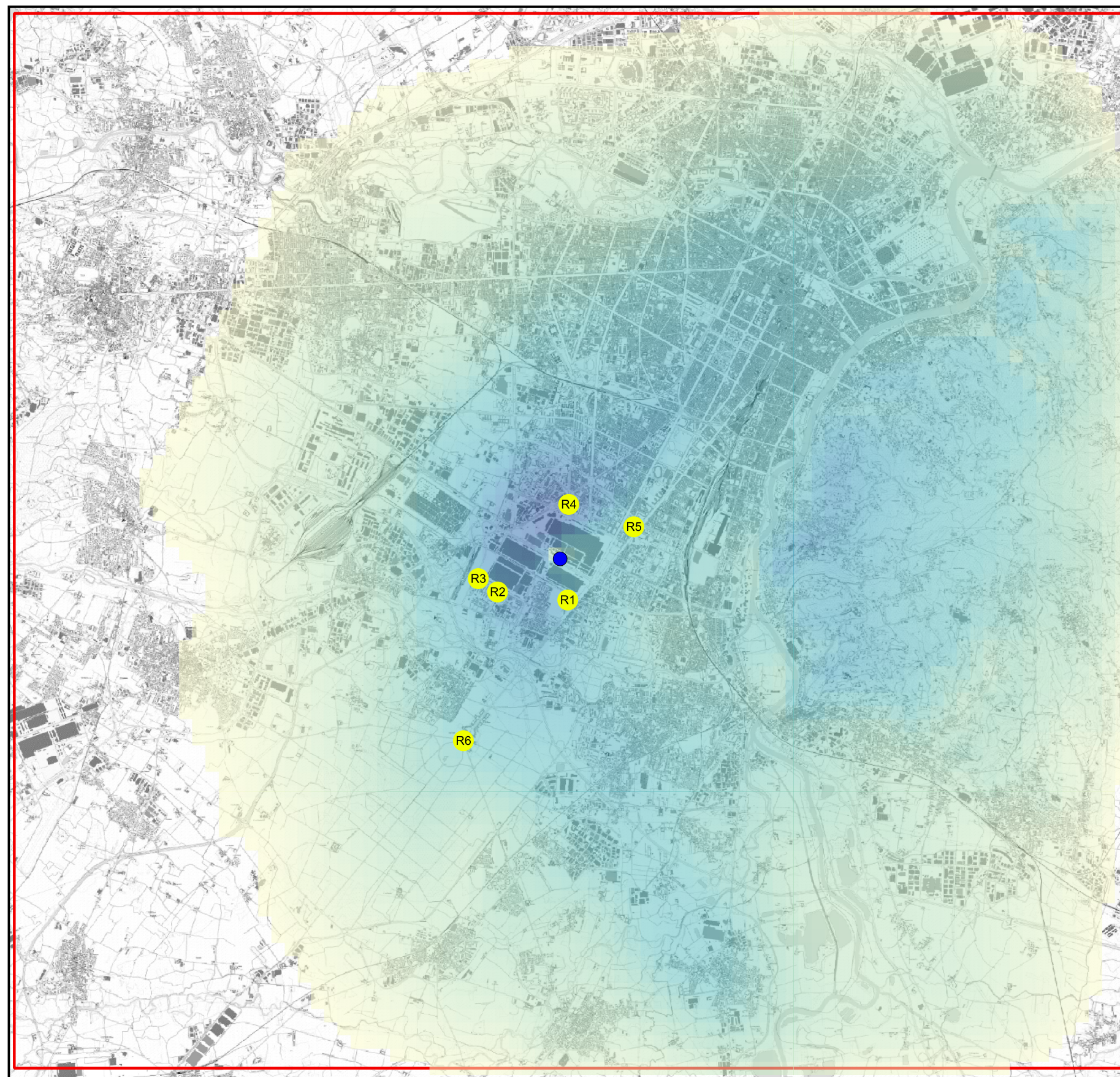
Figura 4.7.2b Concentrazione media annua di NOx scenario FUTURO
