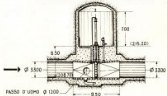
CAMERA DI MANOVRA DELLA PARATOIA DI SEZIONAMENTO DELLA DERIVAZIONE DEL SANGRO SEZIONE A - A
