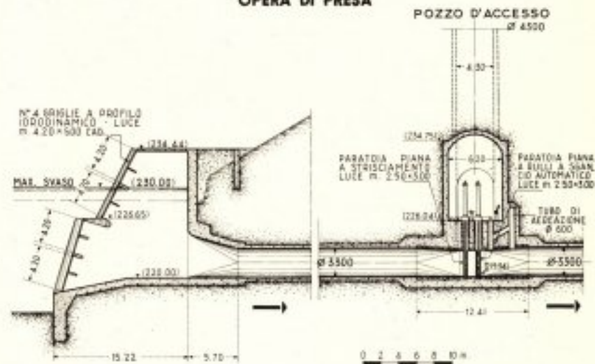
OPERA DI PRESA
