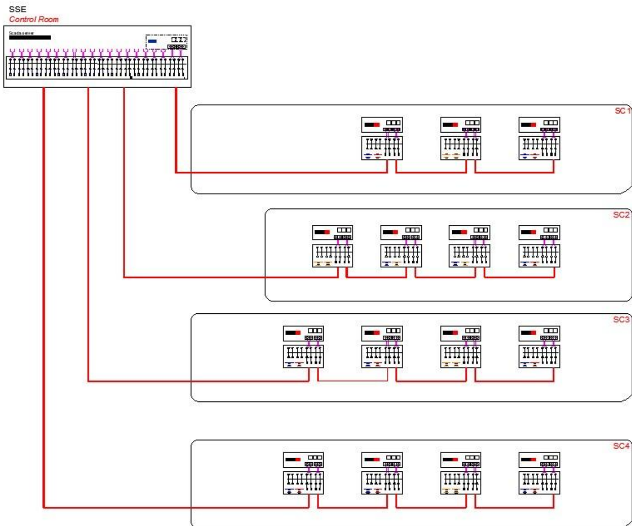
Figura 1 - Schema Fibra ottica
