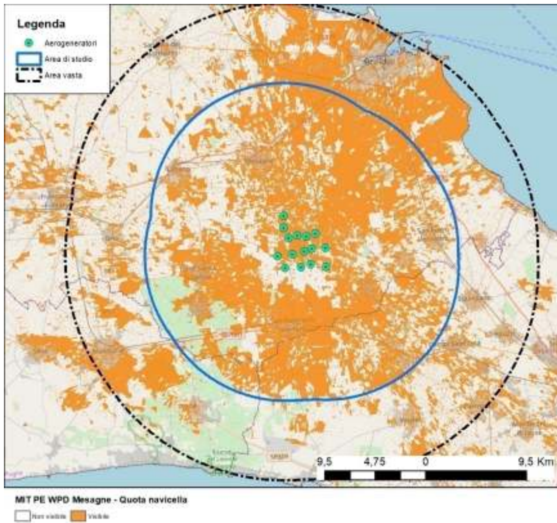
Figura 5 - MIT altezza navicella relativa allo stato di progetto – Classi di visibilità
