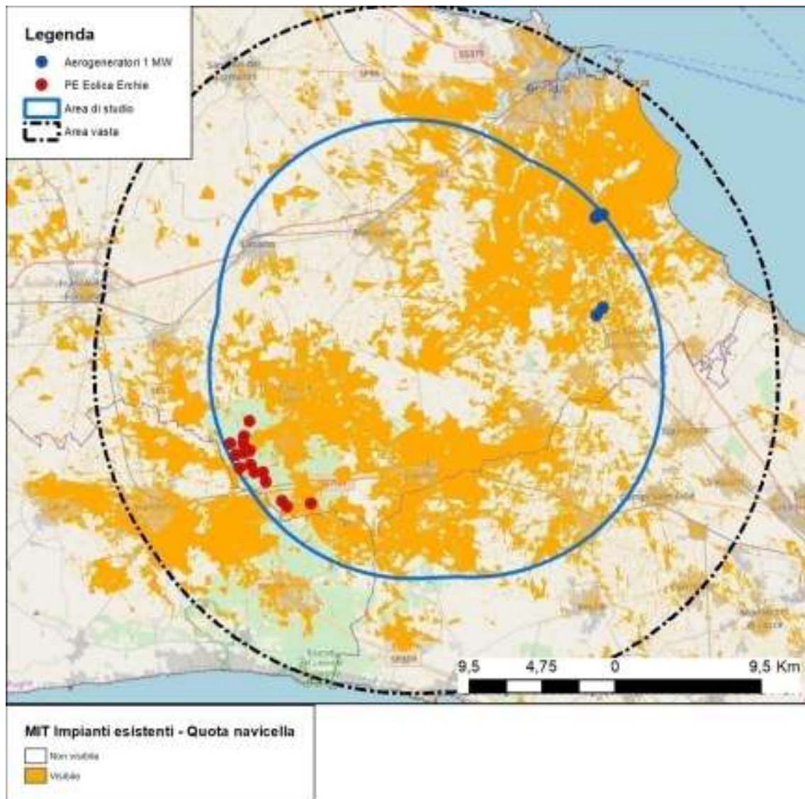
Figura 3 - MIT altezza navicella relativa allo stato di fatto (solo impianto Eolica Erchie ed aerogeneratori singoli nei comuni di Brindisi e San Pietro Vernotico)
