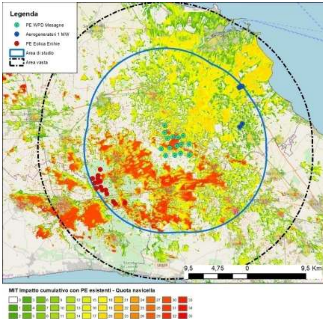
Figura 6 - MIT altezza navicella relativa allo stato di progetto – Classi di visibilità (Ipotesi di non realizzazione del PE Gamesa)
