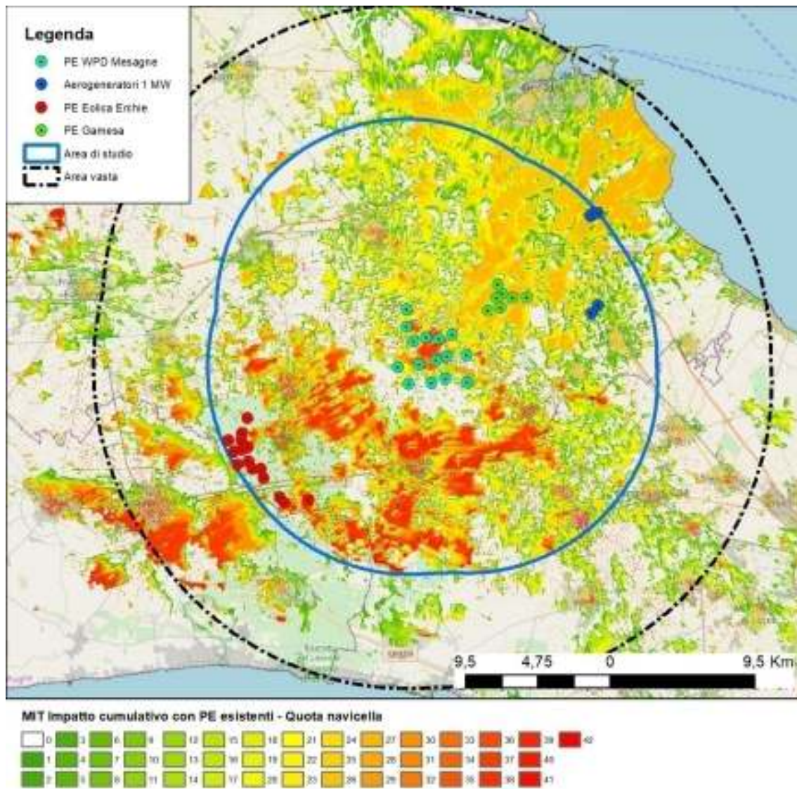
Figura 7 - MIT altezza navicella relativa allo stato di progetto complessivo- Classi di visibilità (Ipotesi di realizzazione del PE Gamesa)
