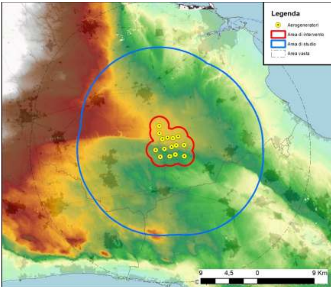
Figura 2 - Area di Impatto Potenziale
