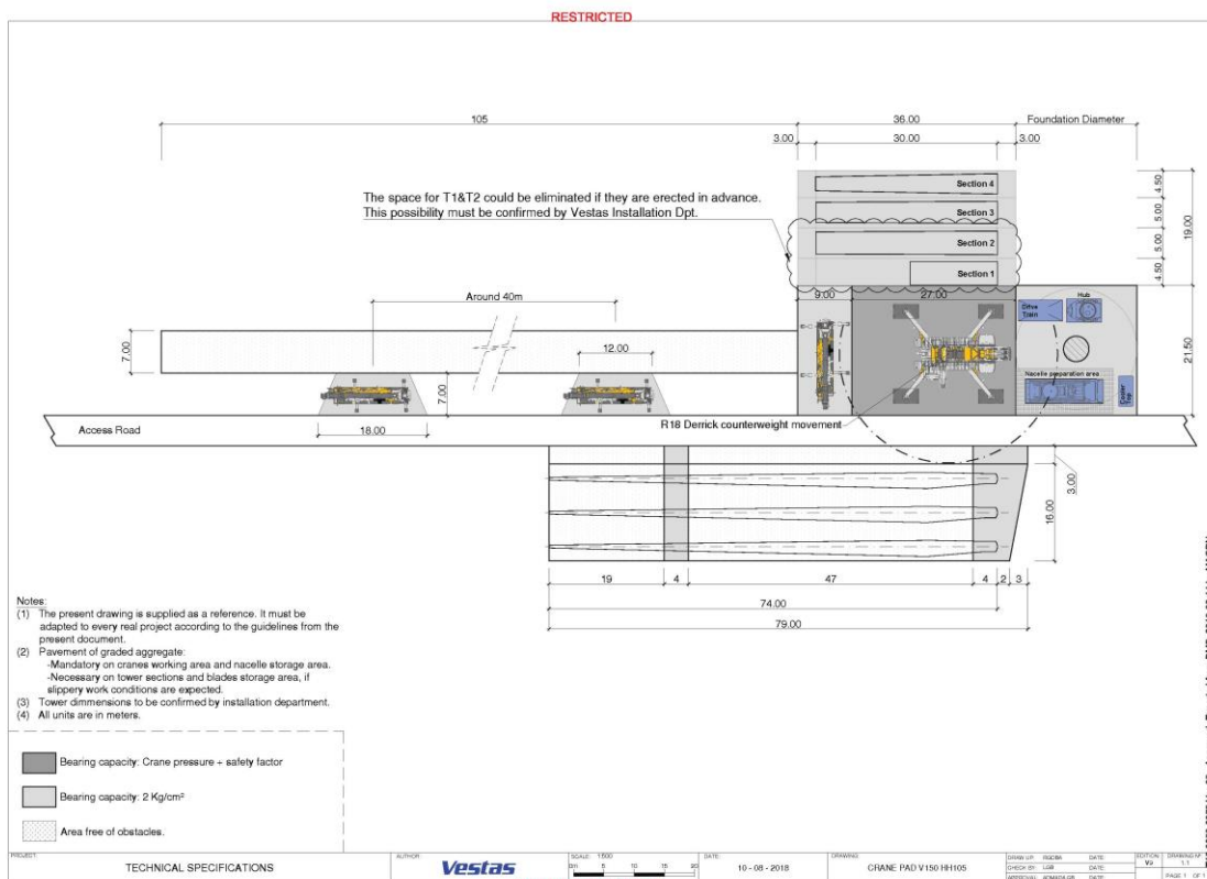
Figura 5. Piazzola aerogeneratore
