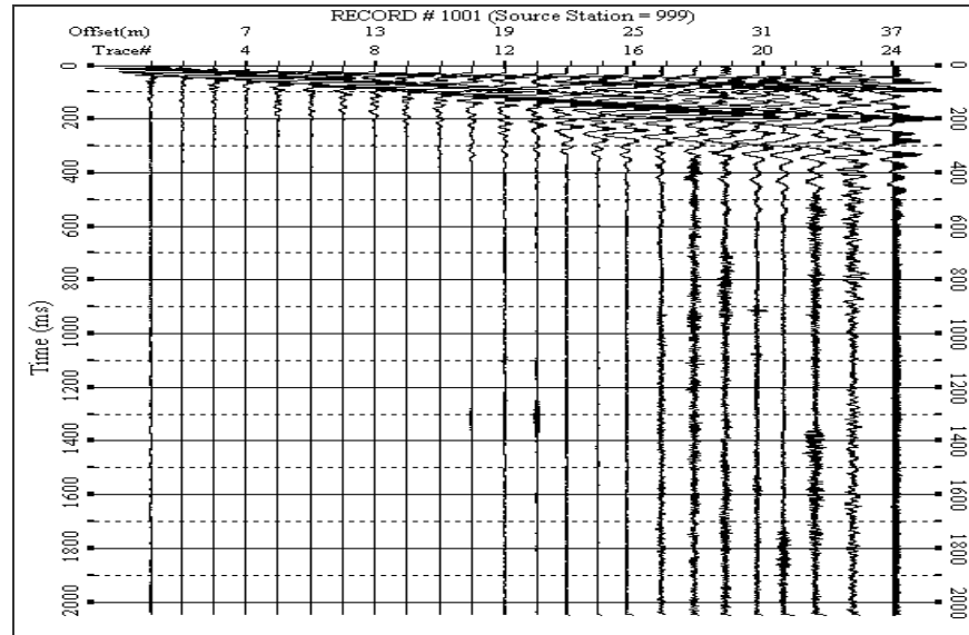
Risultati stendimento MASW
