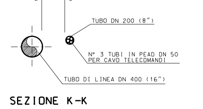
SEZIONE K-K
