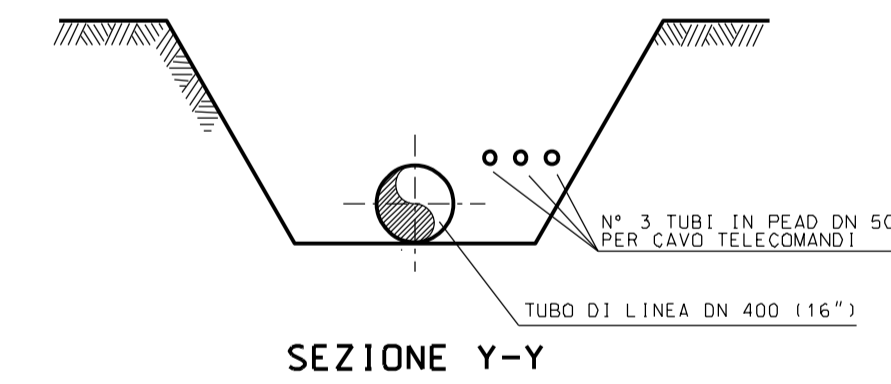
SEZIONE Y-Y
