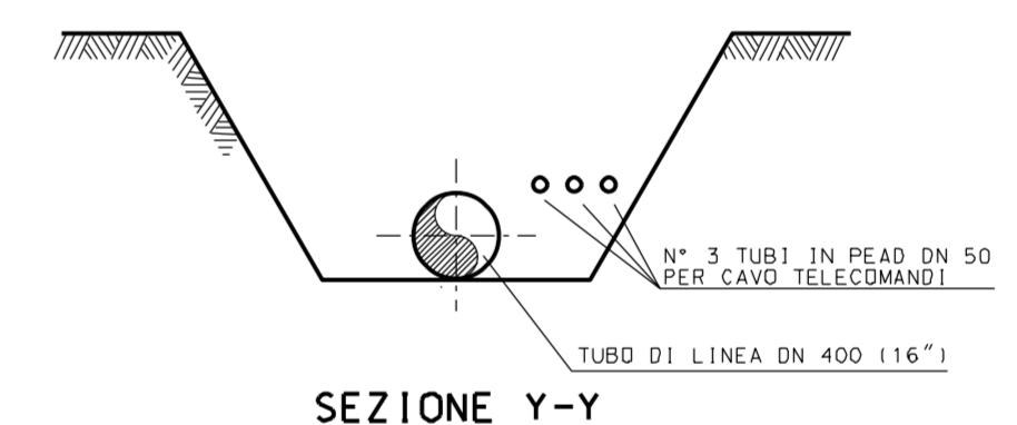
SEZIONE Y-Y
