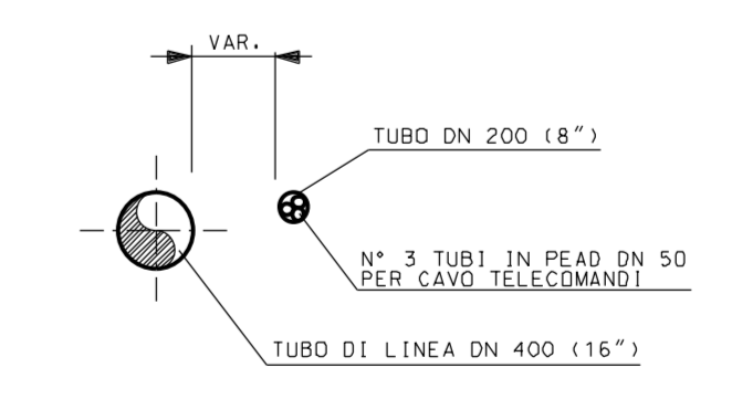
SEZIONE K-K
