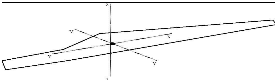
Fig 2 – Sistema di coordinate usato per la pala YY (Flapwise); XX (Pitchwise); ZZ (Edgewise)
