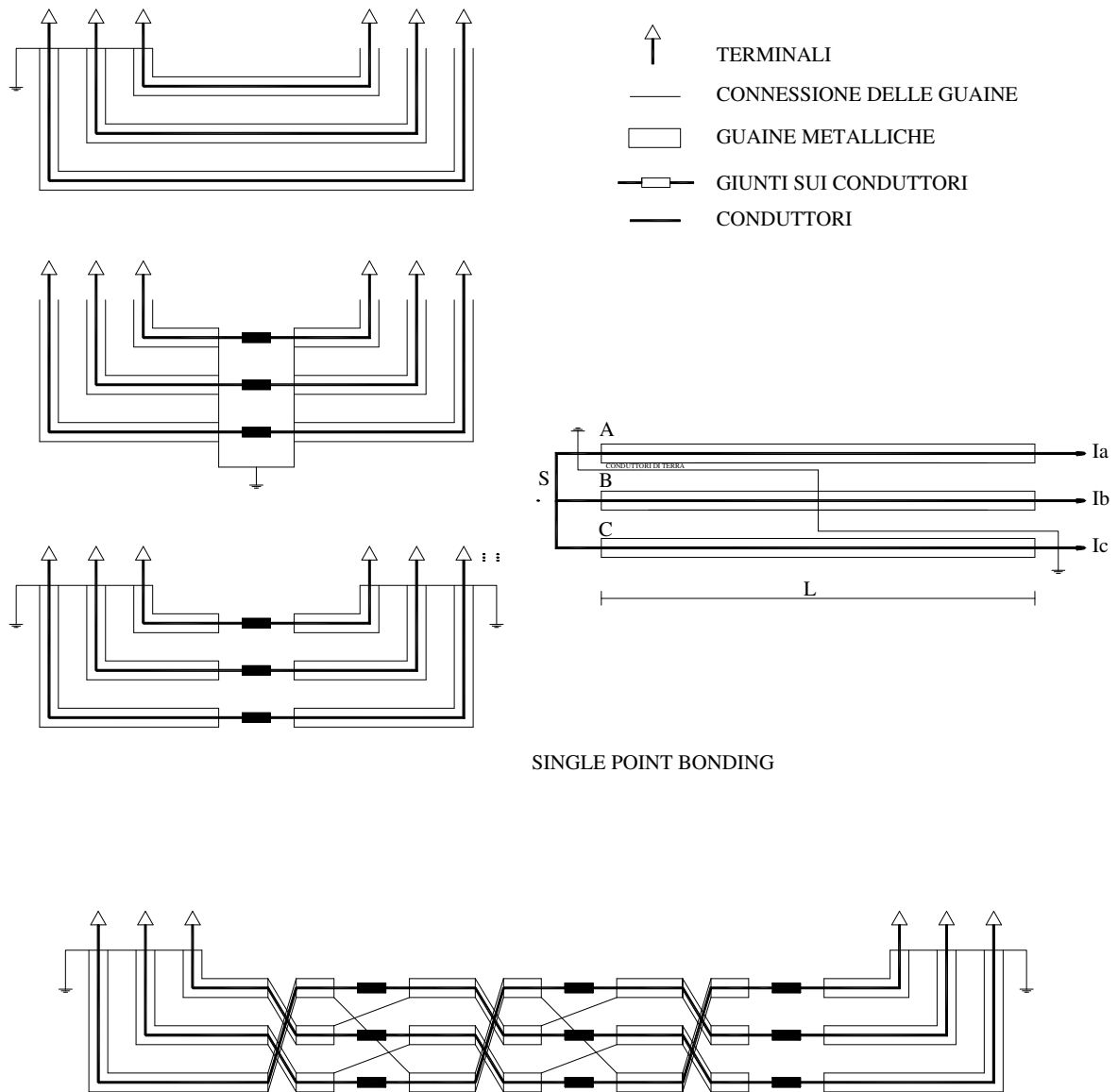
Fig.18.2: Schema di connessione delle guaine metalliche
