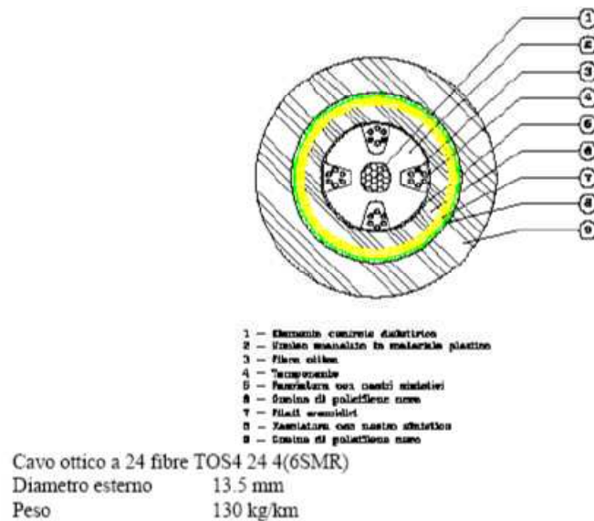
Fig.13.1: Schema cavo fibre ottiche
