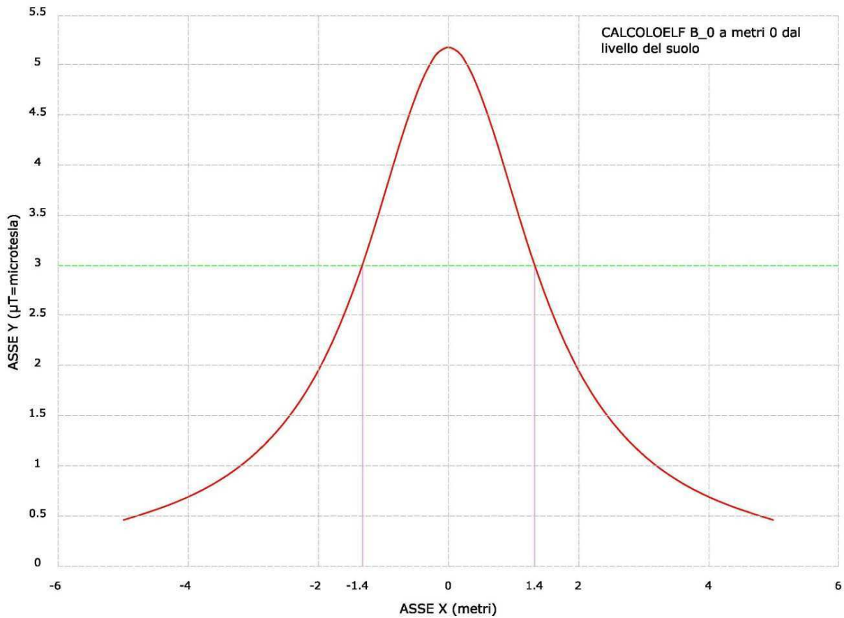
Fig.16.1: andamento dell'induzione magnetica prodotta dalla linea in cavo
