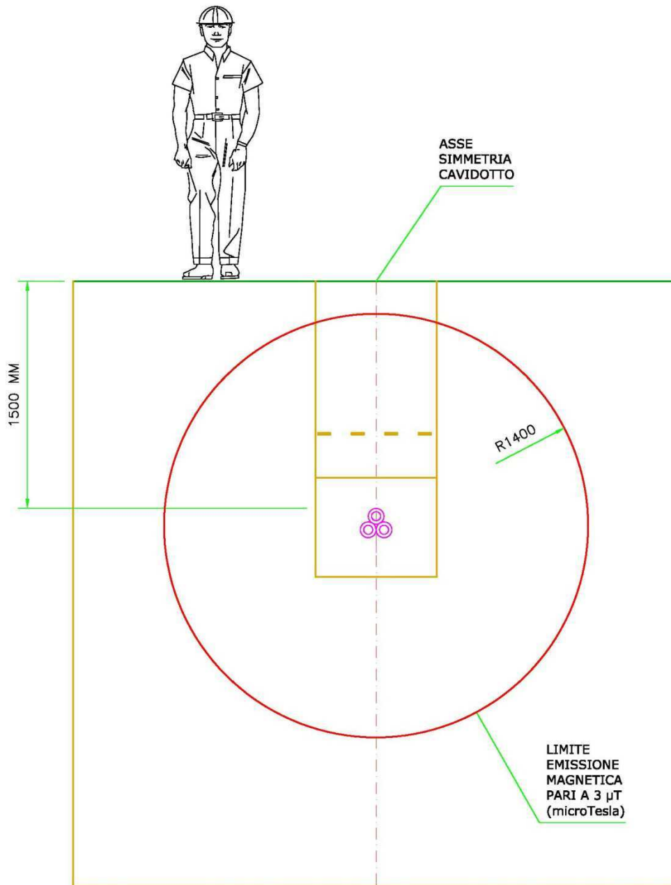
Fig.16.2: sezione tipica cavidotto
