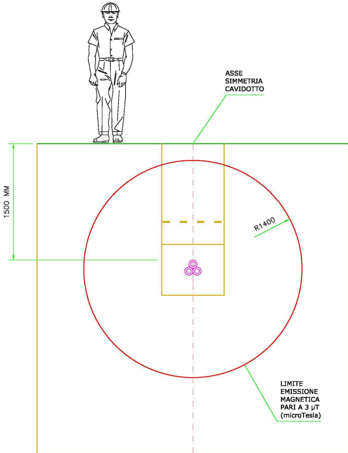
Fig.18.1: Sezione di posa
