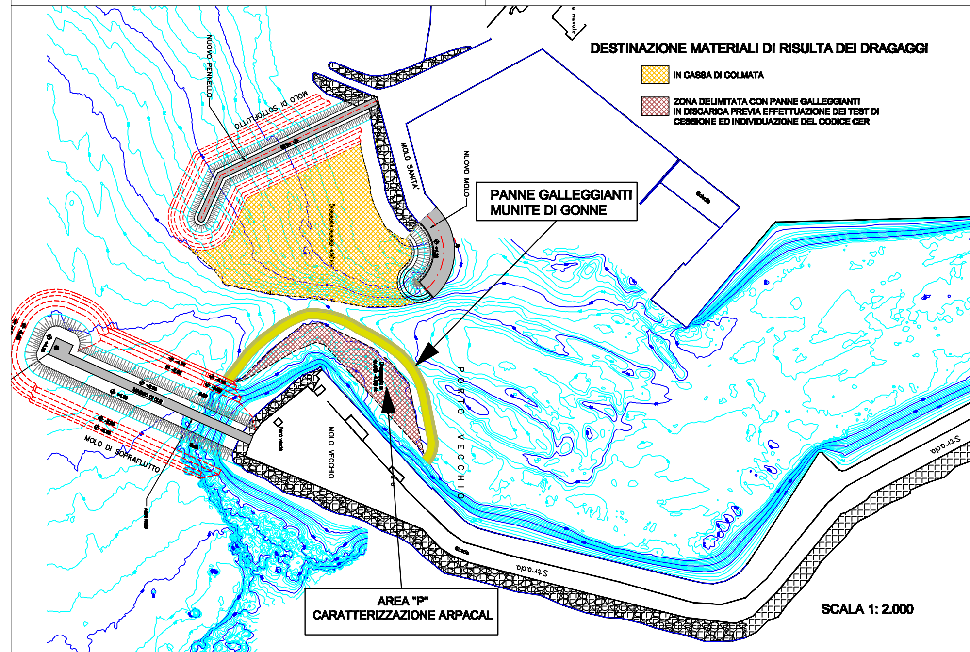
Schermo di protezione rappresentazione della fase di separazione e confinamento dell'area interessata dal dragaggio con panne, dotate di gonne.
